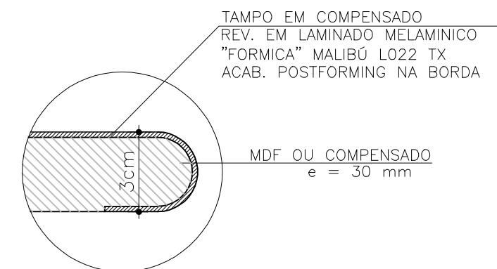
DET. BORDA DO TAMPO
