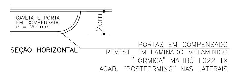
DET. LATERAL PORTAS
