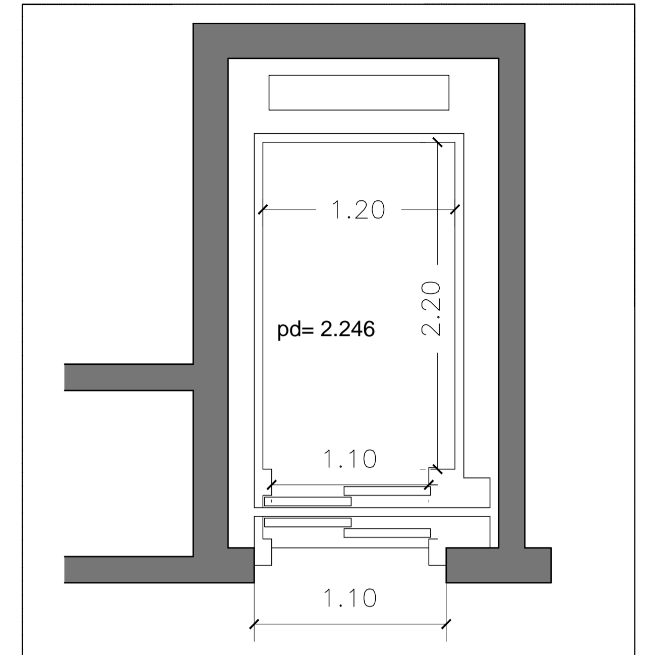
Proposta: Térreo ao 1º pavto
