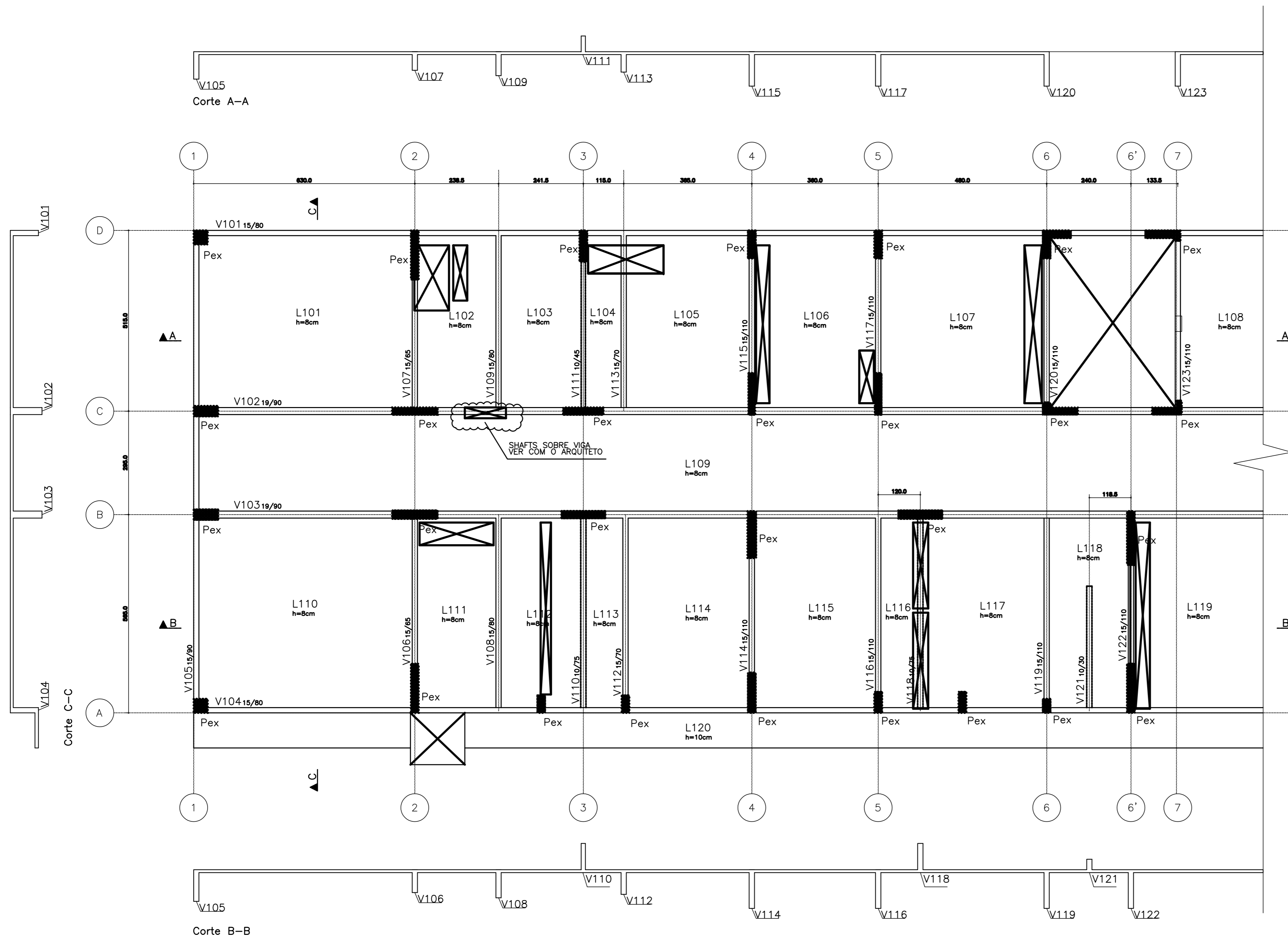
CADASTRAMENTO ESTRUTURAL 1º PAVIMENTO
