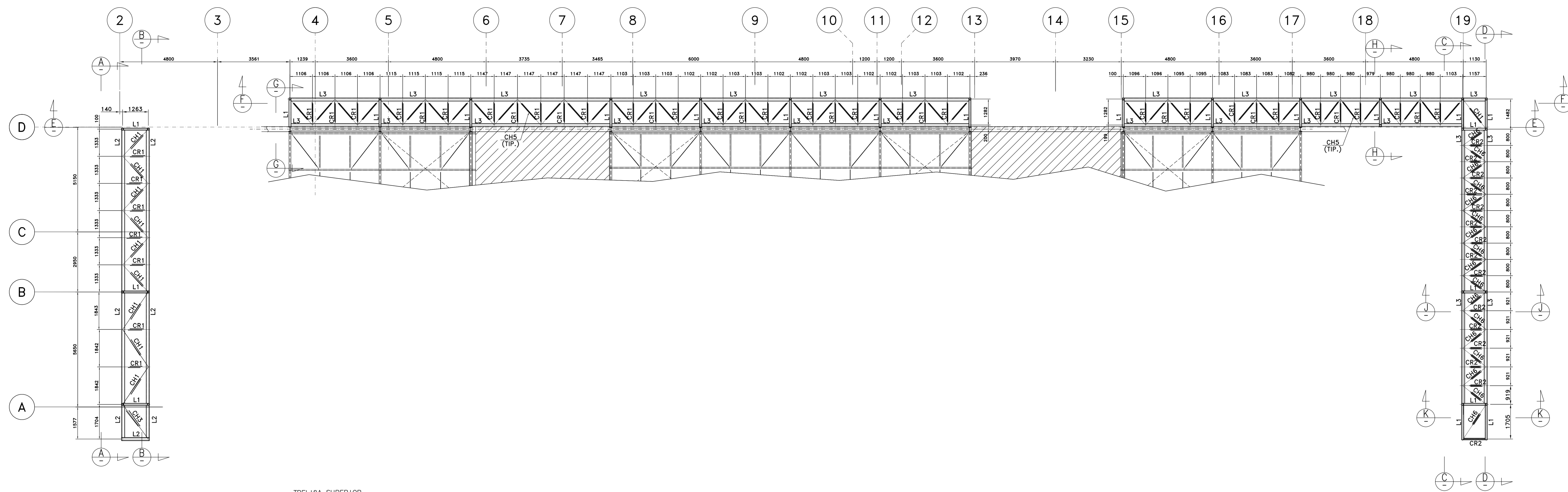
TRELIÇA SUPERIOR ESC. 1:100
