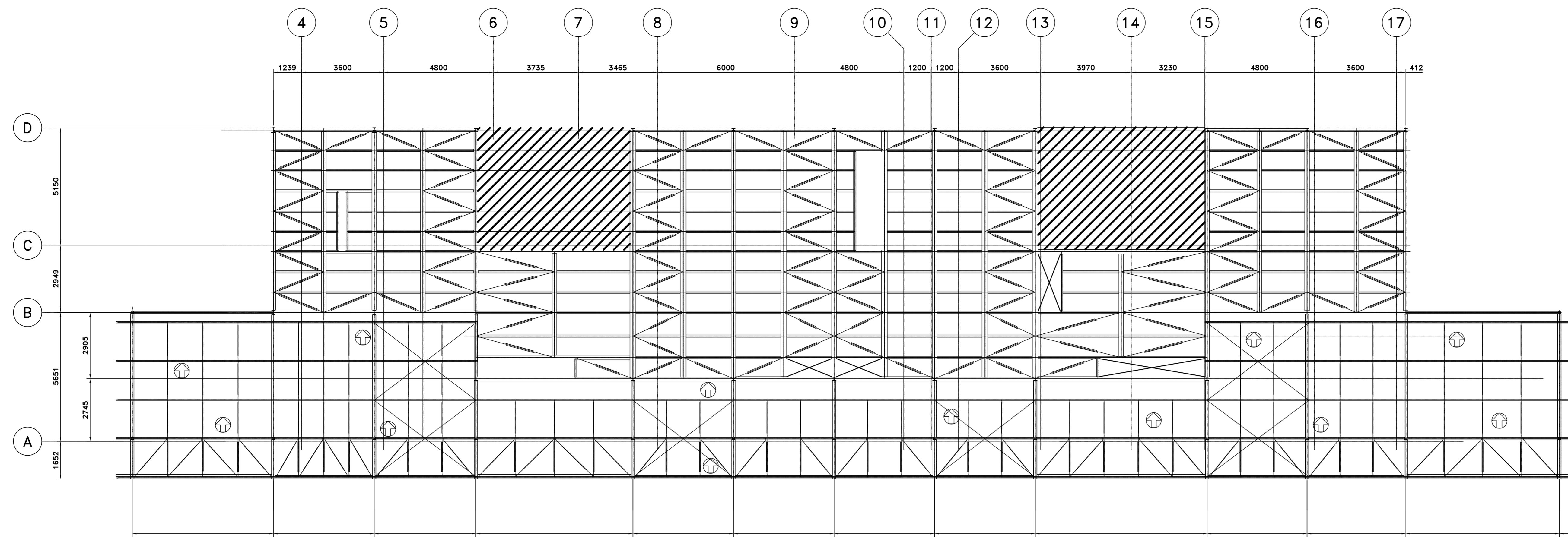
PLANTA DE PISOS ESC. 1:100 (EL. 857,87)
