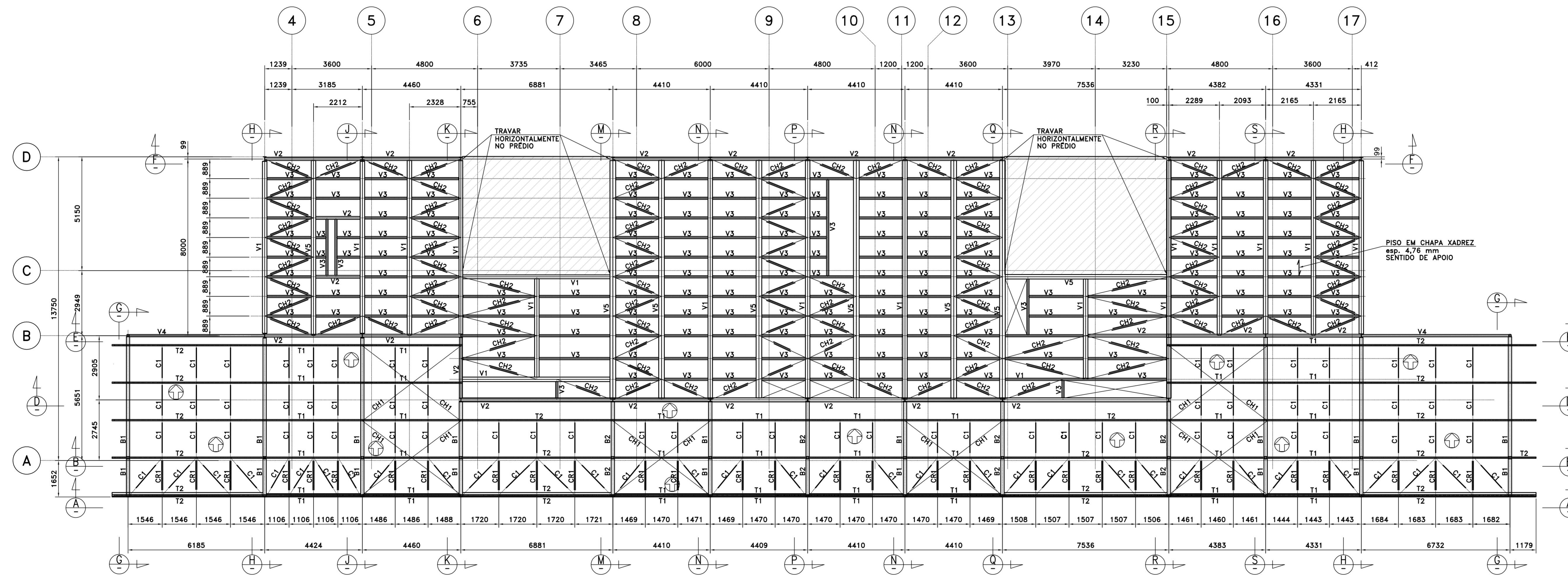
PLANTA DA PLATAFORMA ESC. 1:100 (EL. 853,11)
