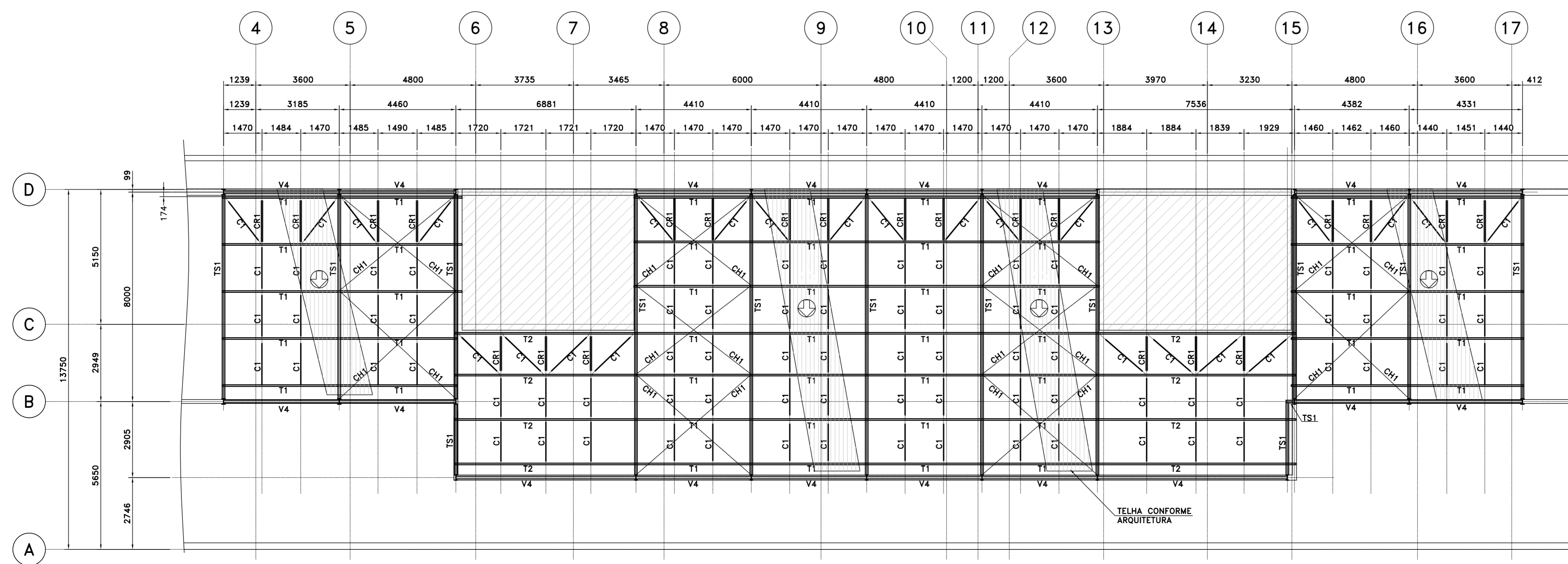
PLANTA DA COBERTURA ESC. 1:100
