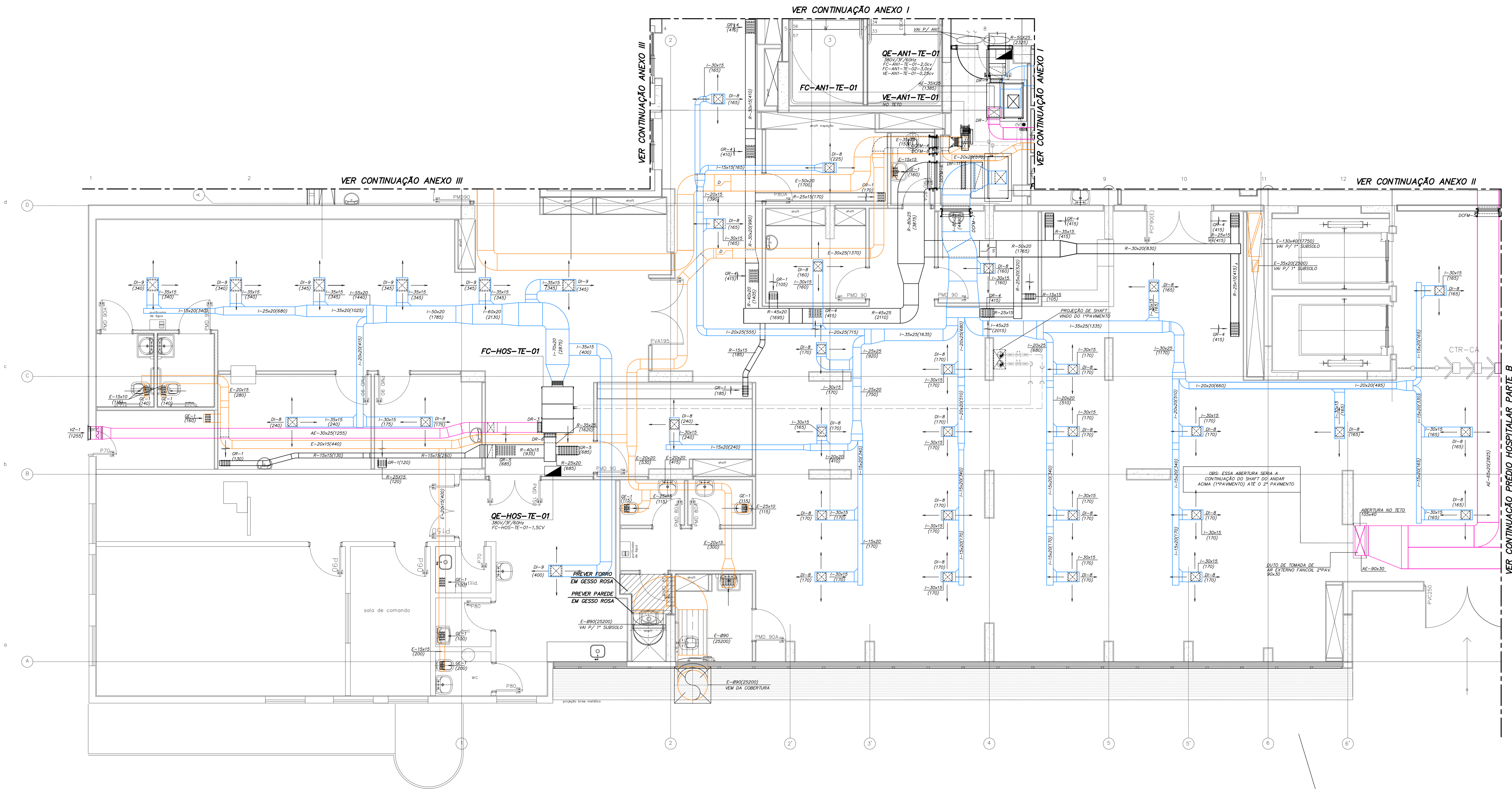
PLANTA PARCIAL DO TERREO-PREDIO HOSPITALAR
