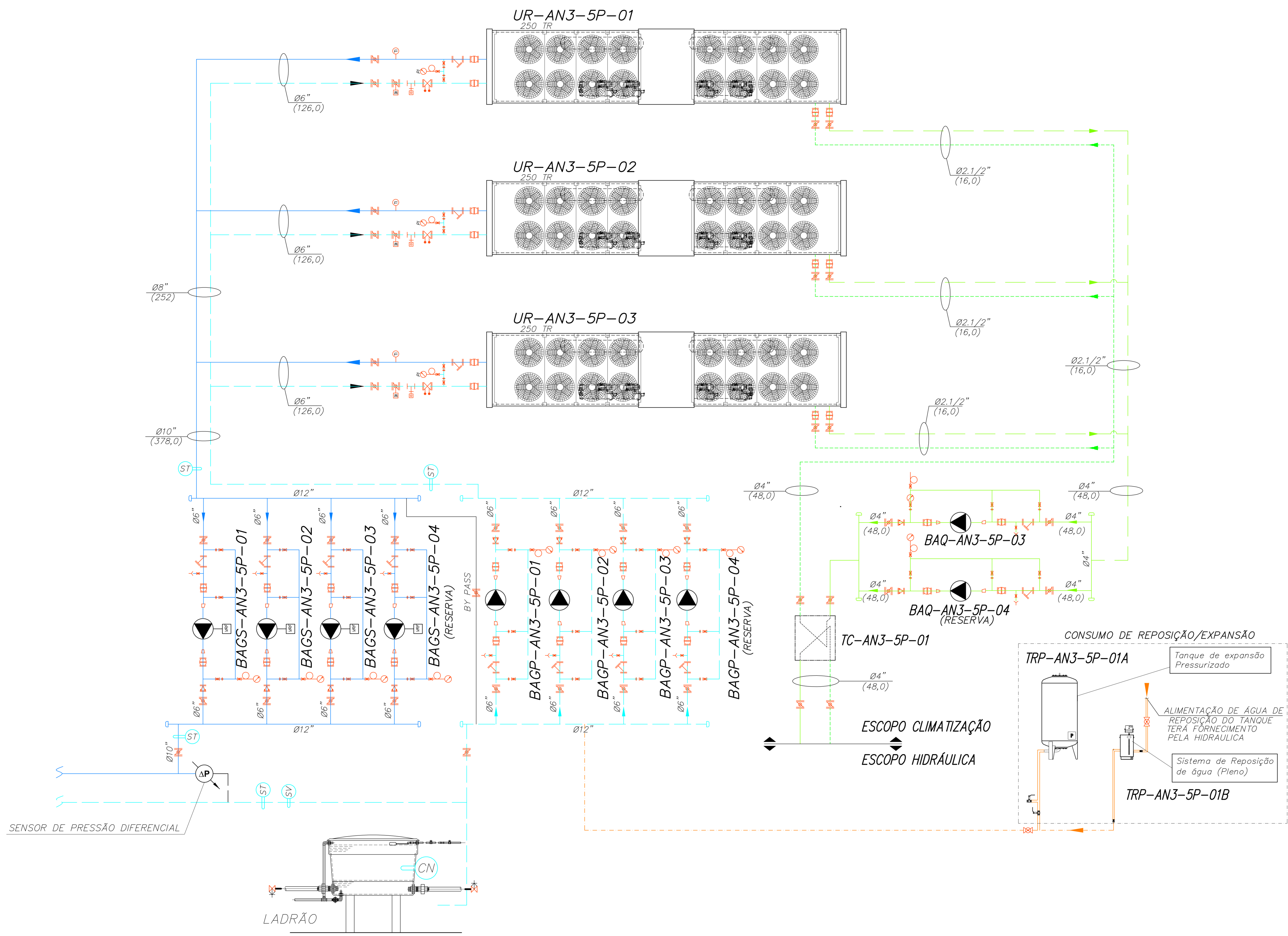
FLUXOGRAMA HIDRÁULICO DA CAG
