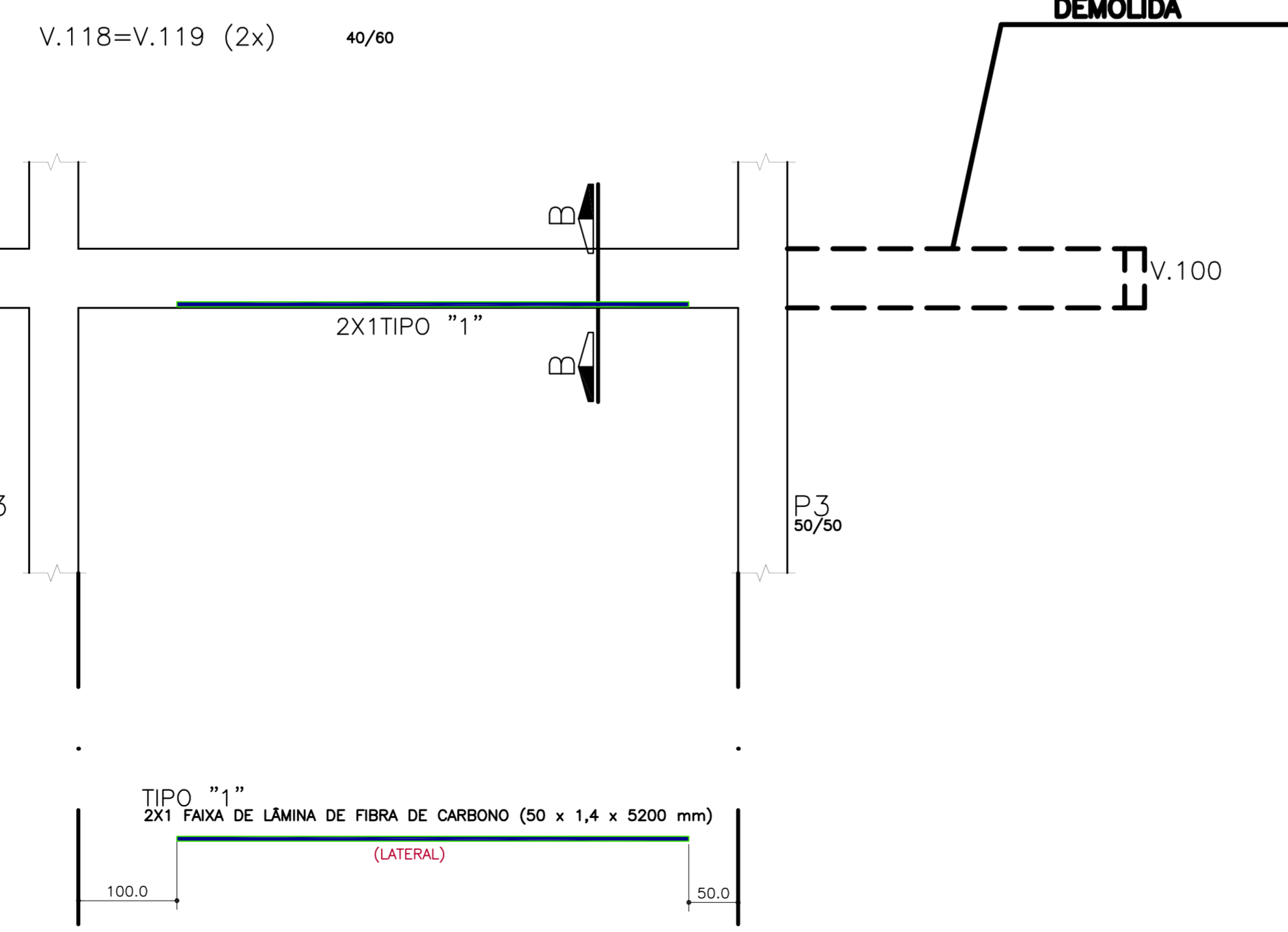
CORTE A-A ESCALA= 1:5
