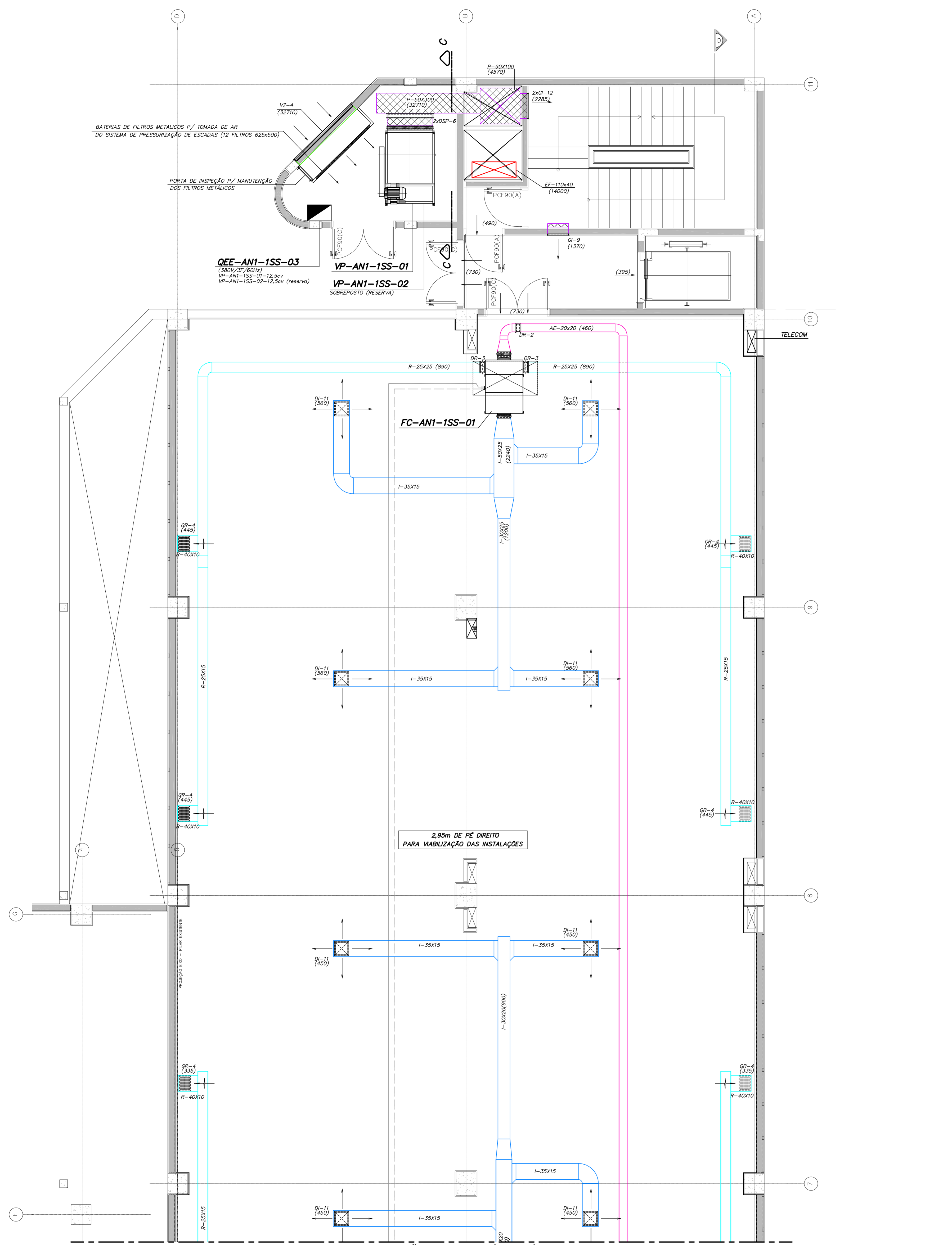
PLANTA 1º SUBSOLO-ANEXO 1
