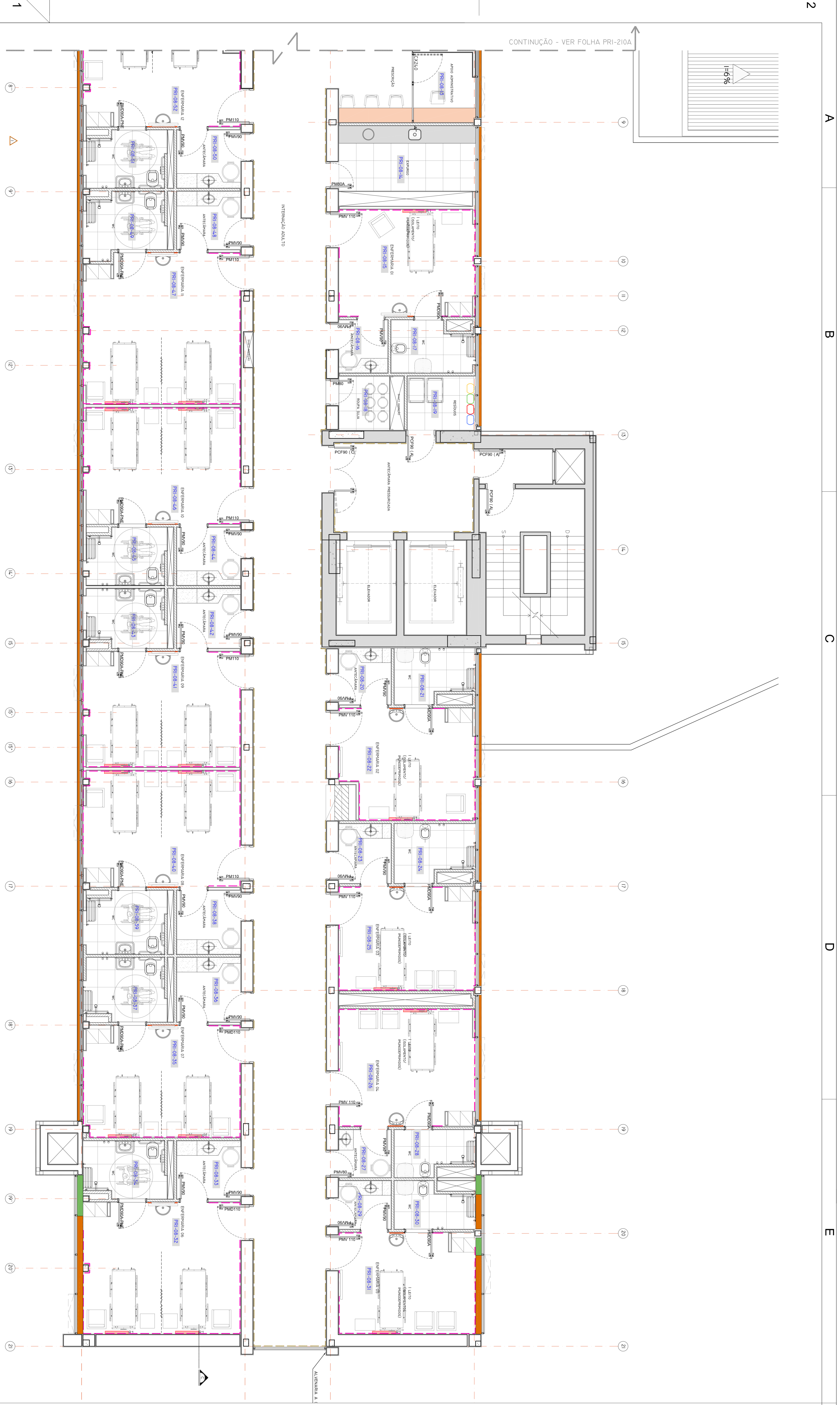
PLANTA DE LAYOUT - 8º PAVIMENTO
