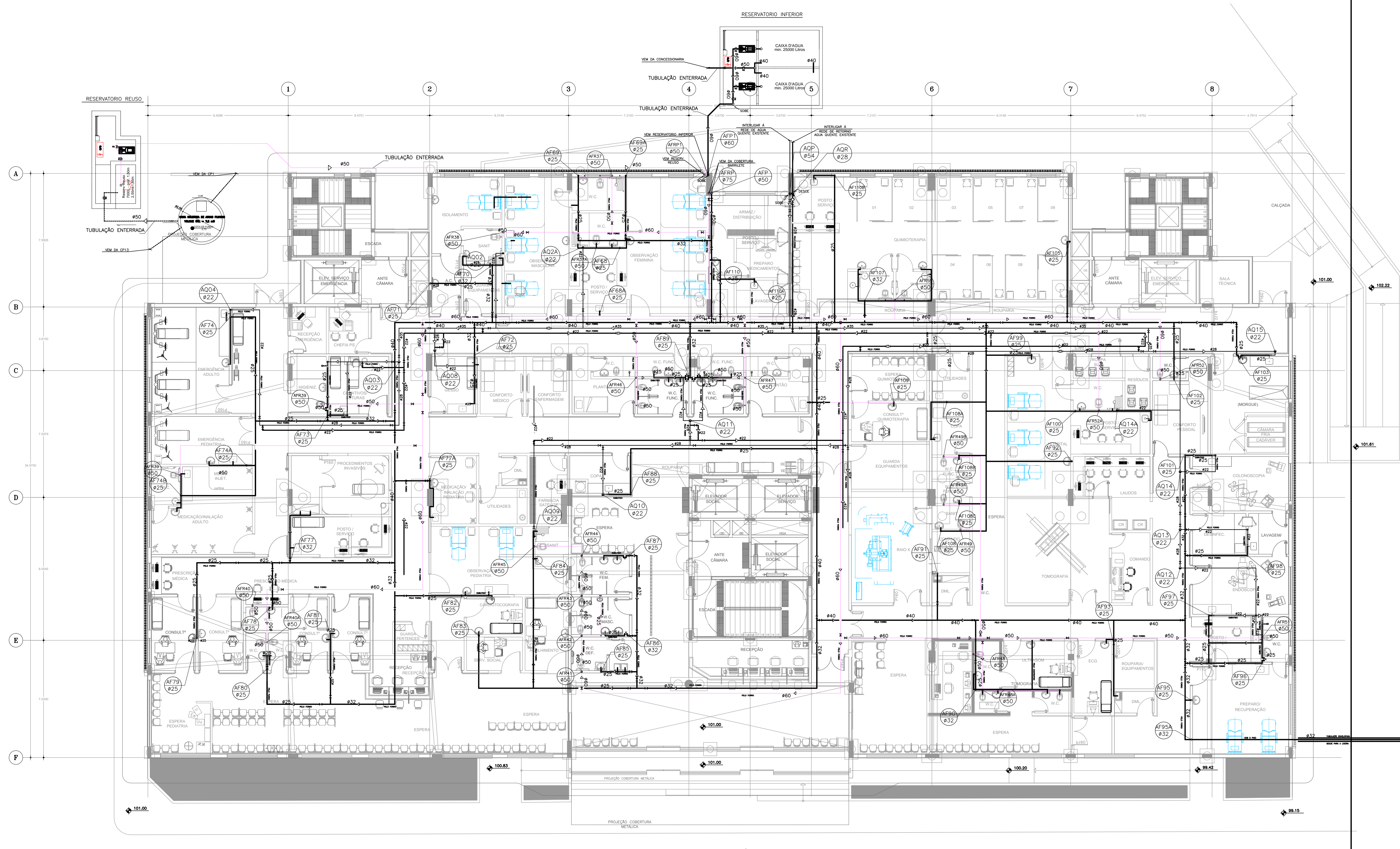
PLANTA REDE DE AGUA FRIA E QUENTE E REUSO
