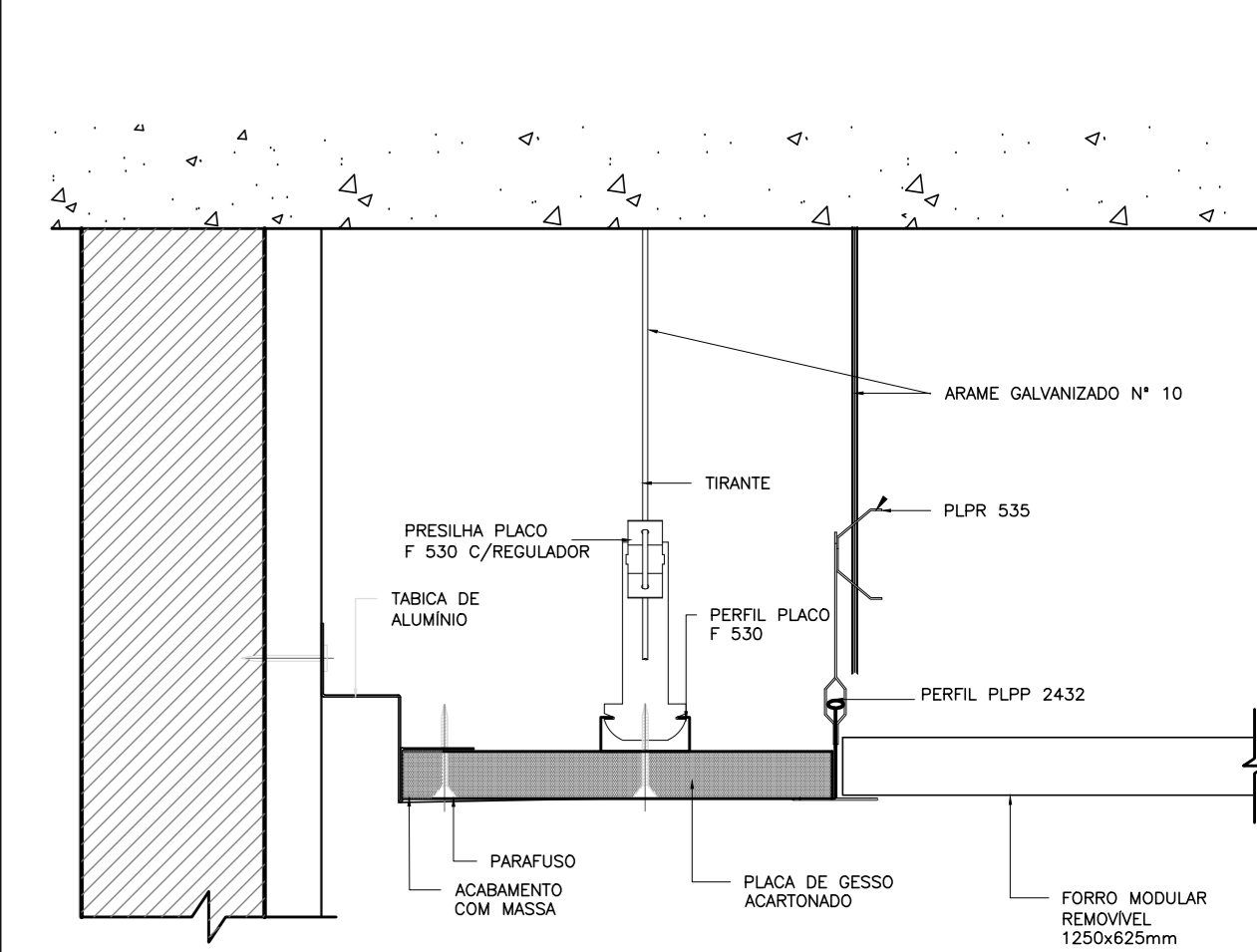
DETALHE ARREIMATE FORRO DE GESSO / FORRO REMOVÍVEL ESQ: 1/2 MEDIDAS CM
