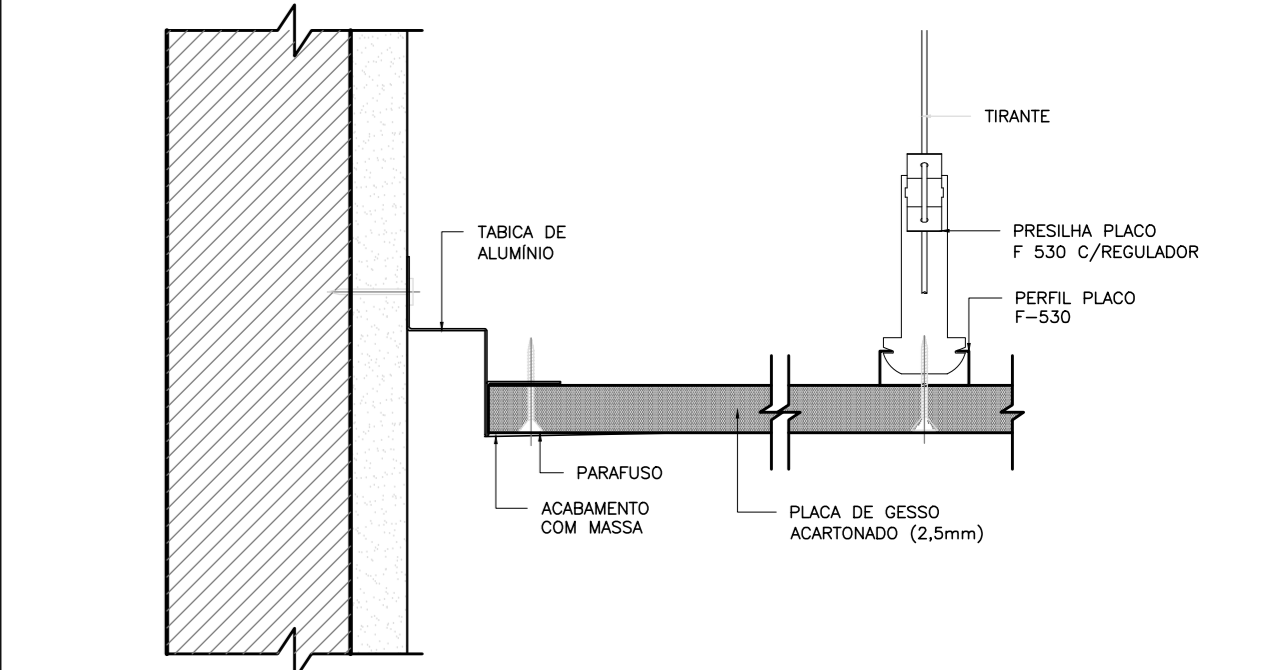
DETALHE TABICA FORRO DE GESSO ESQ: 1/2 MEDIDAS CM
