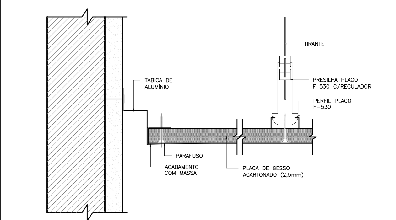
DETALHE TÁBICA FORRO DE GESSO ESC: 1/2 MEDIDAS CM
