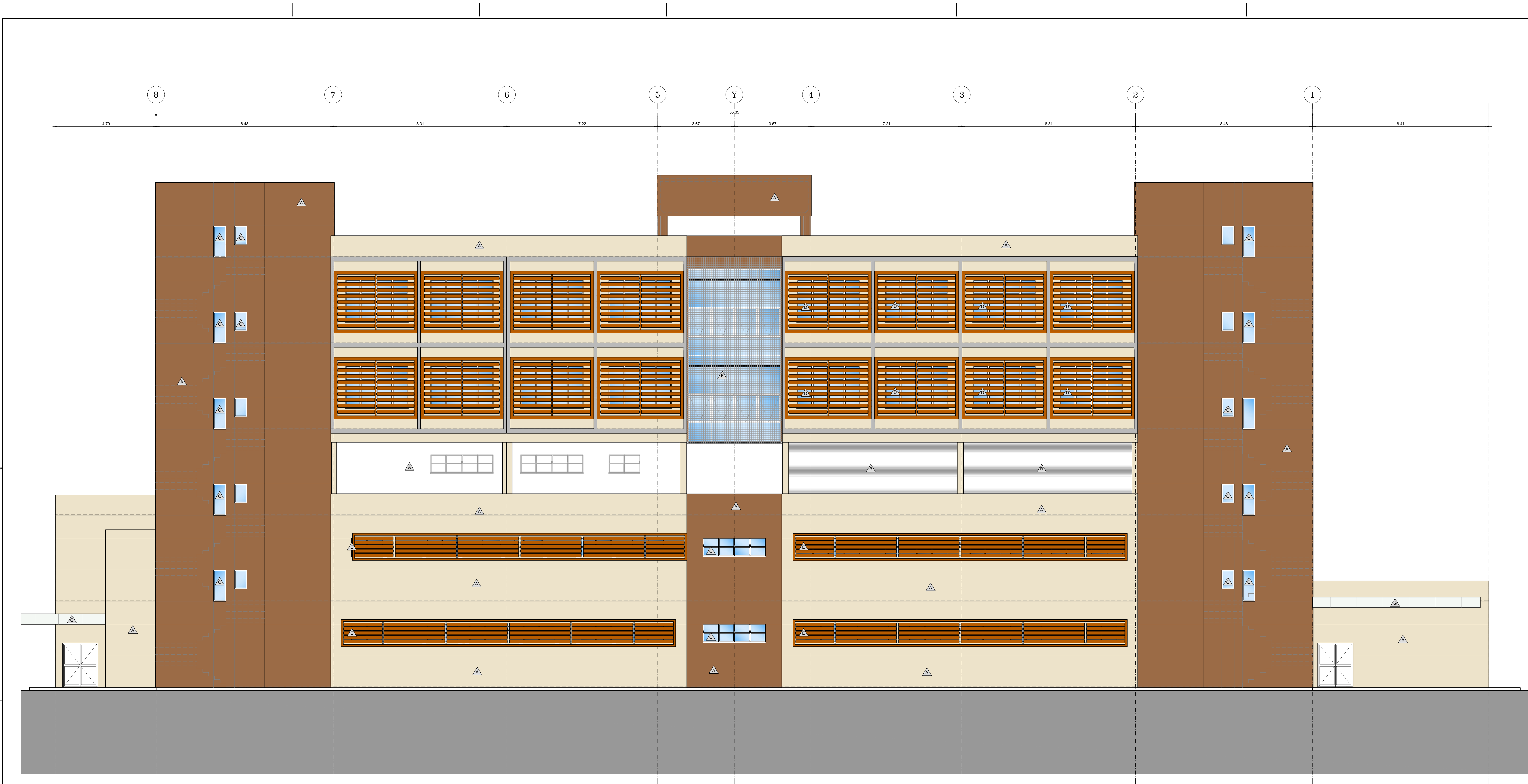
ELEVAÇÃO 02 ESC. 1:75
