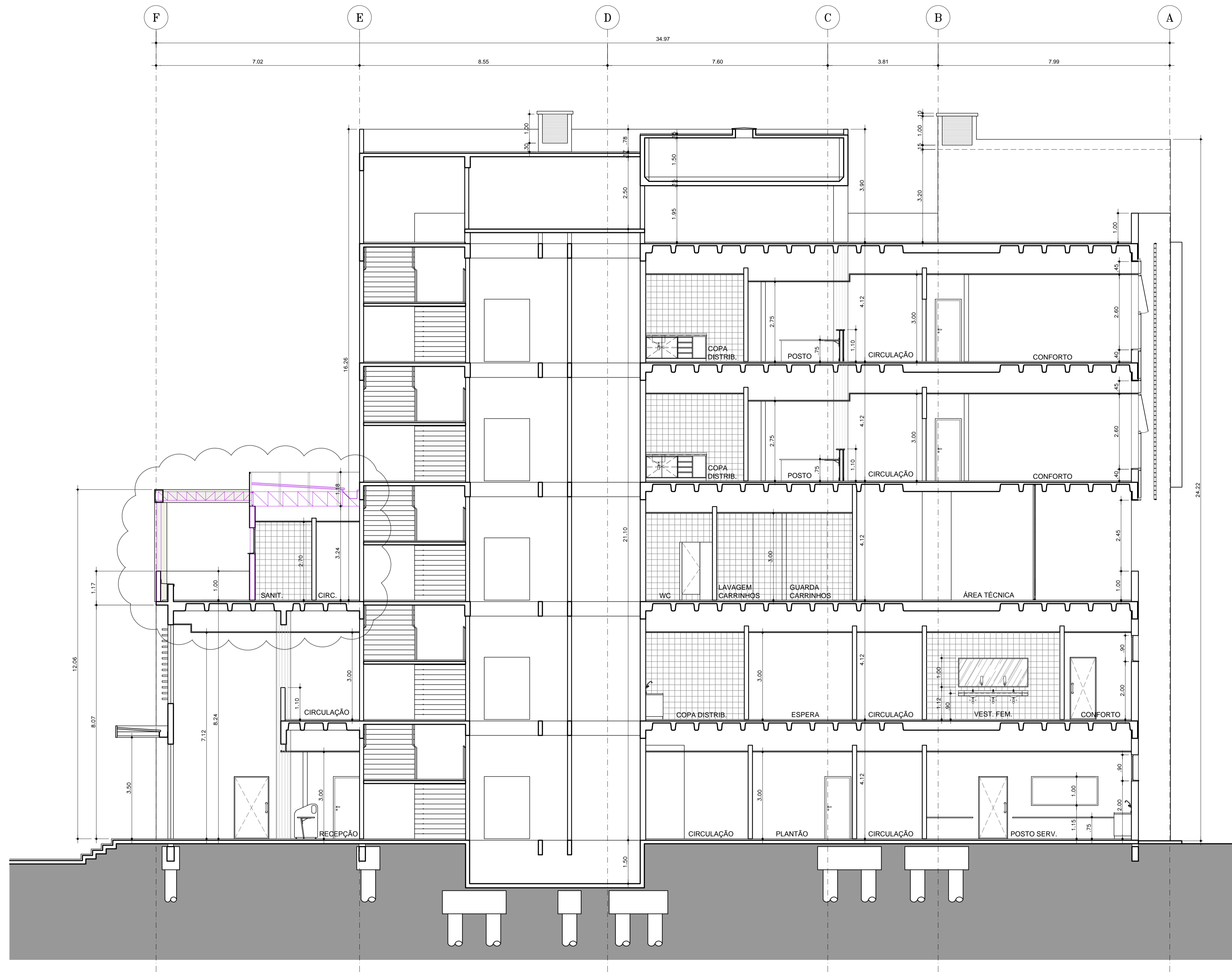
CORTE BB ESC. 1:75
