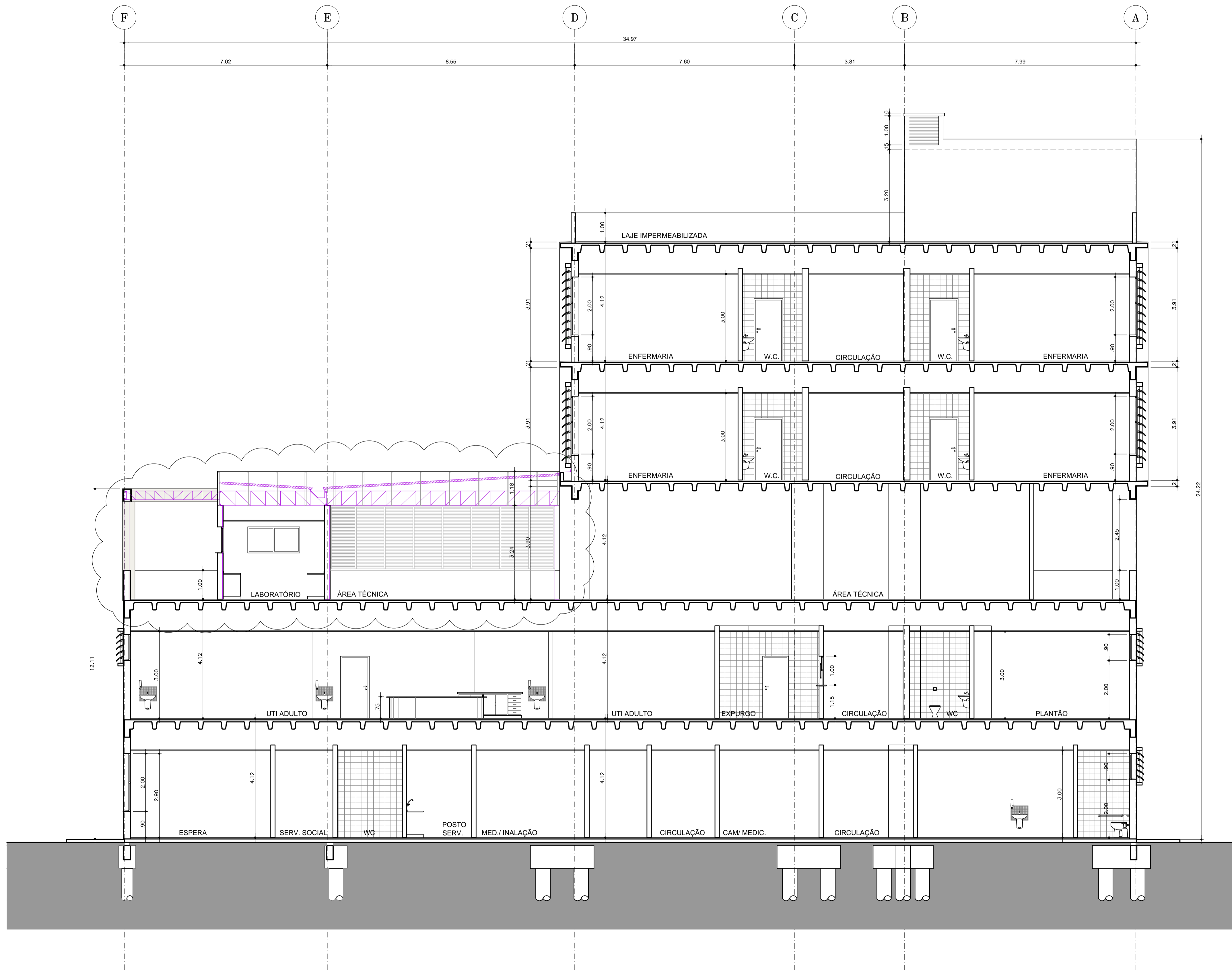
CORTE AA ESC. 1:75
