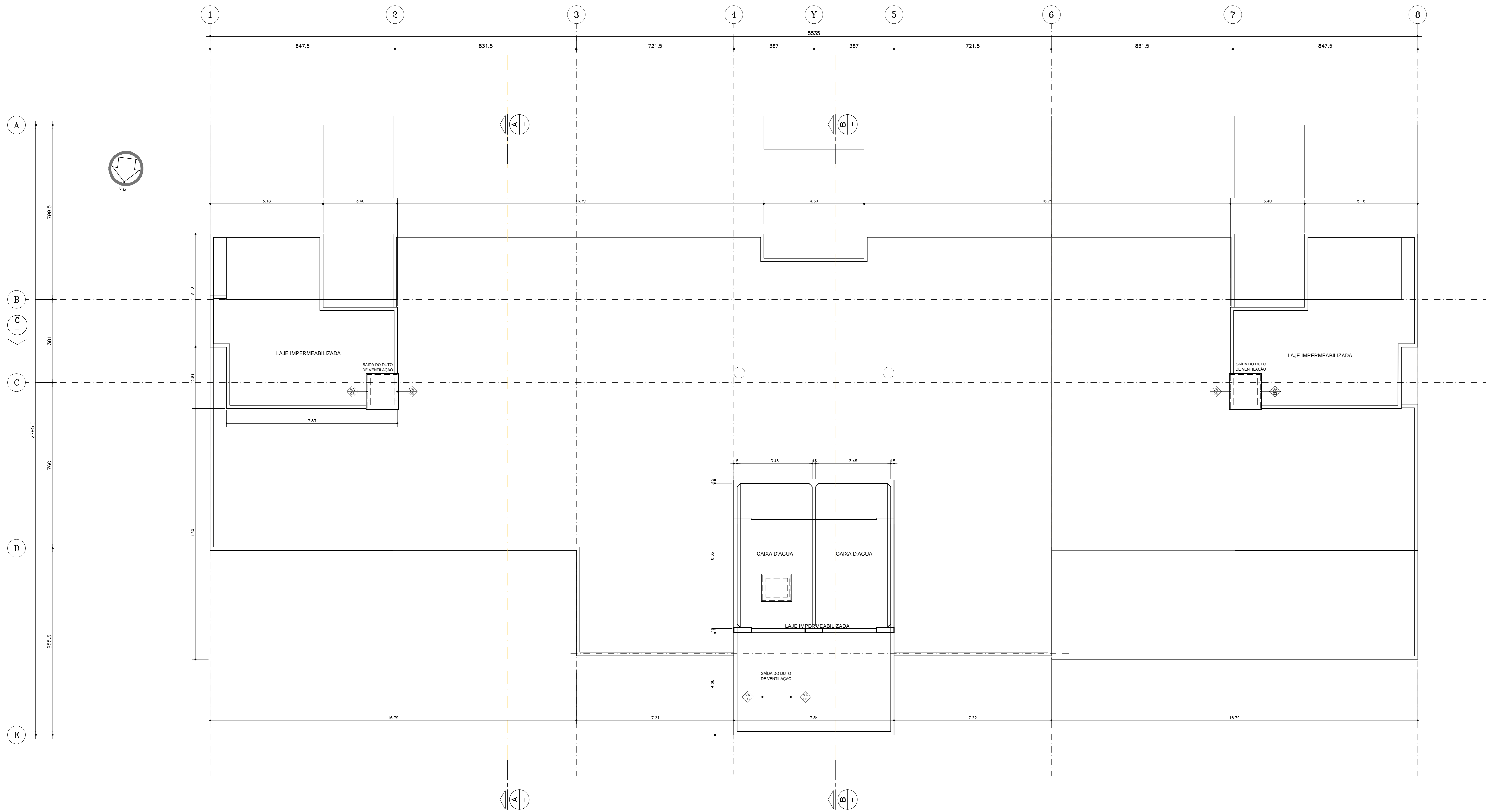
PLANTA DE LAYOUT - COBERTURA/ CAIXA D'AGUA ESC. 1:75
