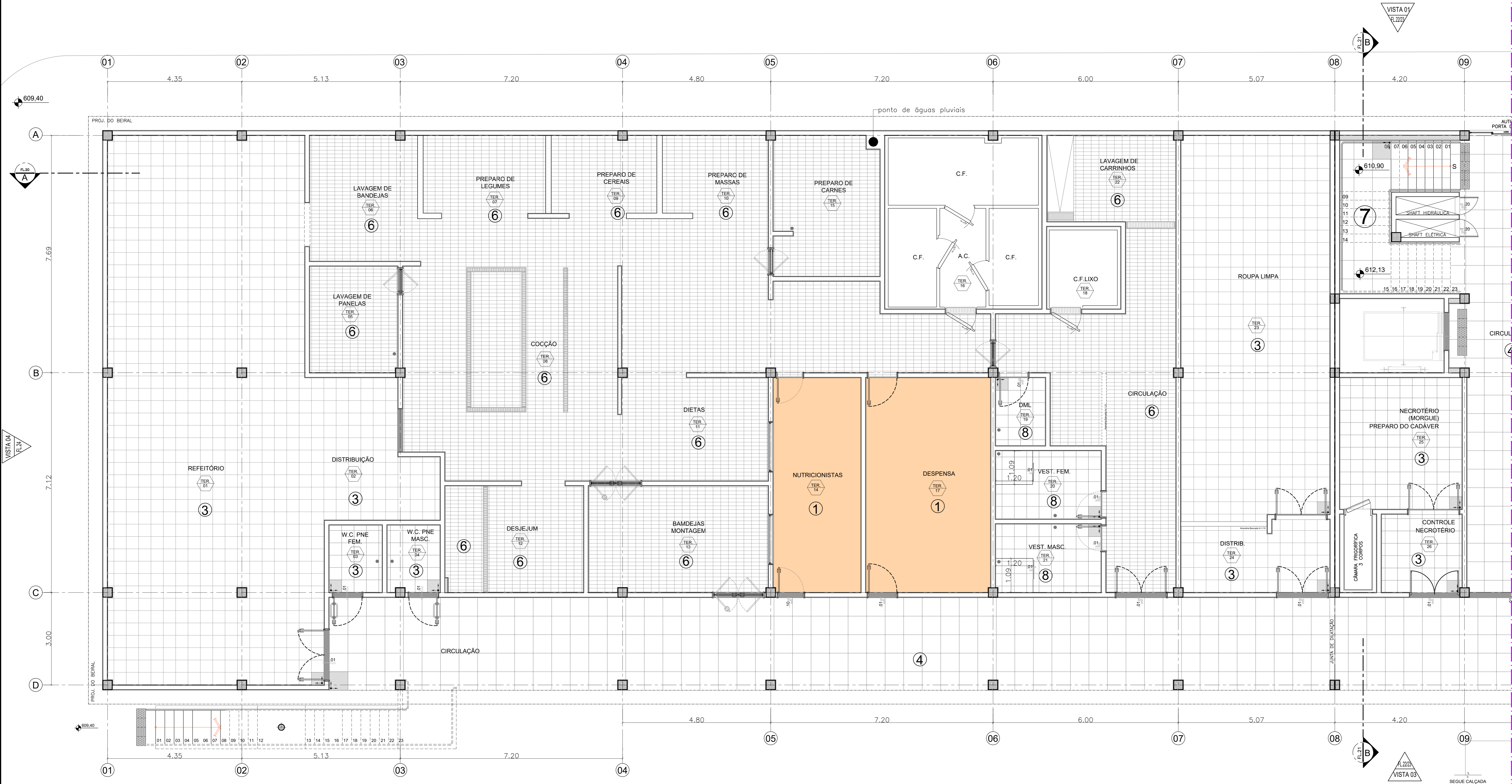
BLOCO 2 - PLANTA PISO PAVIMENTO TÉRREO ESC 1:50
