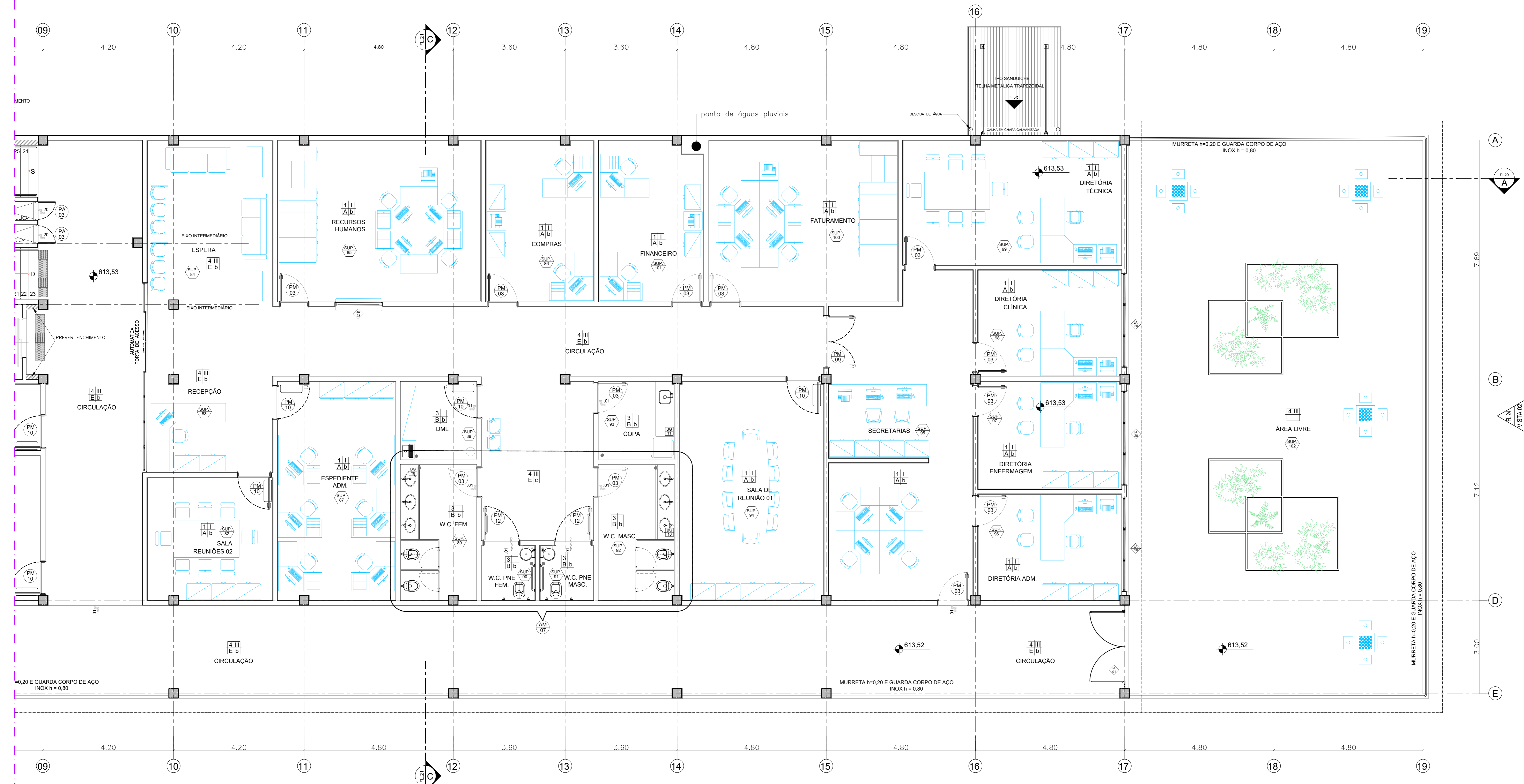
BLOCO 2 - PLANTA PAVIMENTO SUPERIOR ESC 1:50
