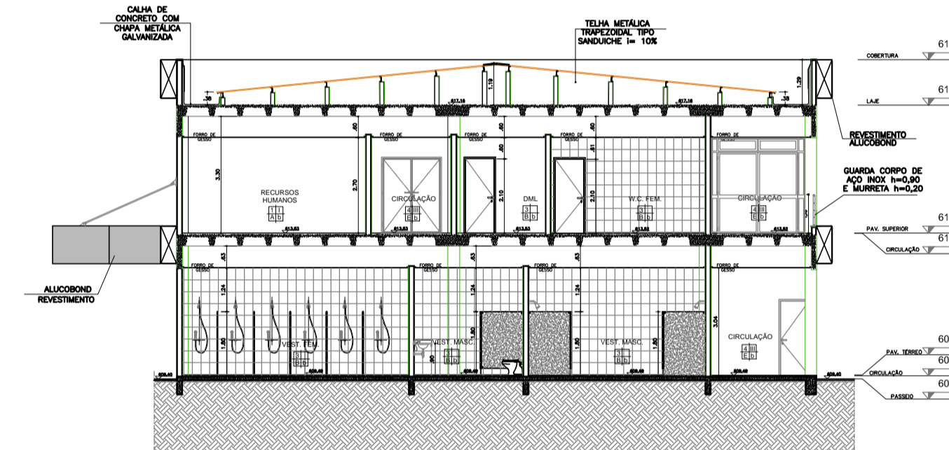
CORTE CC - BLOCO 02
