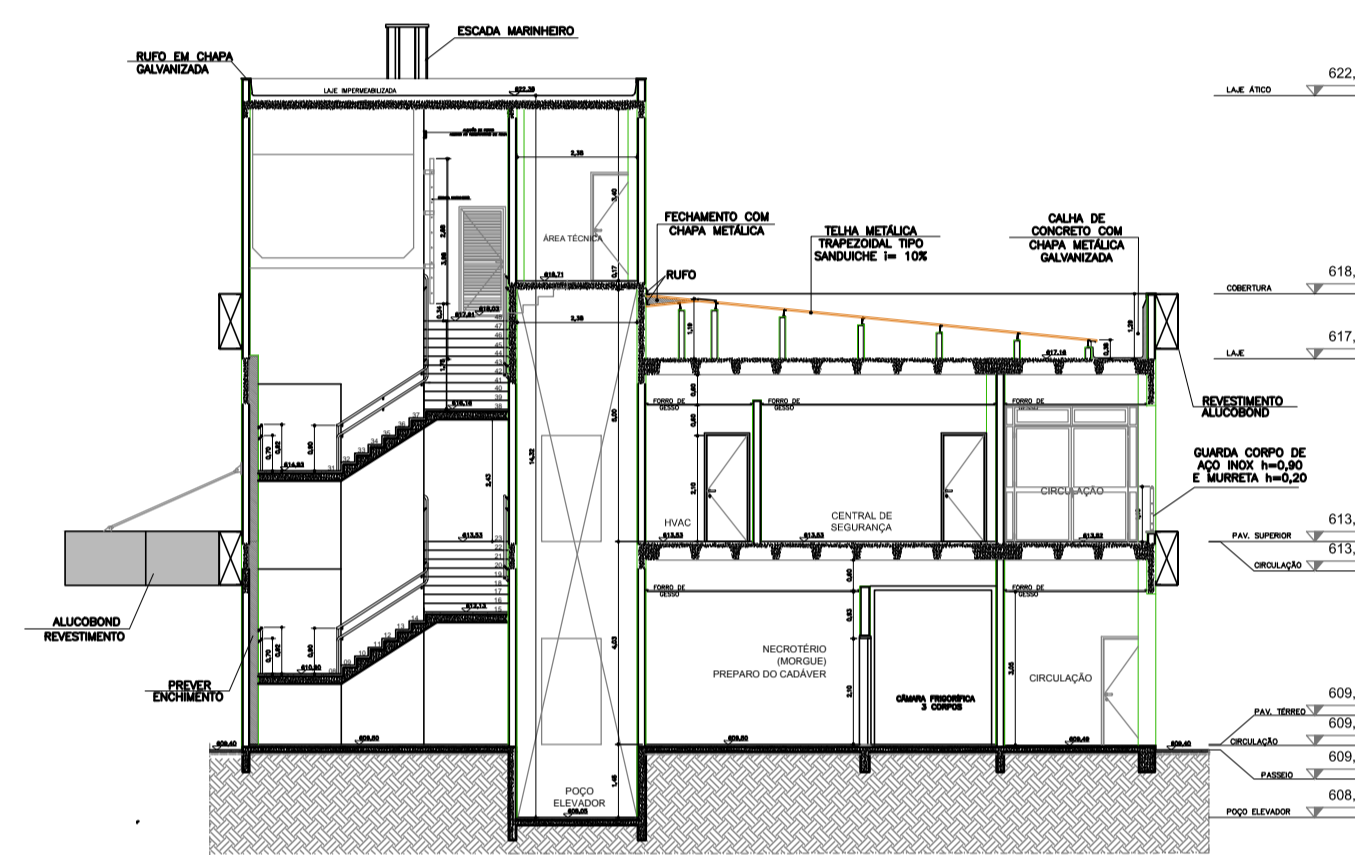
CORTE BB - BLOCO 02
