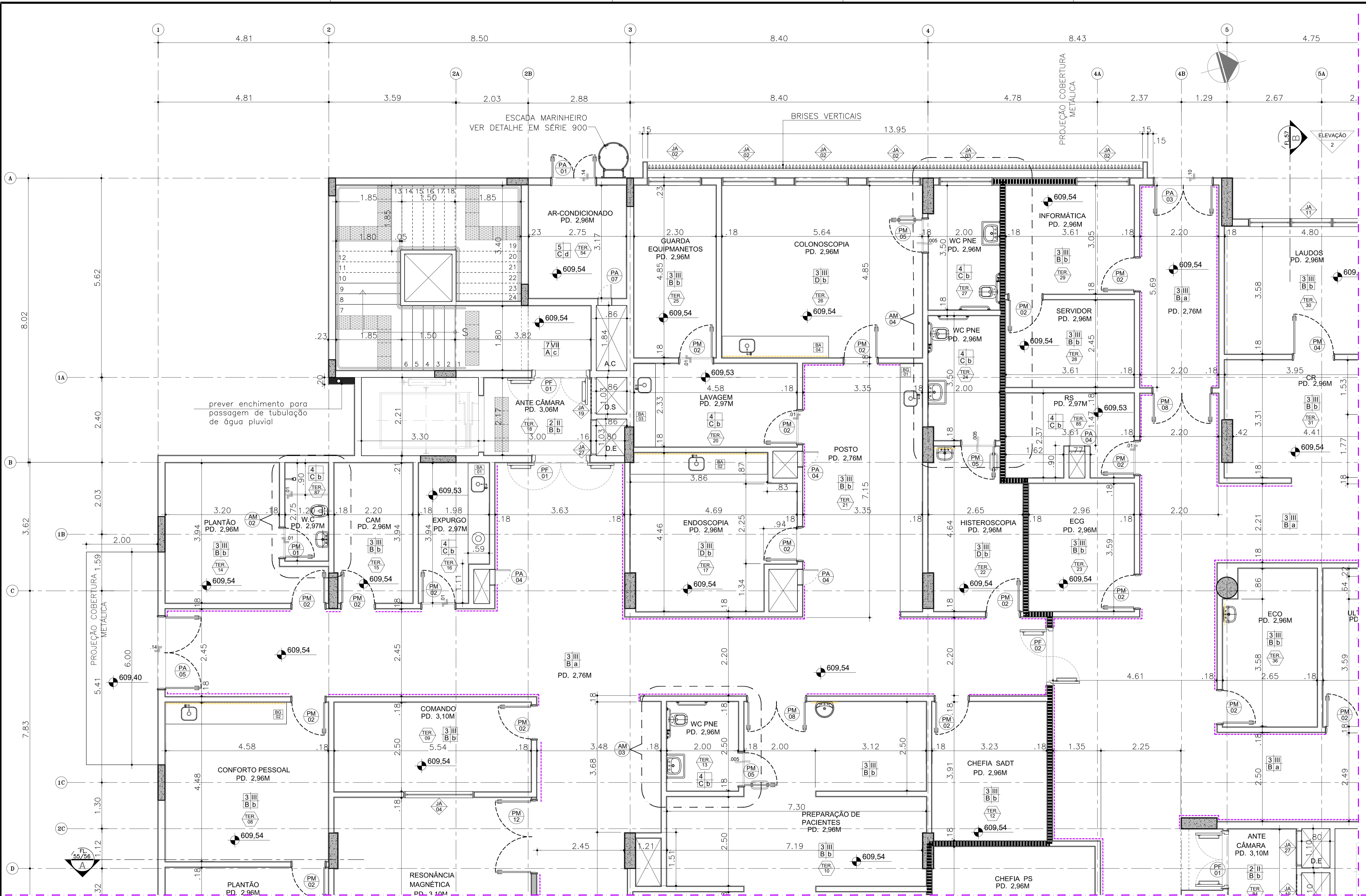
PLANTA ALVENARIA BLOCO 1 - TÉRREO ESC 1:50
