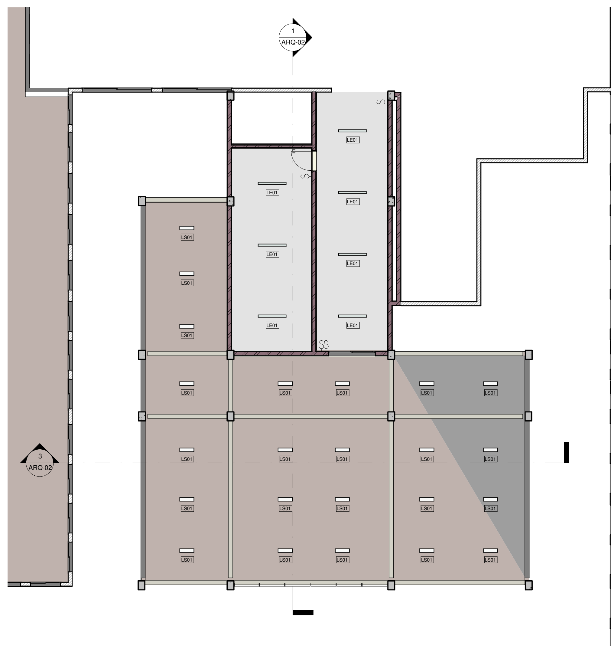
2 Térreo - Luminotécnica 1 : 100
