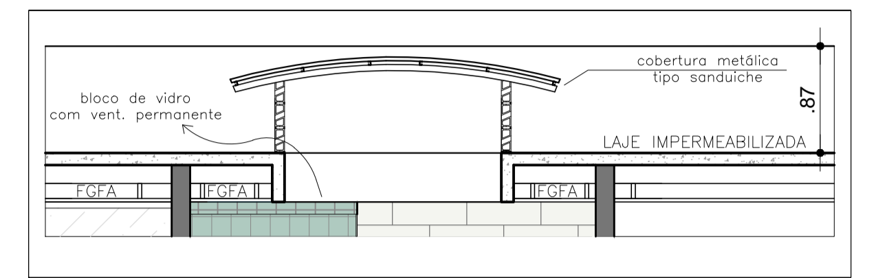
DETALHE 02: SHED SEM ESCALA
