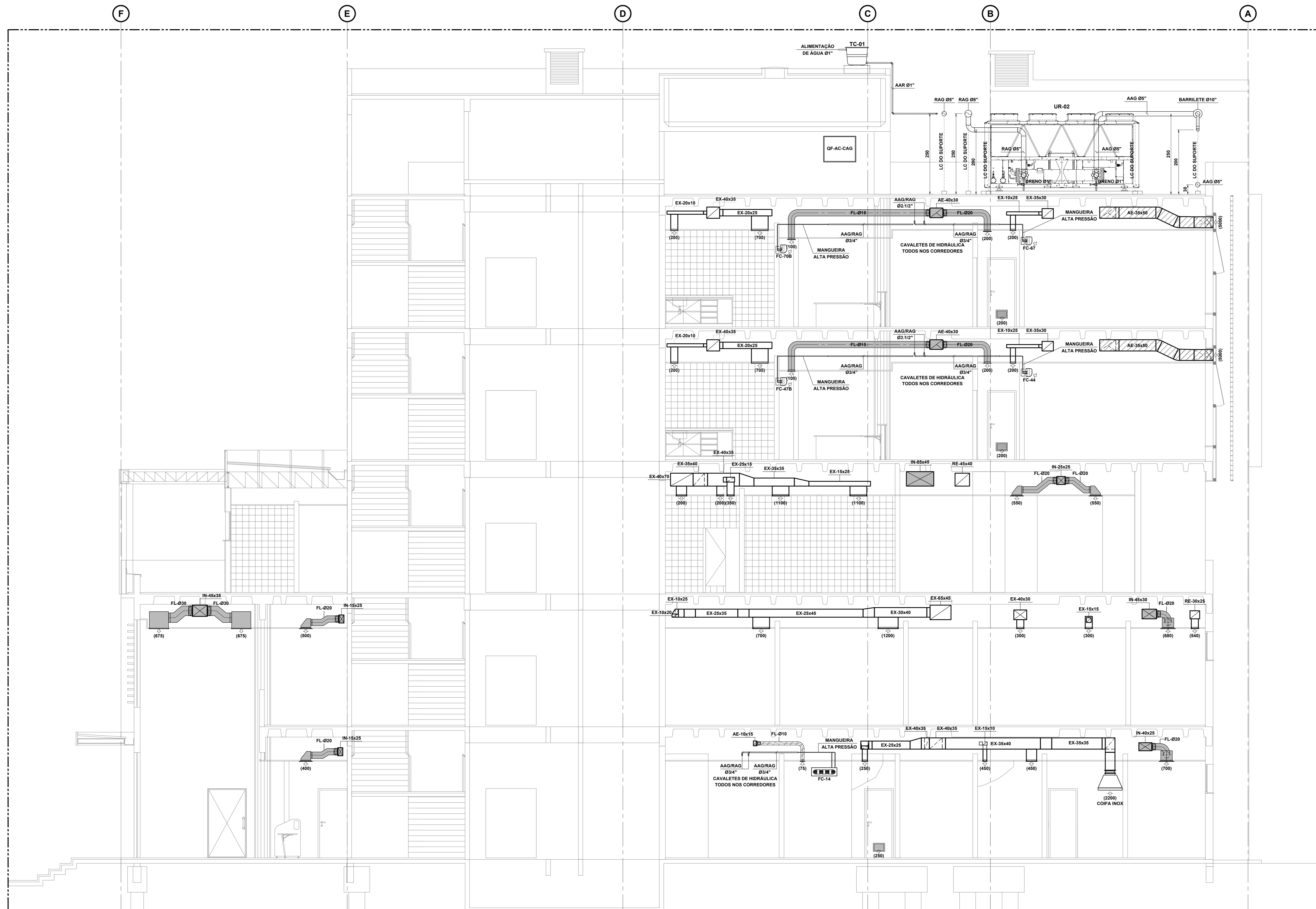
CORTE - BB ESCALA 1:50
