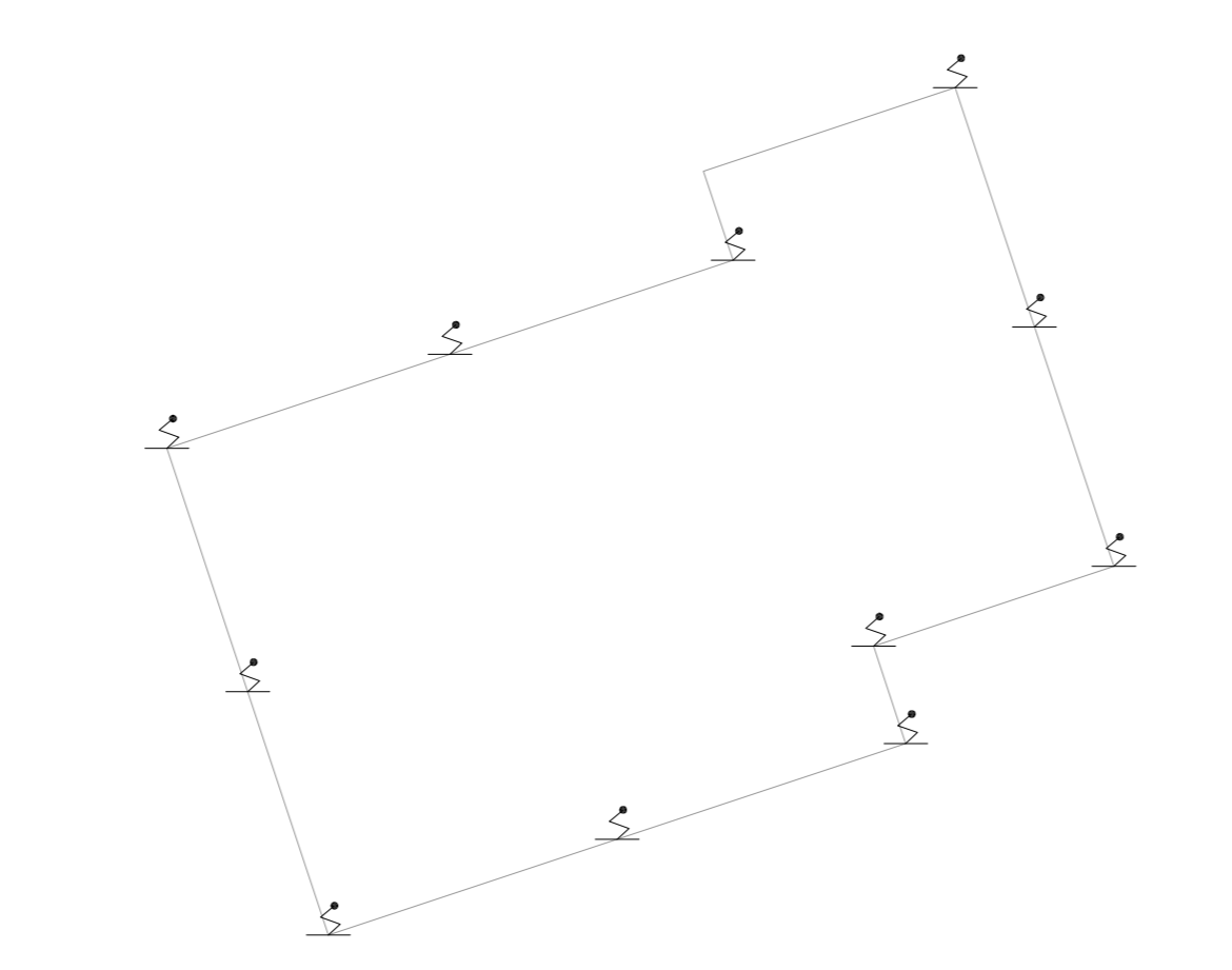
5 HFRA - MANUTENÇÃO II PROJETO BÁSICO DOS SISTEMAS DE INCÊNDIO PLANTA BAIXA - COBERTURA ESCALA 1:100 METRO
