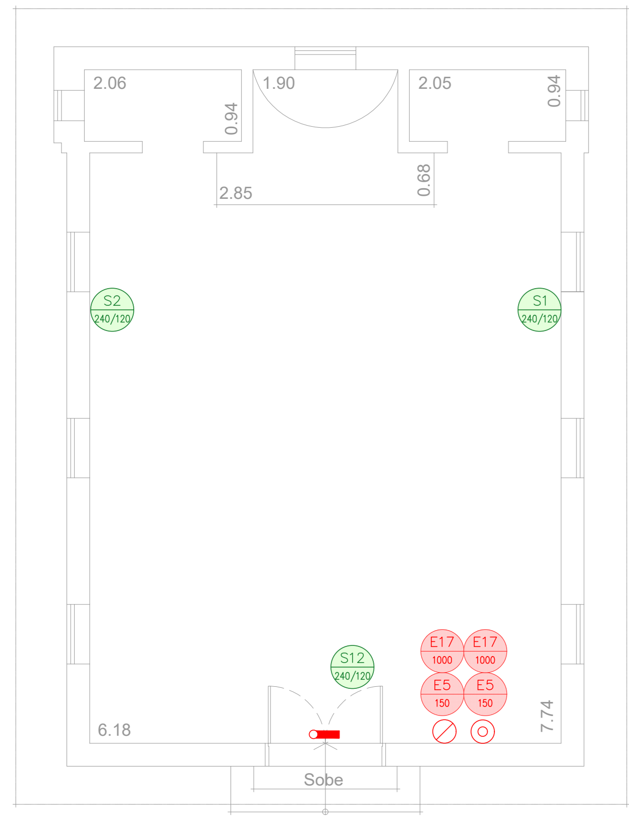
5 CAISM PHILIPPE PINEL - EDIFÍCIO 5 PROJETO BÁSICO DOS SISTEMAS DE INCÊNDIO PLANTA BAIXA - CAPELA ESCALA: 1:50 METRO
