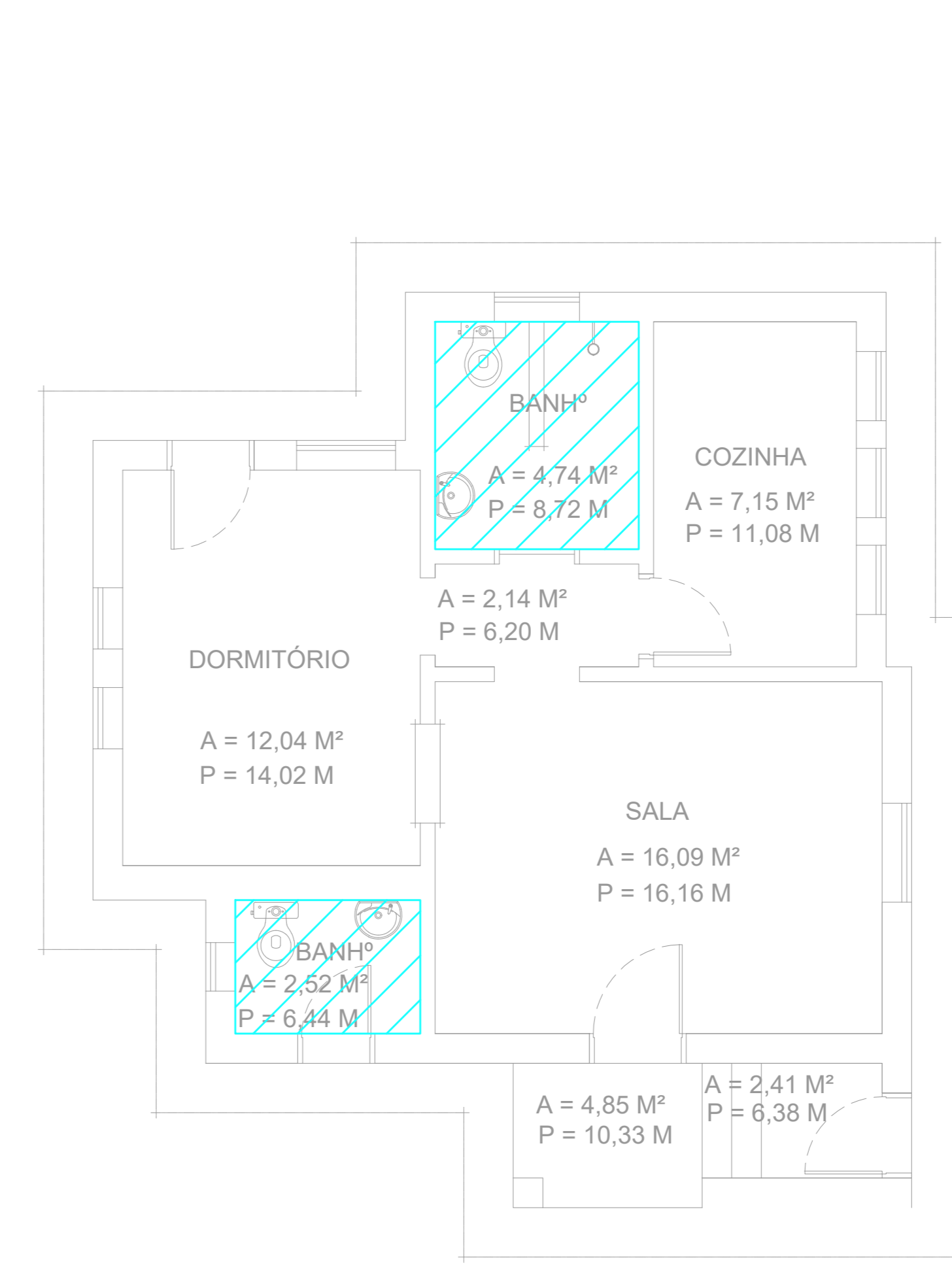
4 CAISM PHILIPPE PINEL - EDIFÍCIO 1 PROJETO BÁSICO DOS SISTEMAS DE INCÊNDIO PLANTA BAIXA - SAÚDE ESCALA: 1:50 METRO
