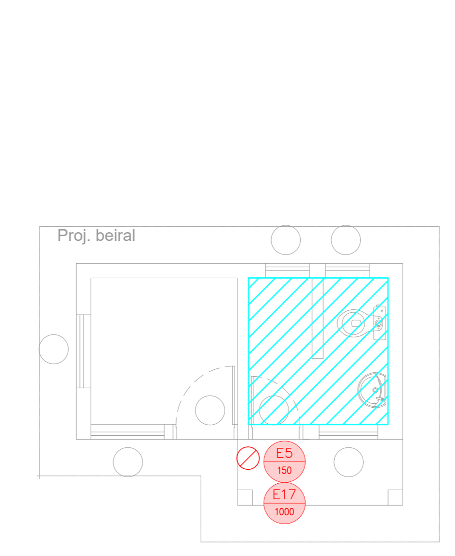
8 CAISM PHILIPPE PINEL - EDIFÍCIO 8 PROJETO BÁSICO DOS SISTEMAS DE INCÊNDIO PLANTA BAIXA - PORTARIA 1 ESCALA: 1:50 METRO
