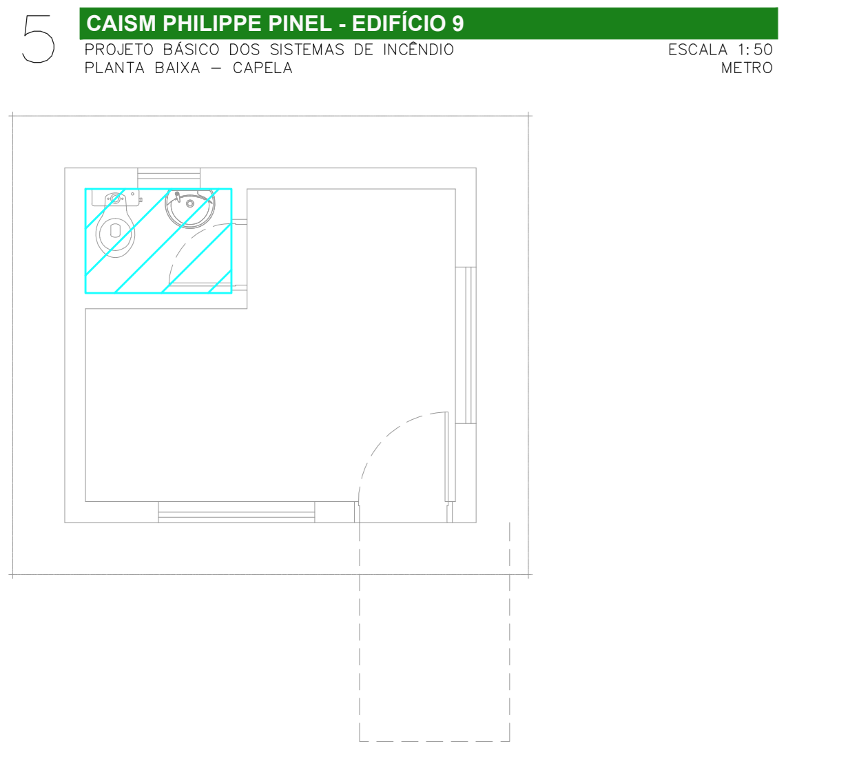
9 CAISM PHILIPPE PINEL - EDIFÍCIO 9 PROJETO BÁSICO DOS SISTEMAS DE INCÊNDIO PLANTA BAIXA - VESTIÁRIO ESCALA: 1:50 METRO
