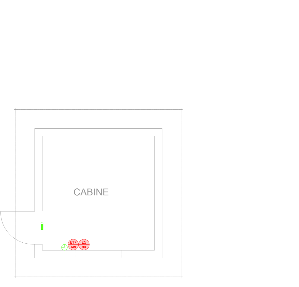
6 CAISM PHILIPPE PINEL - EDIFÍCIO 2 PROJETO BÁSICO DOS SISTEMAS DE INCÊNDIO PLANTA BAIXA - CABINE PRIMÁRIA ESCALA: 1:50 METRO
