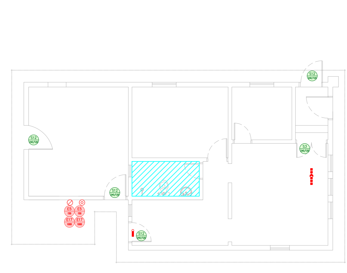
7 CAISM PHILIPPE PINEL - EDIFÍCIO 3 PROJETO BÁSICO DOS SISTEMAS DE INCÊNDIO PLANTA BAIXA - PORTARIA PRINCIPAL DESATIVADA ESCALA: 1:75 METRO
