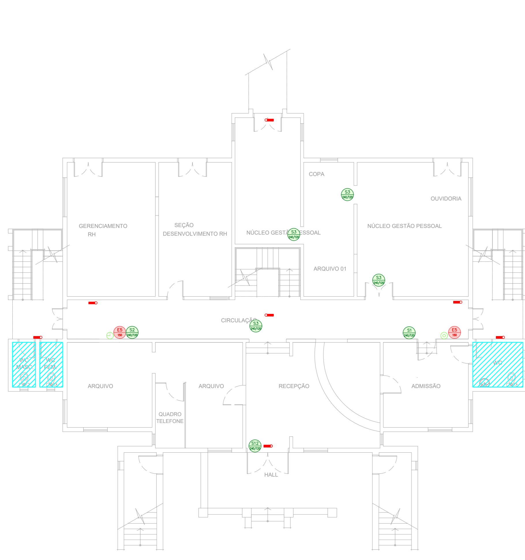
1 CAISM PHILIPPE PINEL - EDIFÍCIO 7 PROJETO BÁSICO DOS SISTEMAS DE INCÊNDIO PLANTA BAIXA - ADMINISTRATIVO SUPERIOR ESCALA: 1:100 METRO
