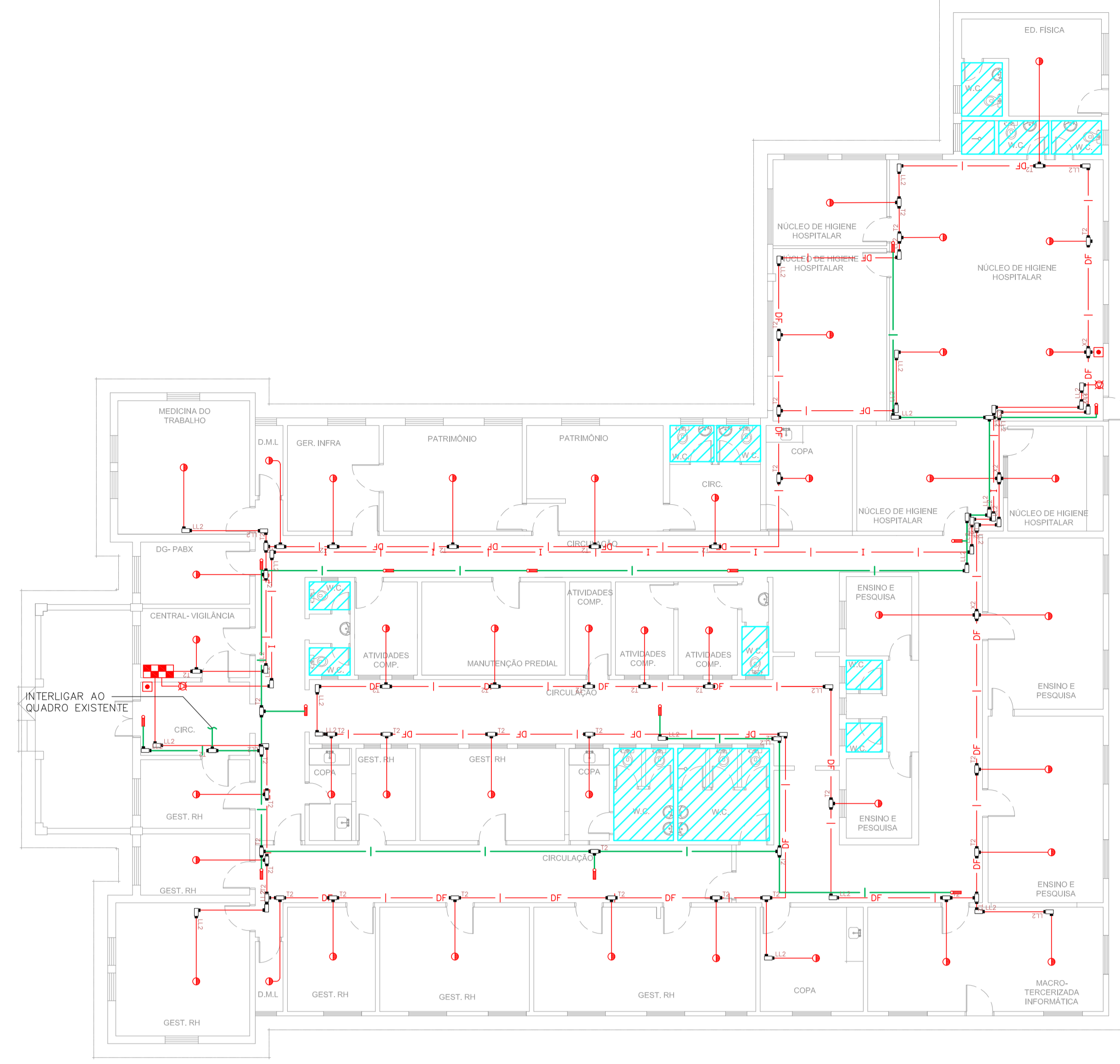
2 CAISM PHILIPPE PINEL - EDIFÍCIO 33 PROJETO BÁSICO DOS SISTEMAS DE INCÊNDIO PLANTA BAIXA - CENTRAL ESCALA: 1:125 METRO
