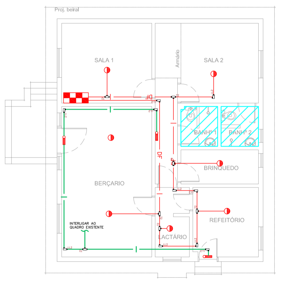
7 CAISM PHILIPPE PINEL - EDIFÍCIO 30 PROJETO BÁSICO DOS SISTEMAS DE INCÊNDIO PLANTA BAIXA - CASA 2 CREAPP ESCALA: 1:100 METRO
