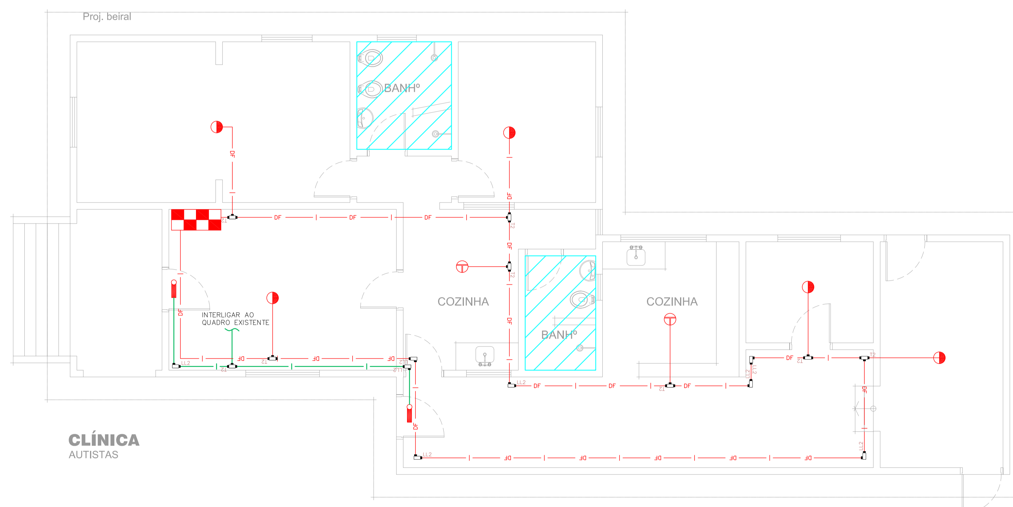
5 CAISM PHILIPPE PINEL - EDIFÍCIO 31 PROJETO BÁSICO DOS SISTEMAS DE INCÊNDIO PLANTA BAIXA - CASA 3 CREAPP CLÍNICA AUTISTAS ESCALA: 1:100 METRO
