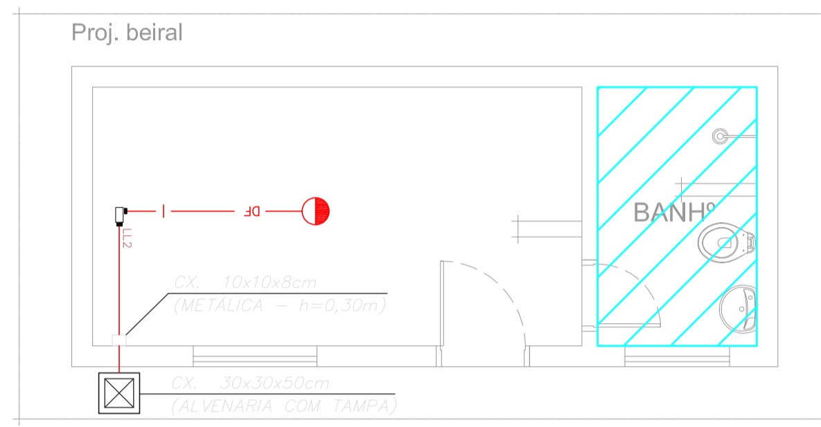
4 CAISM PHILIPPE PINEL - EDIFÍCIO 31 PROJETO BÁSICO DOS SISTEMAS DE INCÊNDIO PLANTA BAIXA - CASA 3 CREAPP ESCALA: 1:50 METRO
