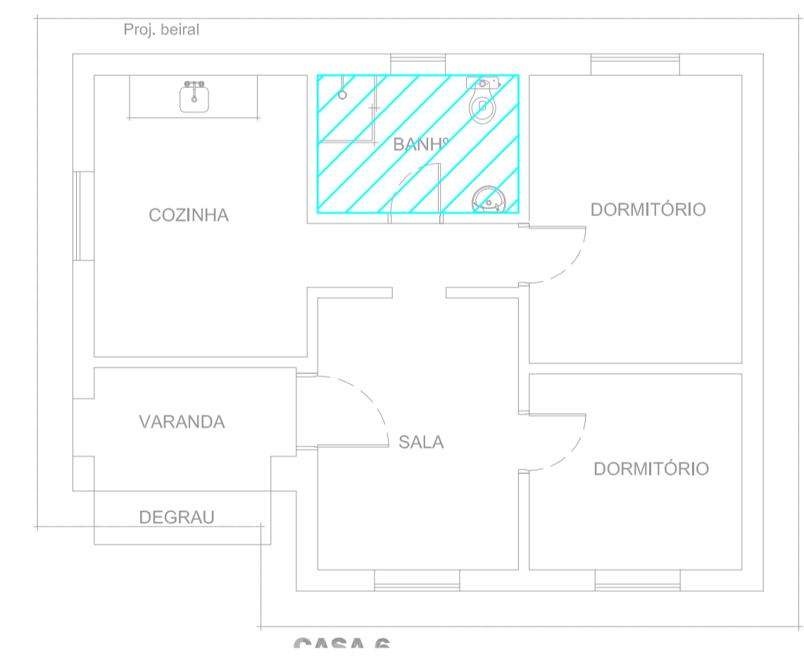
6 CAISM PHILIPPE PINEL - EDIFÍCIO 32 PROJETO BÁSICO DOS SISTEMAS DE INCÊNDIO PLANTA BAIXA - CASA 6 QUADRUA ESCALA: 1:75 METRO
