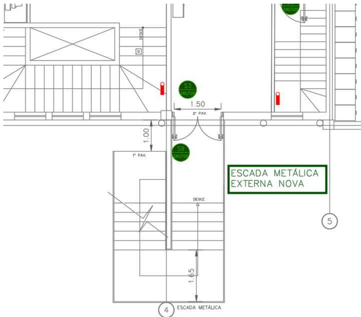
Figura 21 – PLANTA DA NOVA ESCADA METÁLICA – CHEGADA AO 2ºPAVIMENTO
