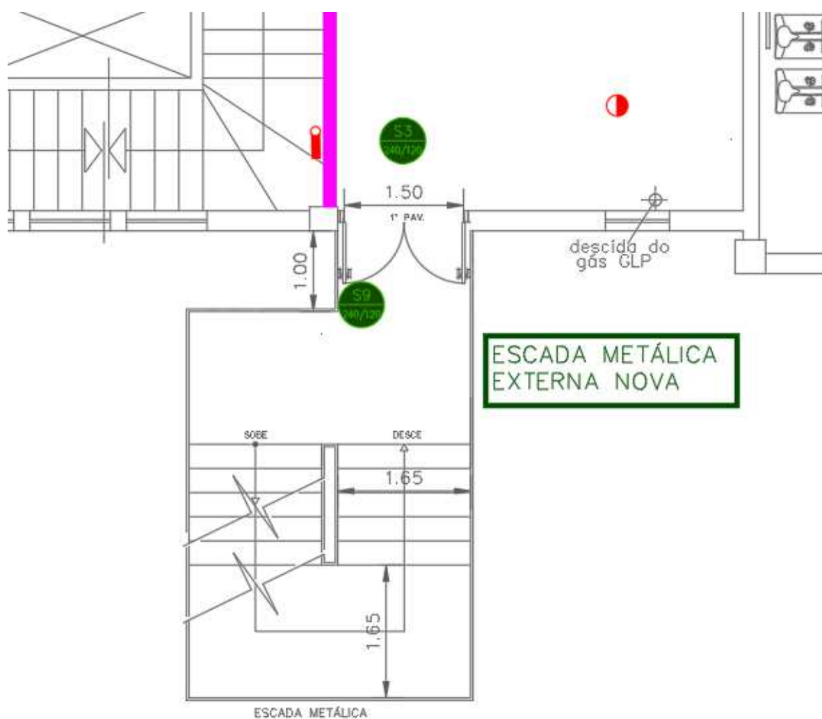
Figura 20 – PLANTA DA NOVA ESCADA METÁLICA – SAÍDA DO 1ºPAVIMENTO AO 2ºPAVIMENTO
