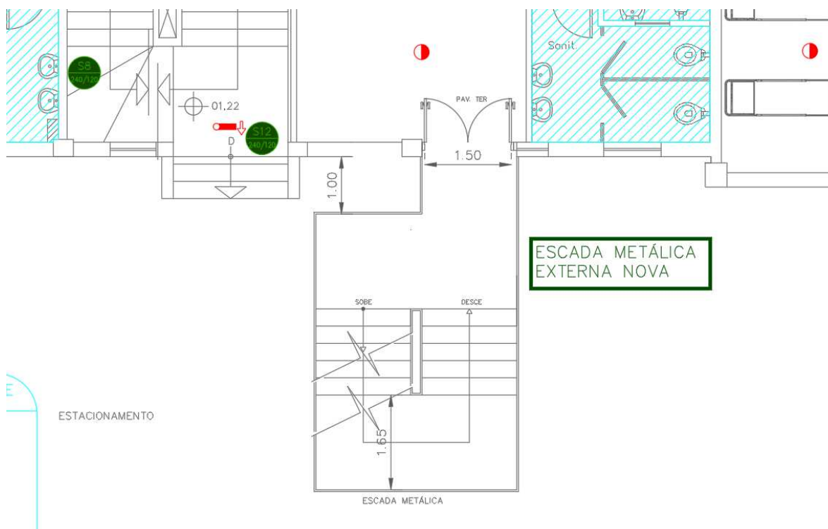
Figura 19 – PLANTA DA NOVA ESCADA METÁLICA – SAÍDA DO TÉRREO AO 1º PAVIMENTO
