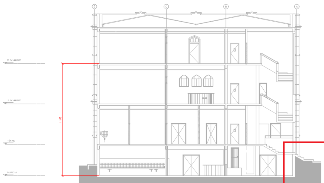
Figura 16 – CORTE DA ESTRUTURA EXISTENTE
