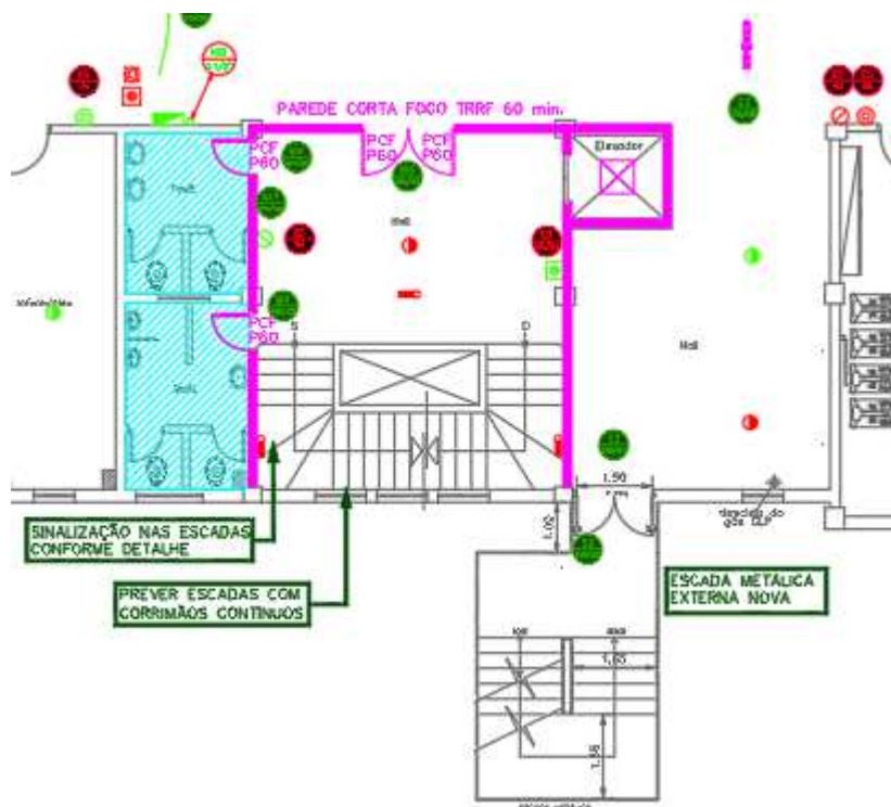
Figura 5 – 1º PAVIMENTO – Paredes corta fogo
