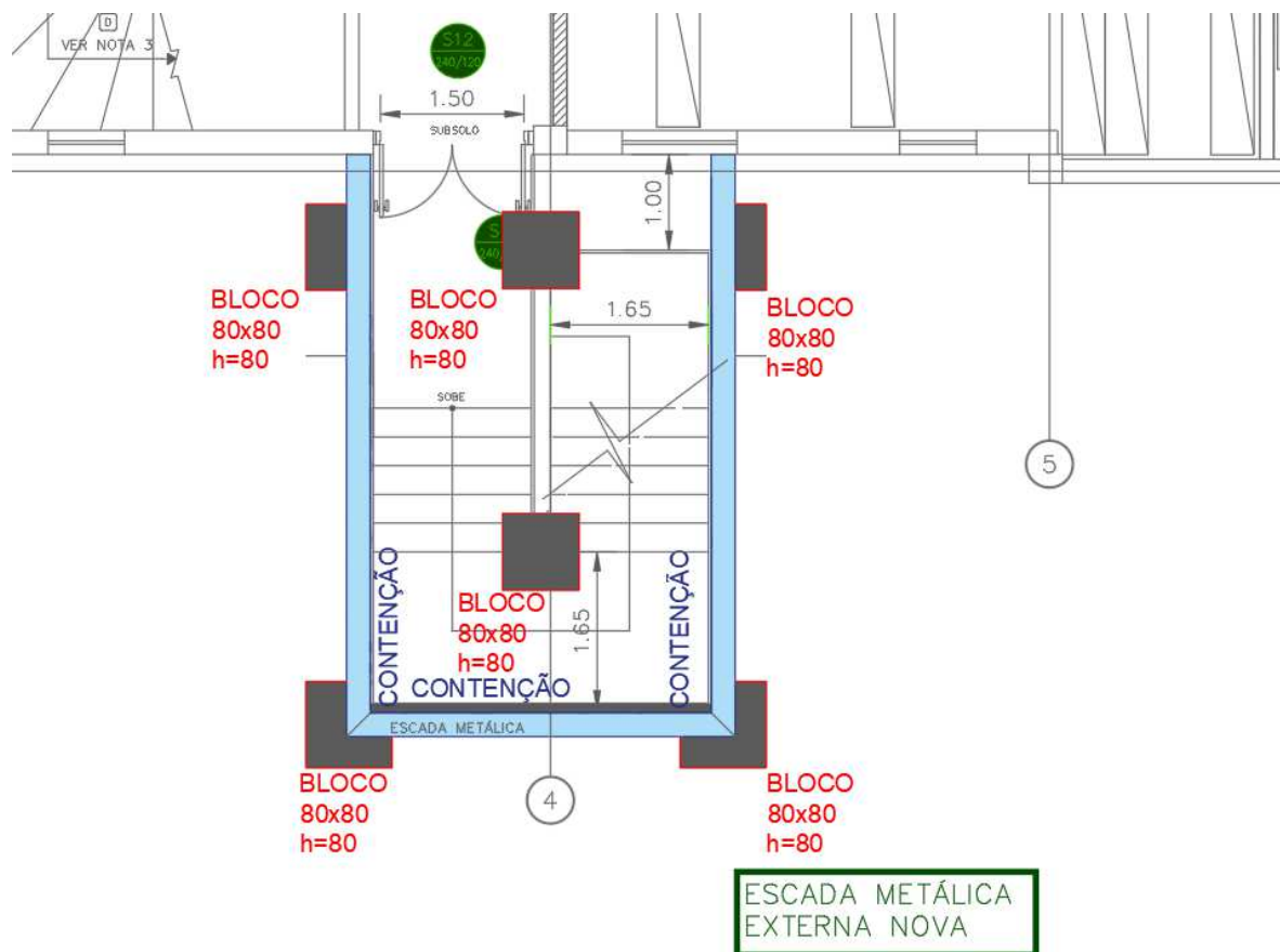
Figura 18 – PLANTA DA NOVA ESCADA METÁLICA COM PROJEÇÃO DA ESTRUTURA DE CONCRETO – SAÍDA DO SUBSOLO AO TÉRREO
