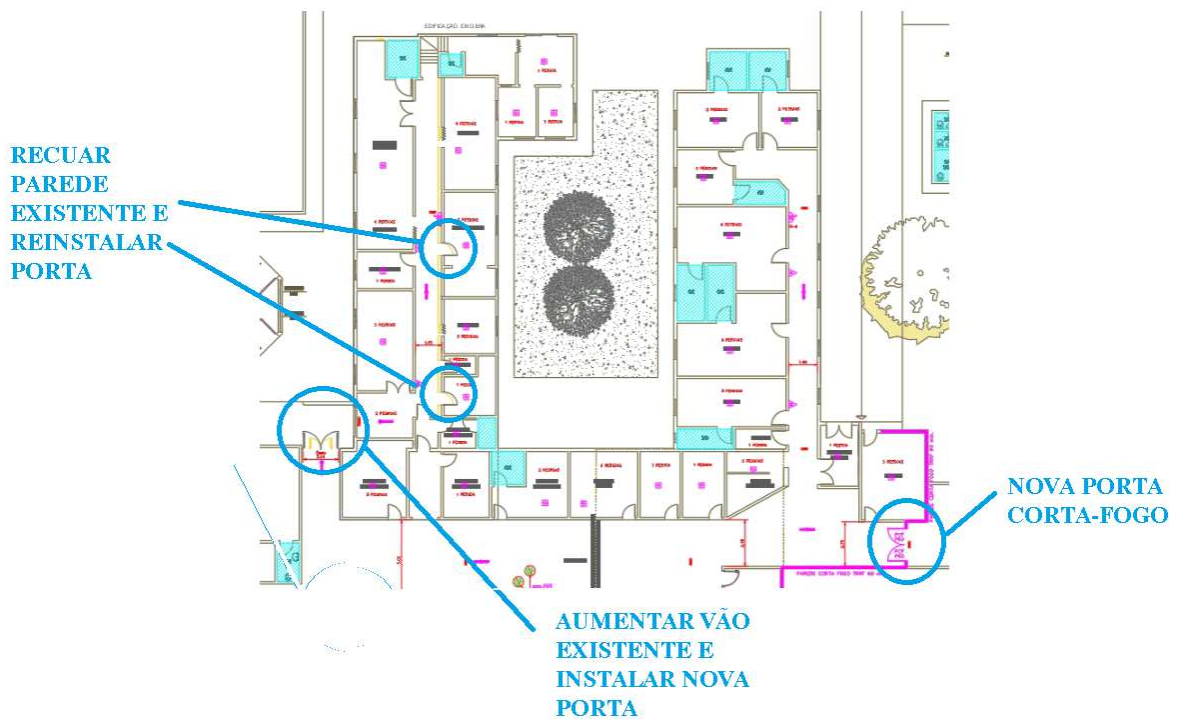
Figura 7 – PAVIMENTO TÉRREO – Reposicionamento/instalação portas
