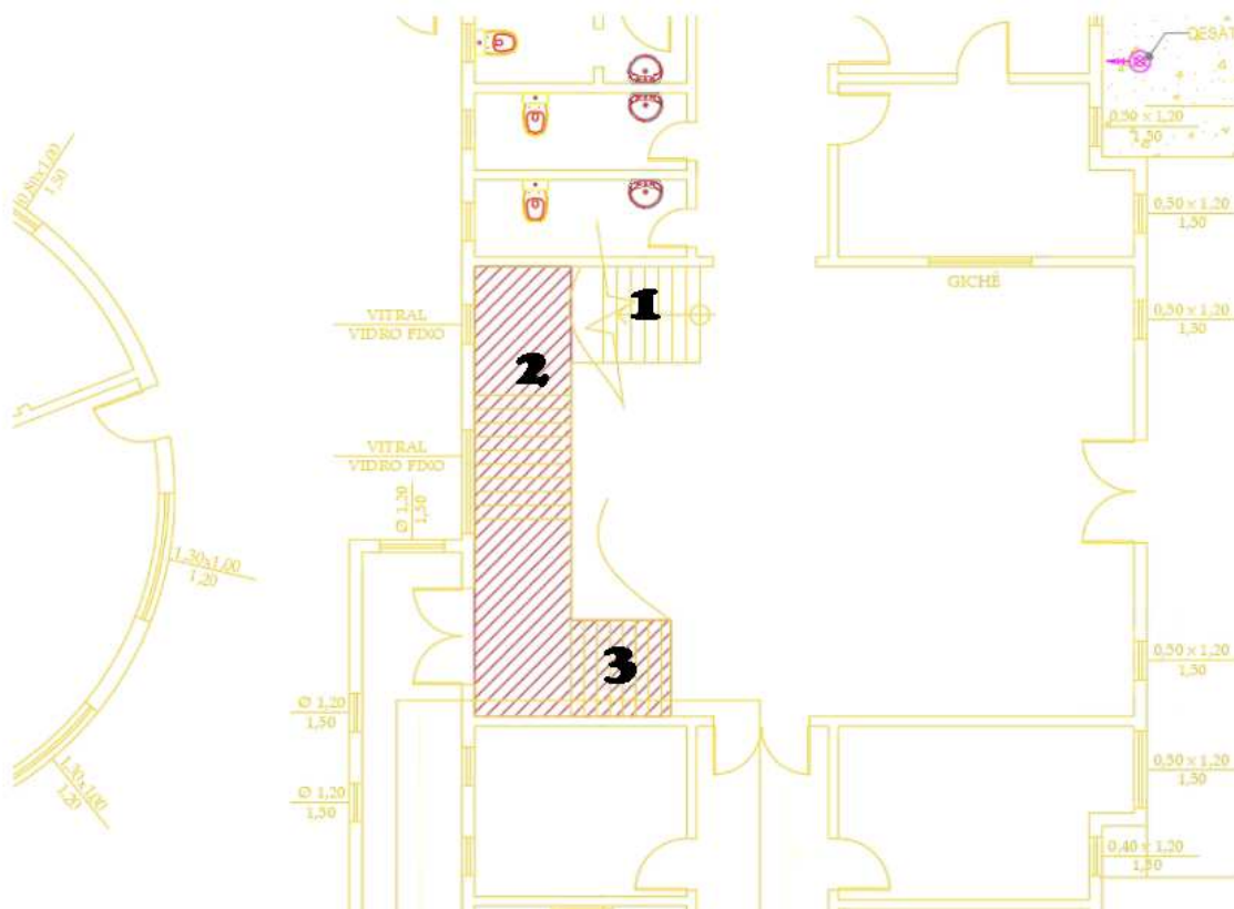
Figura 17 – LEVANTAMENTO TÉRREO – ESCADA A DEMOLIR/RECONSTRUIR
