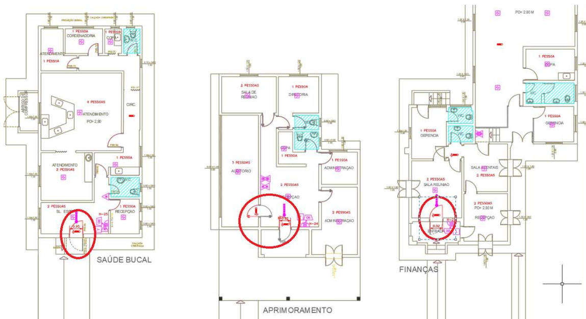
Figura 3 – PAVIMENTO TÉRREO – Inversão sentido de porta
