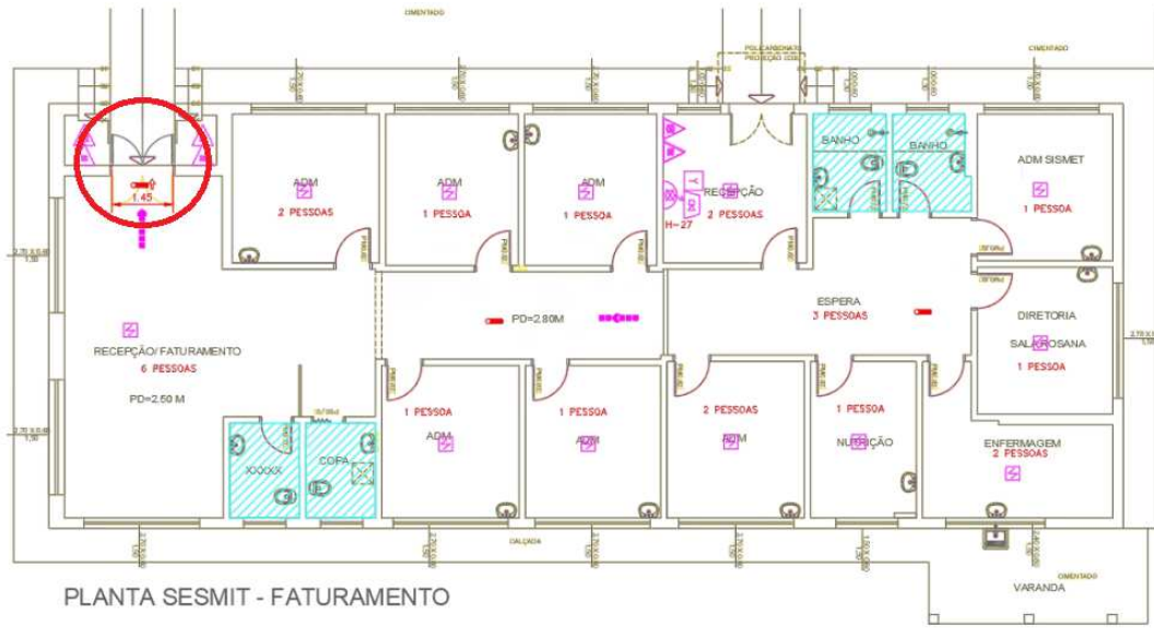
Figura 2 – PAVIMENTO TÉRREO – Inversão sentido de porta
