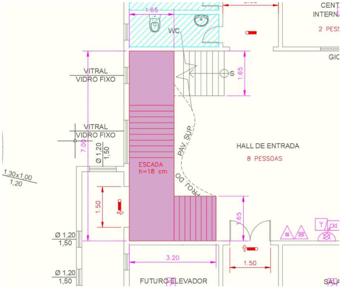
Figura 22 – ESTRUTURA DA NOVA ESCADA DE CONCRETO
