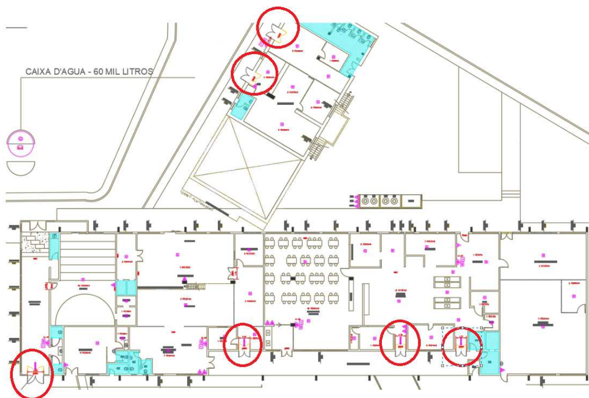
Figura 1 – PAVIMENTO TÉRREO – Inversão sentido de porta
