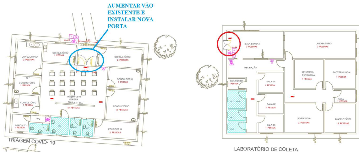
Figura 11 – PAVIMENTO TÉRREO – inversão de sentido e instalação de portas
