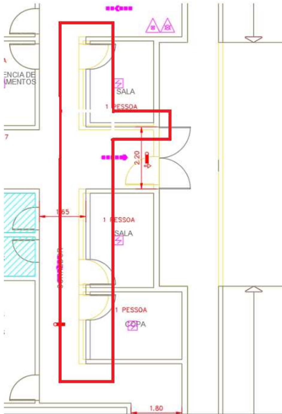
Figura 15 – PAVIMENTO TÉRREO – CORREDOR P.S. OFTALMOLOGIA – Demolição/reconstrução corredor
