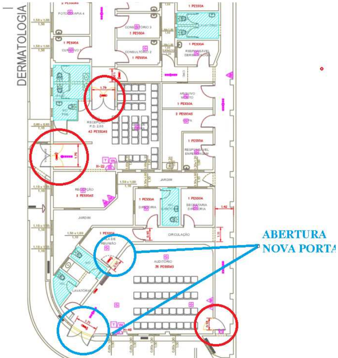
Figura 5 – PAVIMENTO TÉRREO – Inversão sentido de porta / abertura porta
