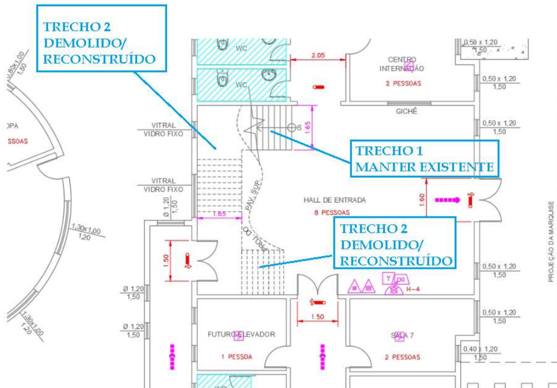
Figura 21 – NOVO LAYOUT DA ESCADA
