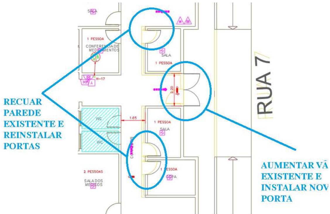
Figura 10 – PAVIMENTO TÉRREO – Reposicionamento/instalação de portas
