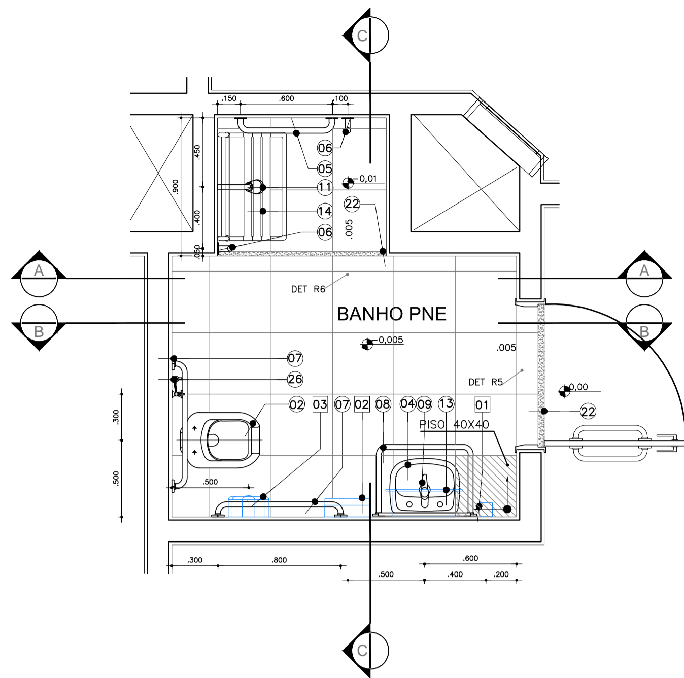
AM-25- SANITÁRIOS QUARTOS ENFERMARIA QUANTIDADE : ESC.: 1:25
