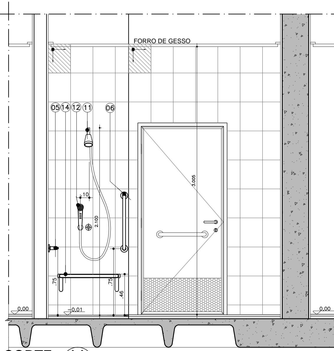
CORTE AA ESCALA 1:25
