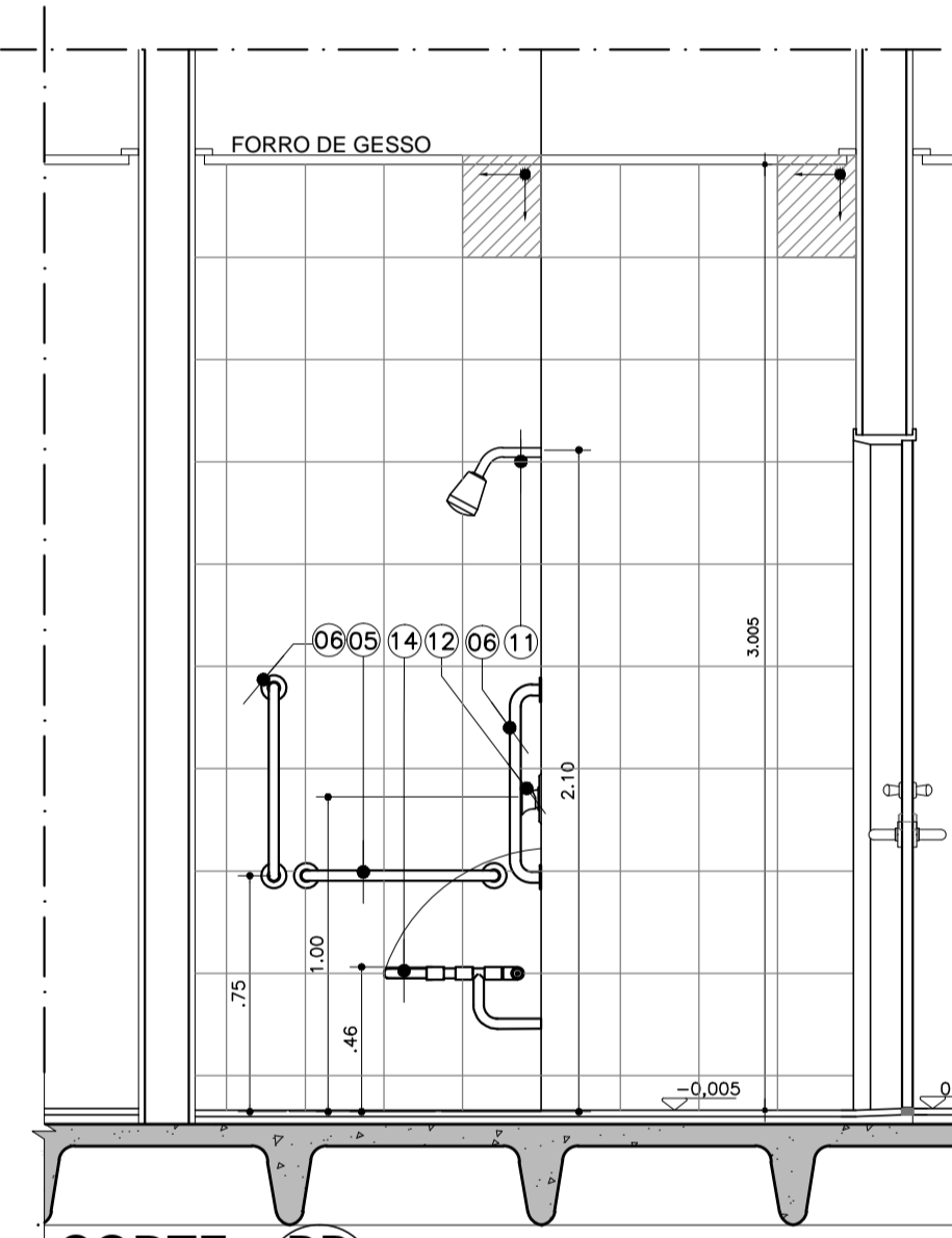
CORTE BB ESCALA 1:25
