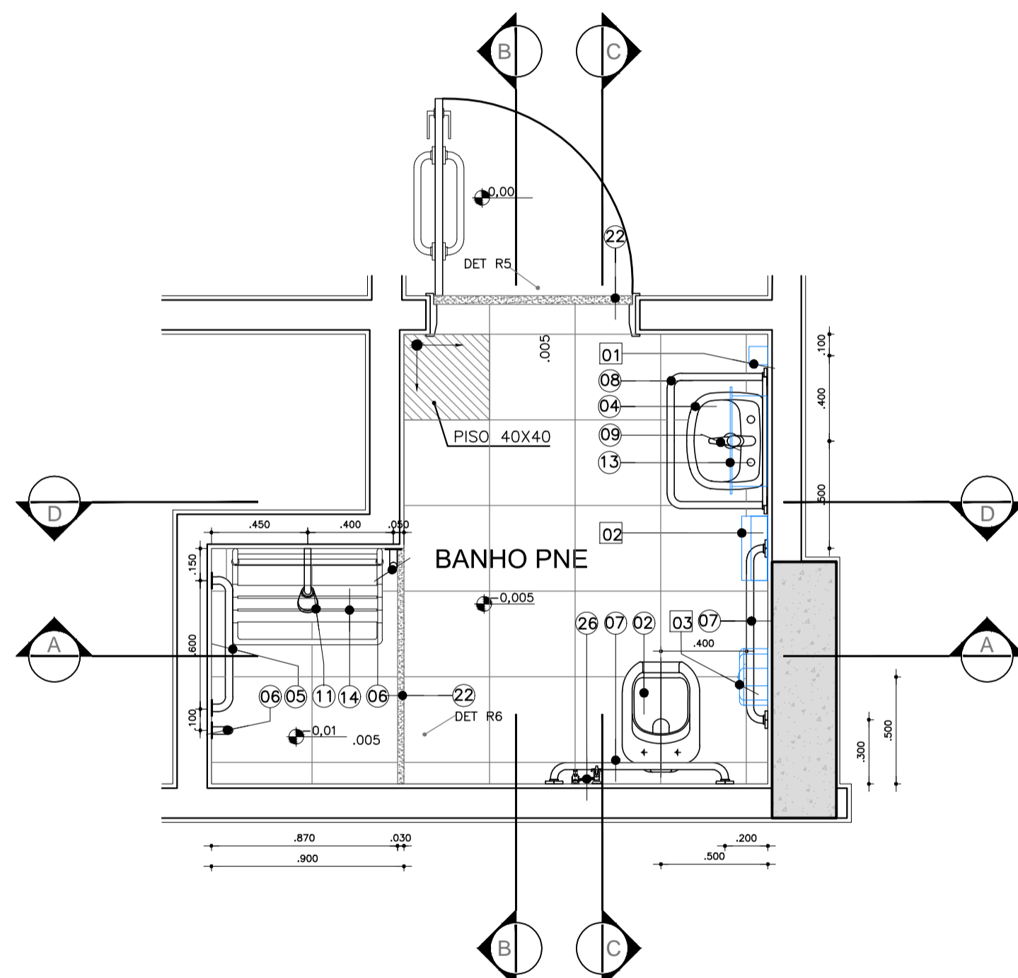
AM-26- SANITÁRIO PNE ISOLAMENTO QUANTIDADE : ESC.: 1:25
