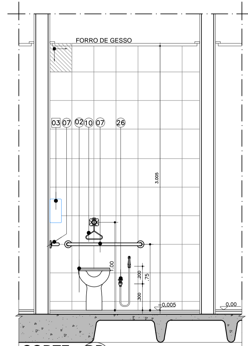
CORTE DD ESCALA 1:25
