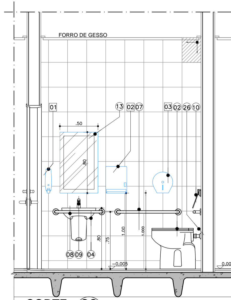
CORTE CC ESCALA 1:25
