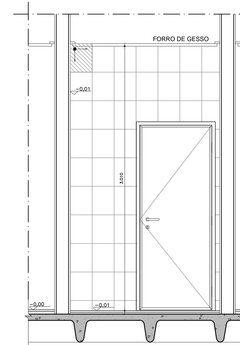
CORTE CC ESCALA 1:25
