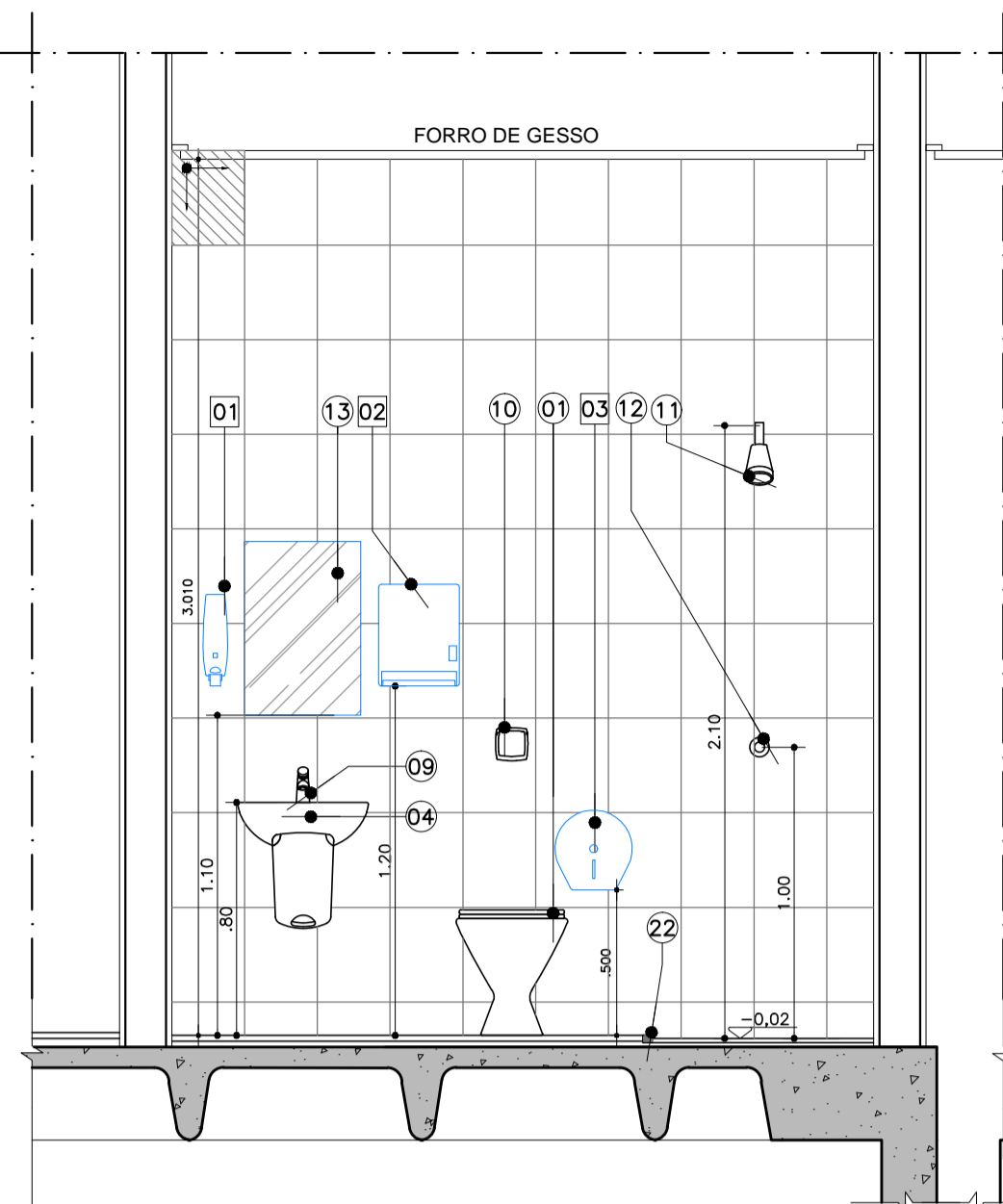
CORTE BB ESCALA 1:25
