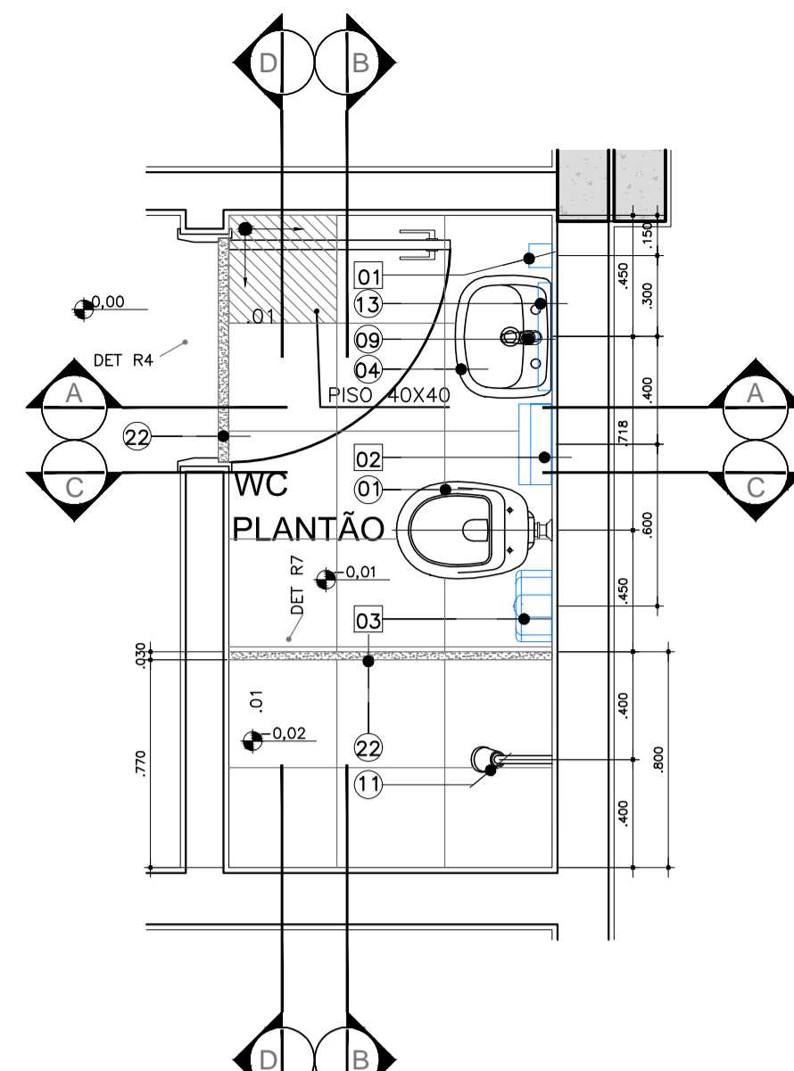
AM-15- W.C PLANTÃO - 1º PAV. QUANTIDADE : ESC.: 1:25
