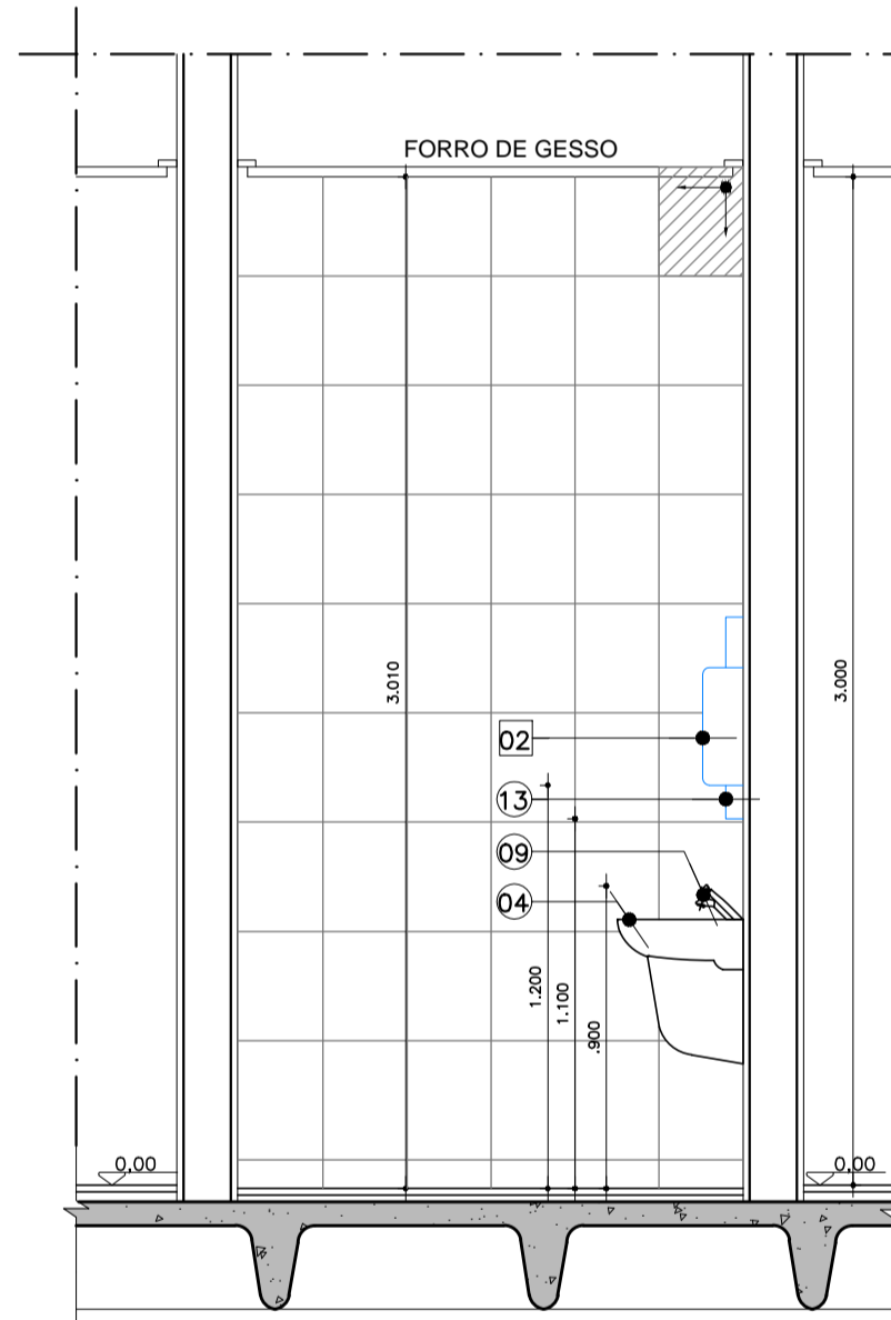
CORTE BB ESCALA 1:25
