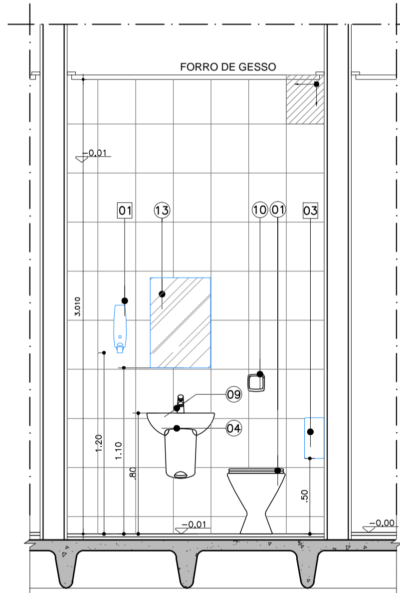
CORTE AA ESCALA 1:25
