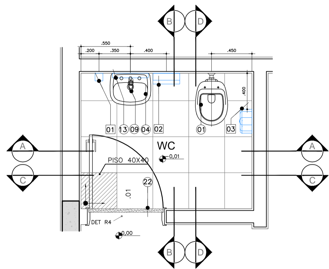
AM-16- W.C - 1º PAV QUANTIDADE : 01 ESC.: 1:25
