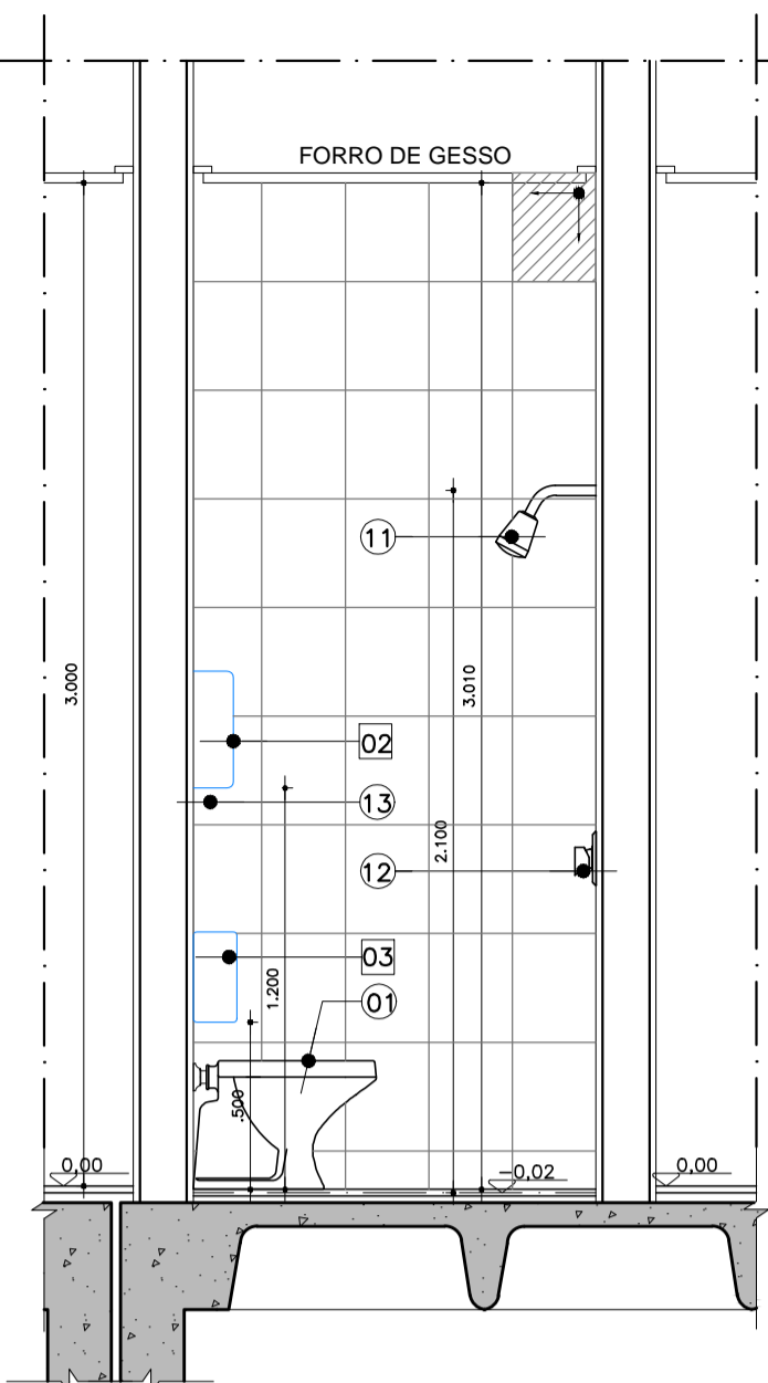
CORTE CC ESCALA 1:25
