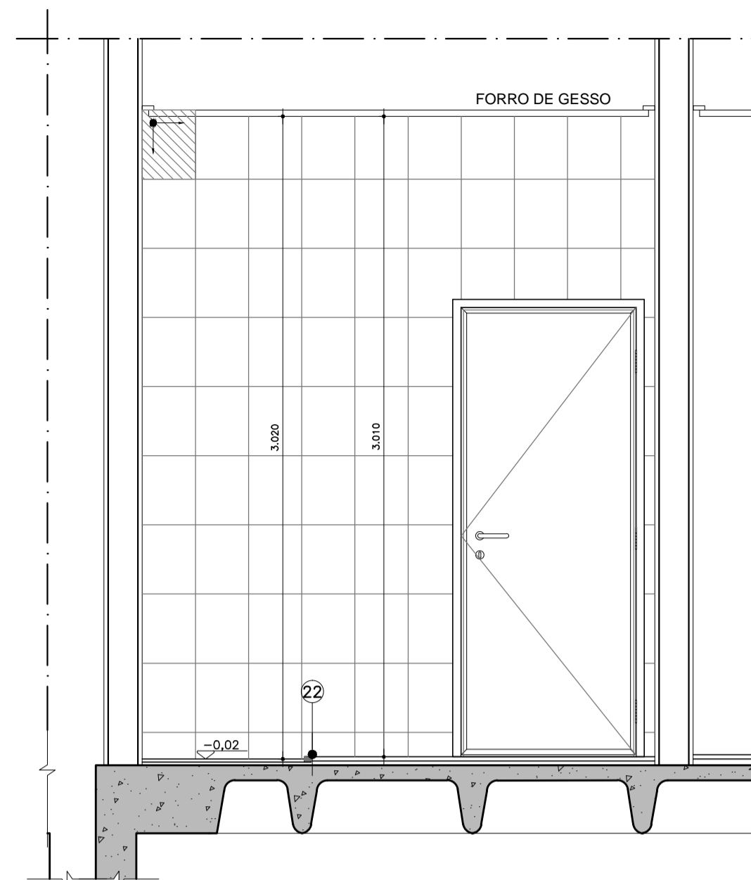
CORTE DD ESCALA 1:25
