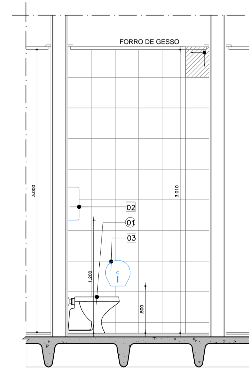
CORTE DD ESCALA 1:25
