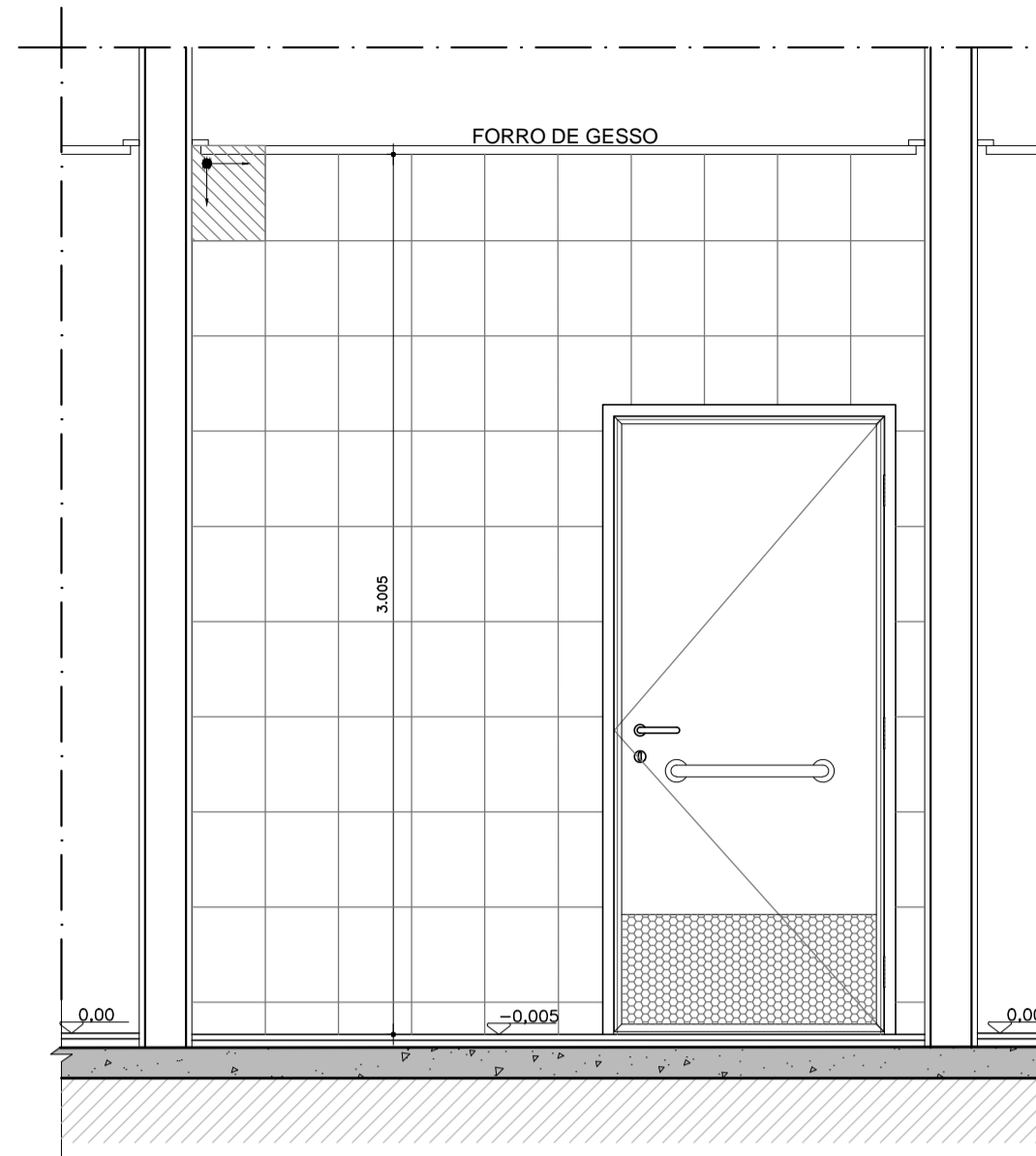
CORTE DD ESCALA 1:25 AM-03- SANITÁRIO PNE - TÉRREO
