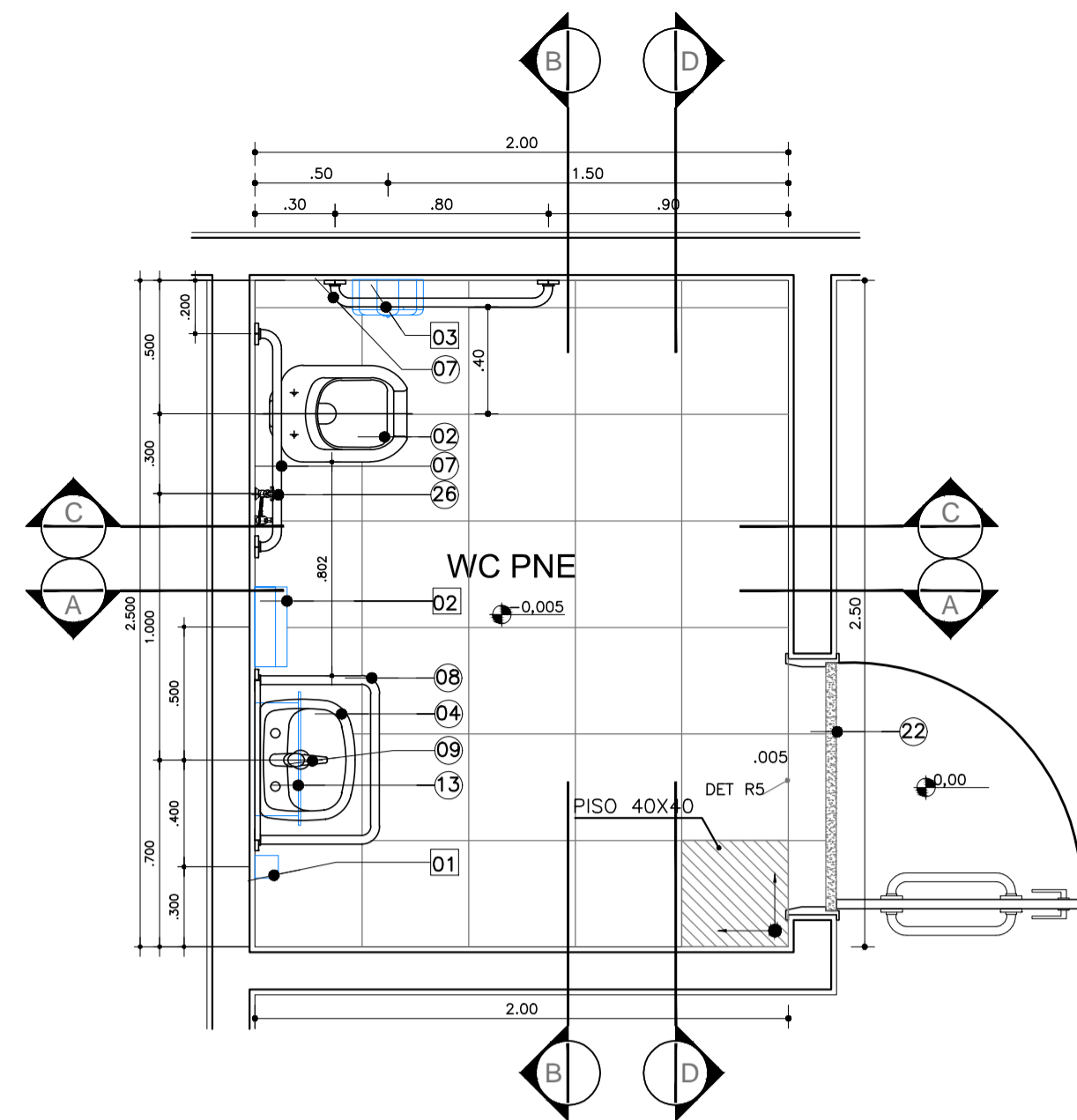
AM-03- SANITÁRIO PNE PREPARAÇÃO DE PACIENTES - TÉRREO QUANTIDADE: 1 ESC.: 1:25
