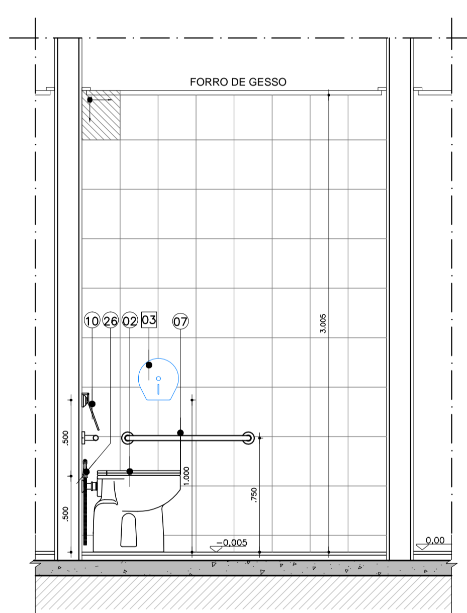
CORTE AA ESCALA 1:25 AM-04 SANITÁRIOS PNE - TÉRREO
