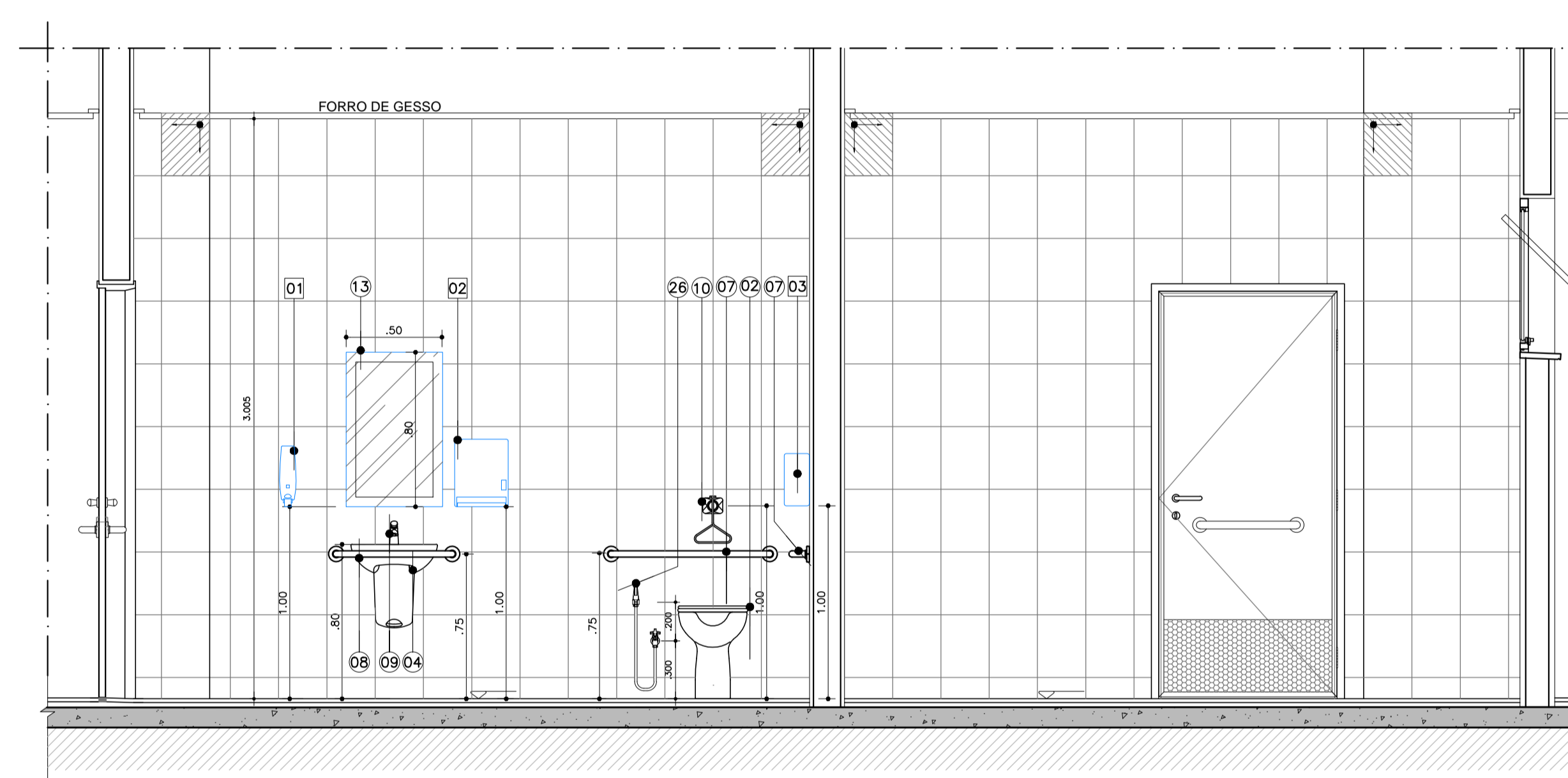
CORTE BB ESCALA 1:25 AM-04 SANITÁRIOS PNE - TÉRREO
