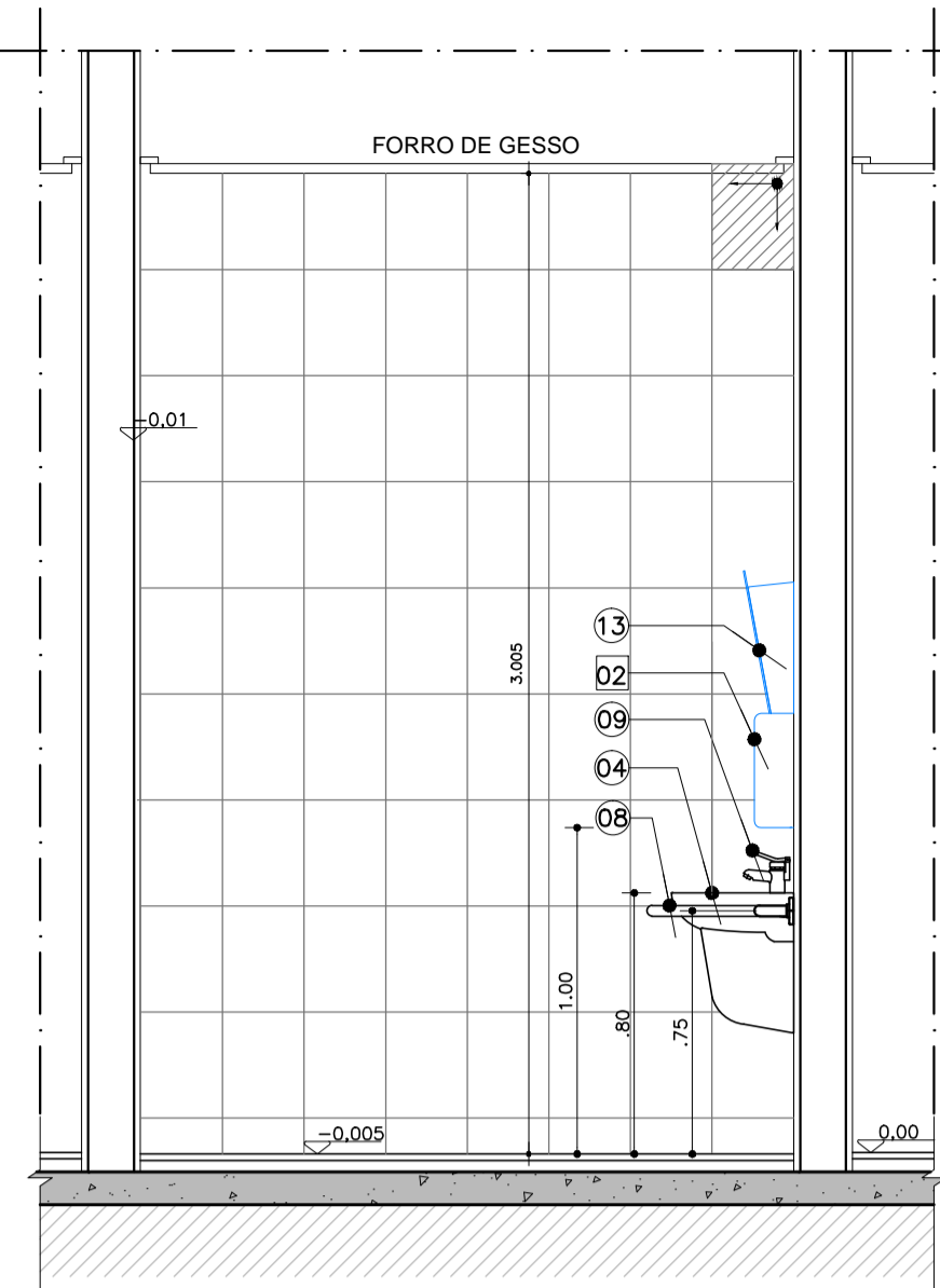
CORTE AA ESCALA 1:25 AM-03- SANITÁRIO PNE - TÉRREO
