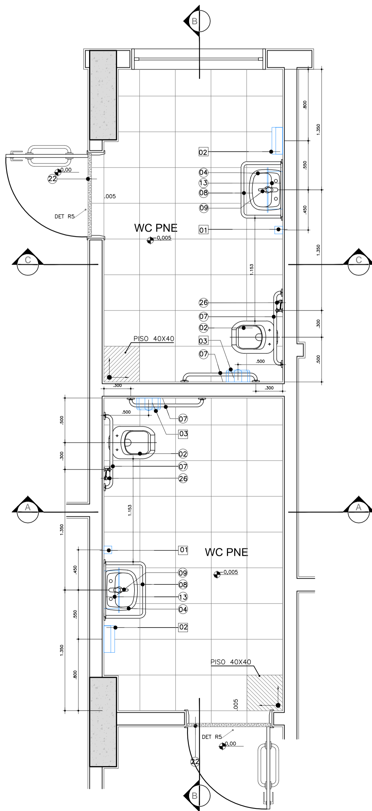
AM-04 SANITÁRIOS PNE - TÉRREO QUANTIDADE: 1 ESC.: 1:25
