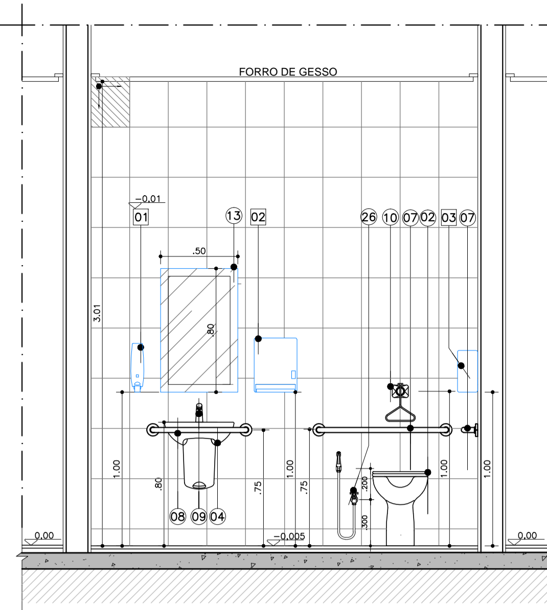
CORTE BB ESCALA 1:25 AM-03- SANITÁRIO PNE - TÉRREO
