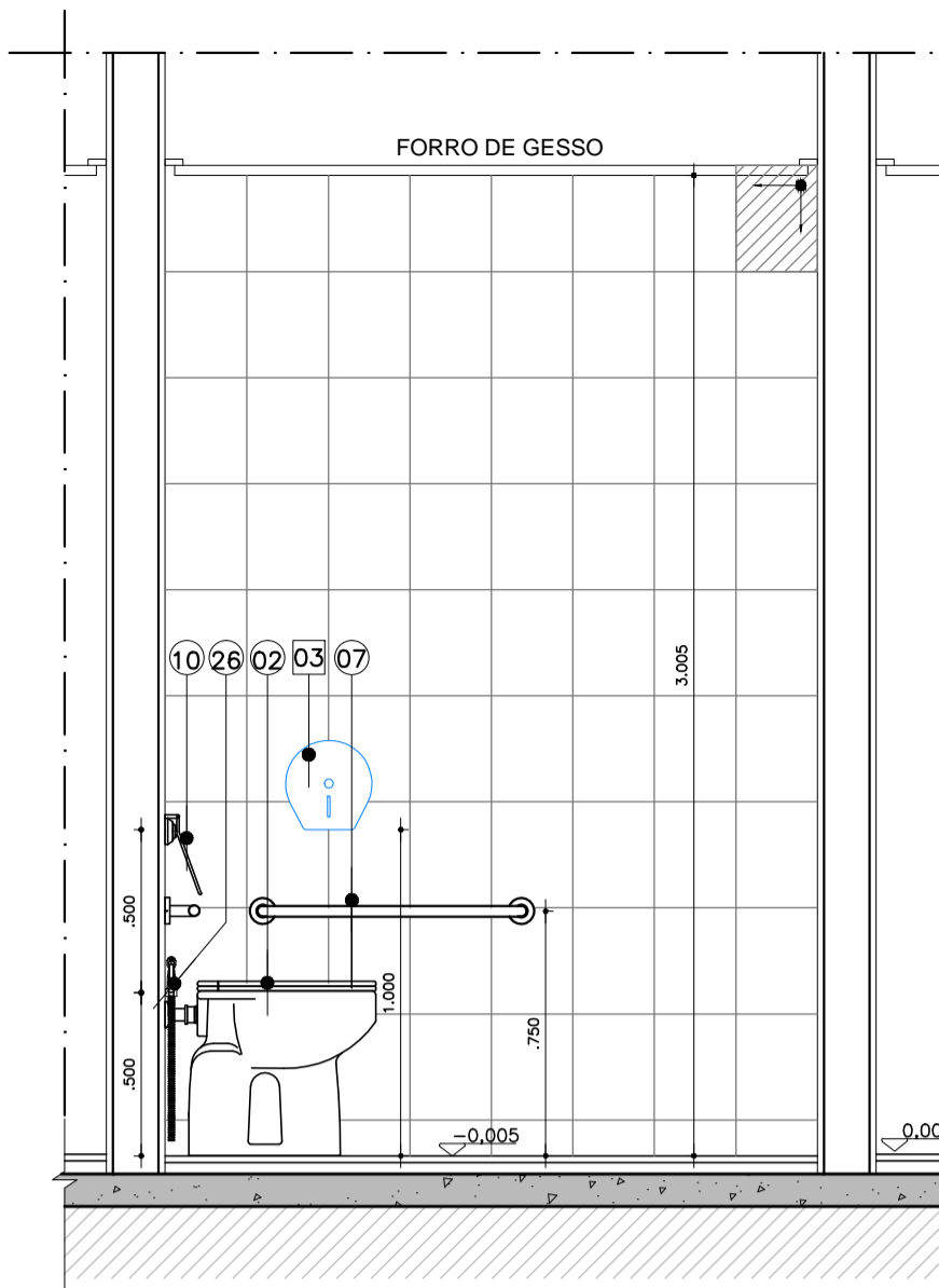
CORTE BB ESCALA 1:25 AM-01- WC PLANTÃO - TÉRREO
