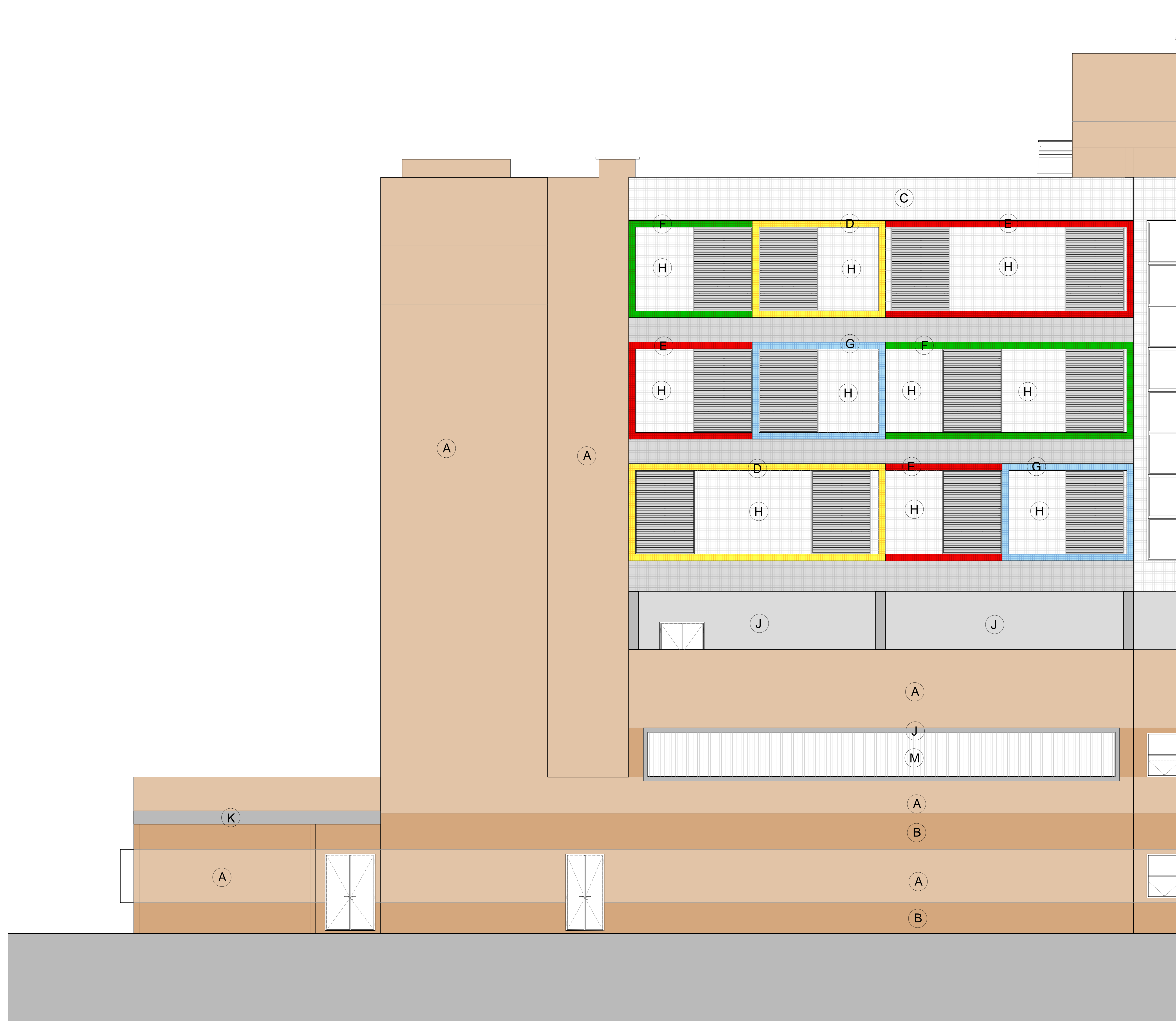
BLOCO 1 - ELEVÇÃO 02 ESC 1:50
