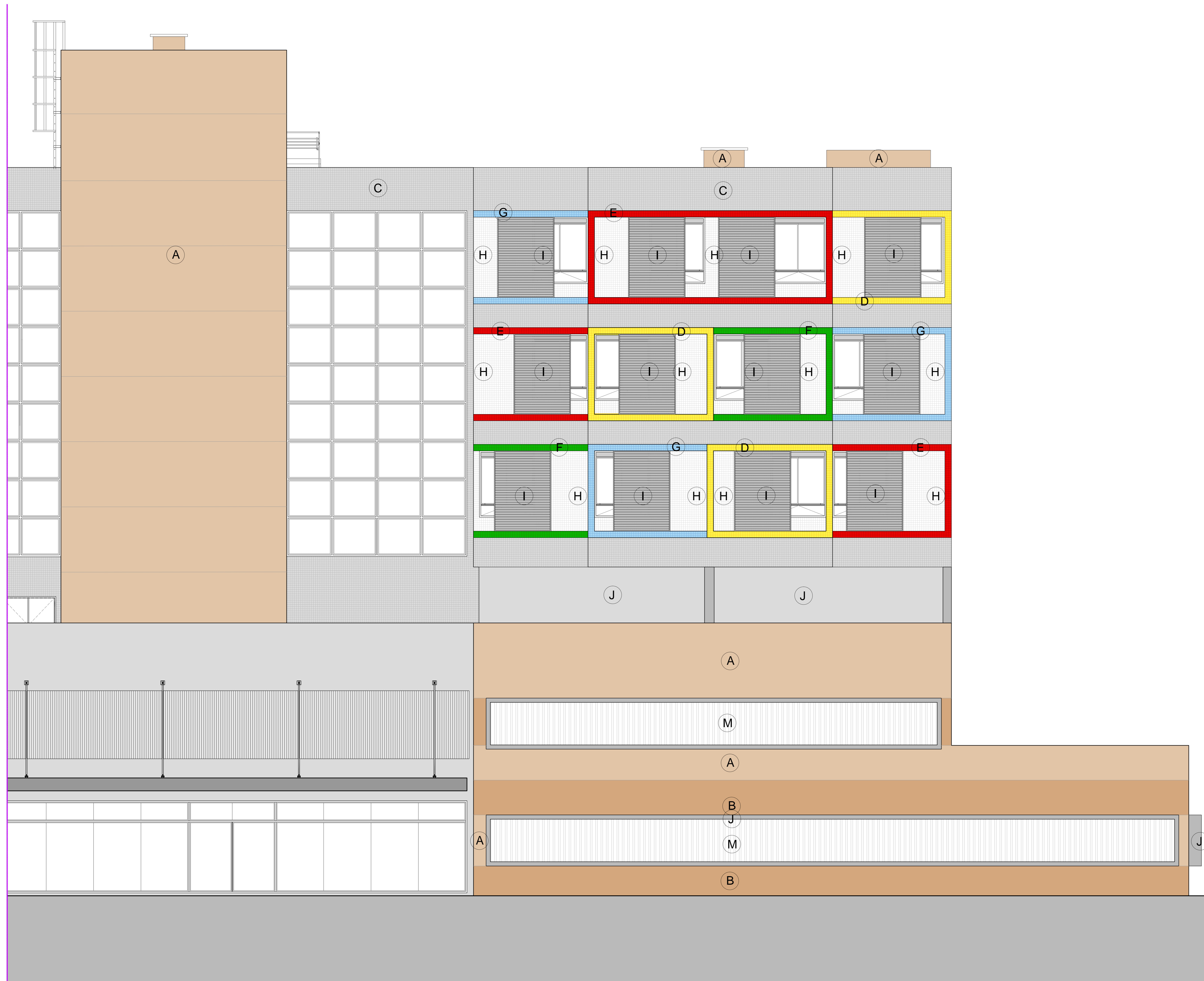
1B BLOCO 1 - ELEVAÇÃO 01 ESC 1:50
