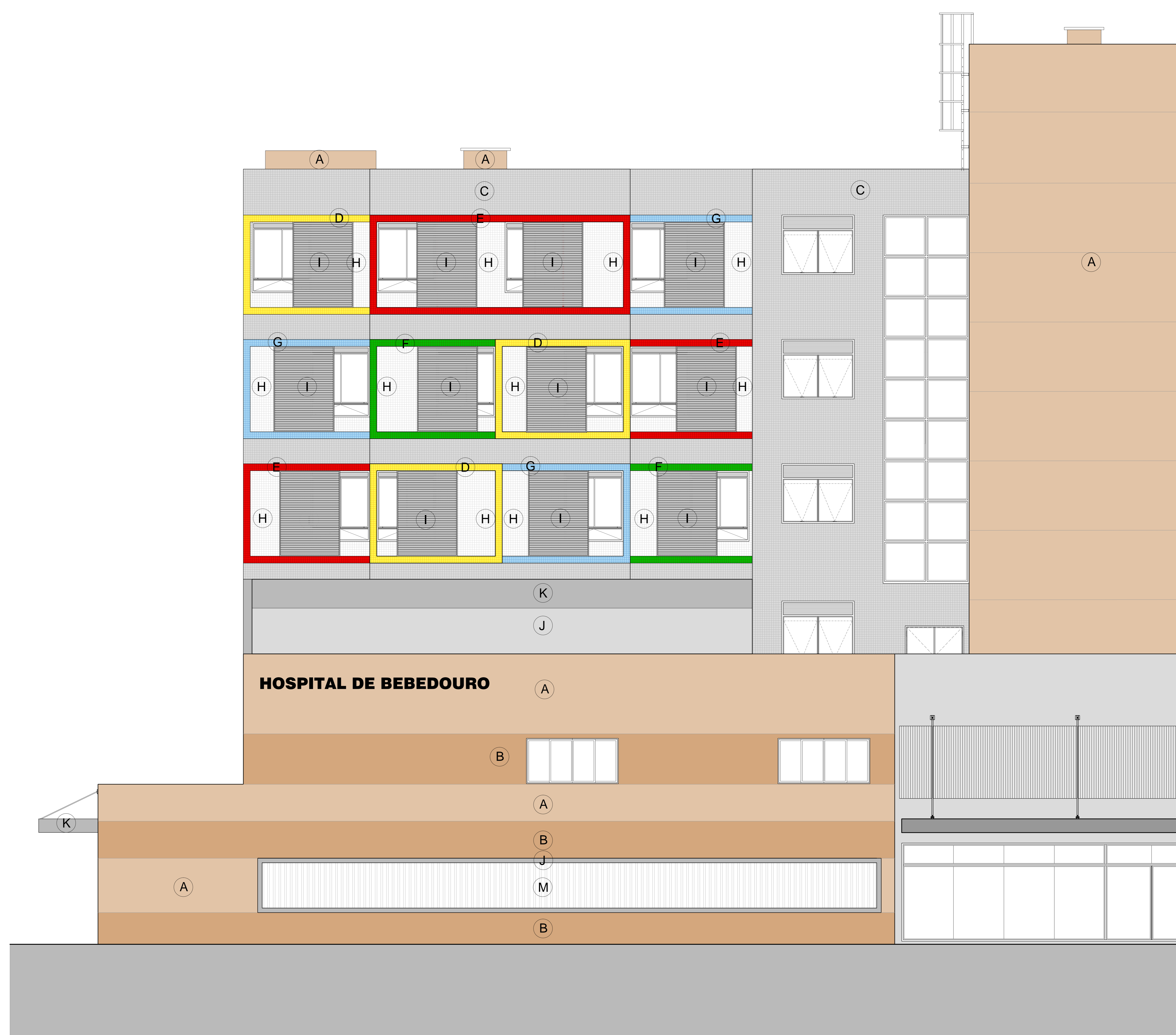
BLOCO 1 - ELEVÇÃO 01 ESC 1:50
