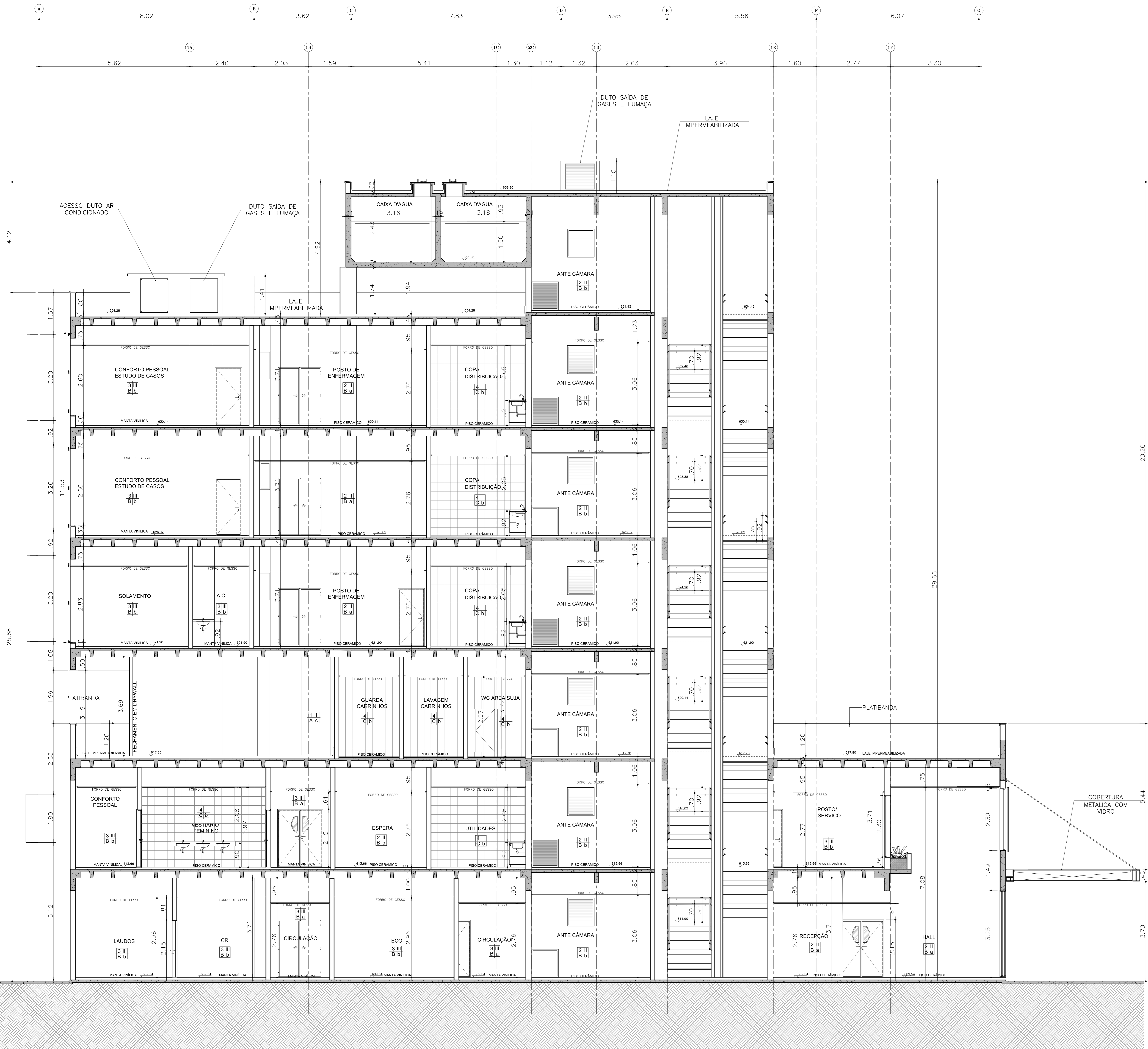
BLOCO 1 - CORTE BB ESC 1:50
