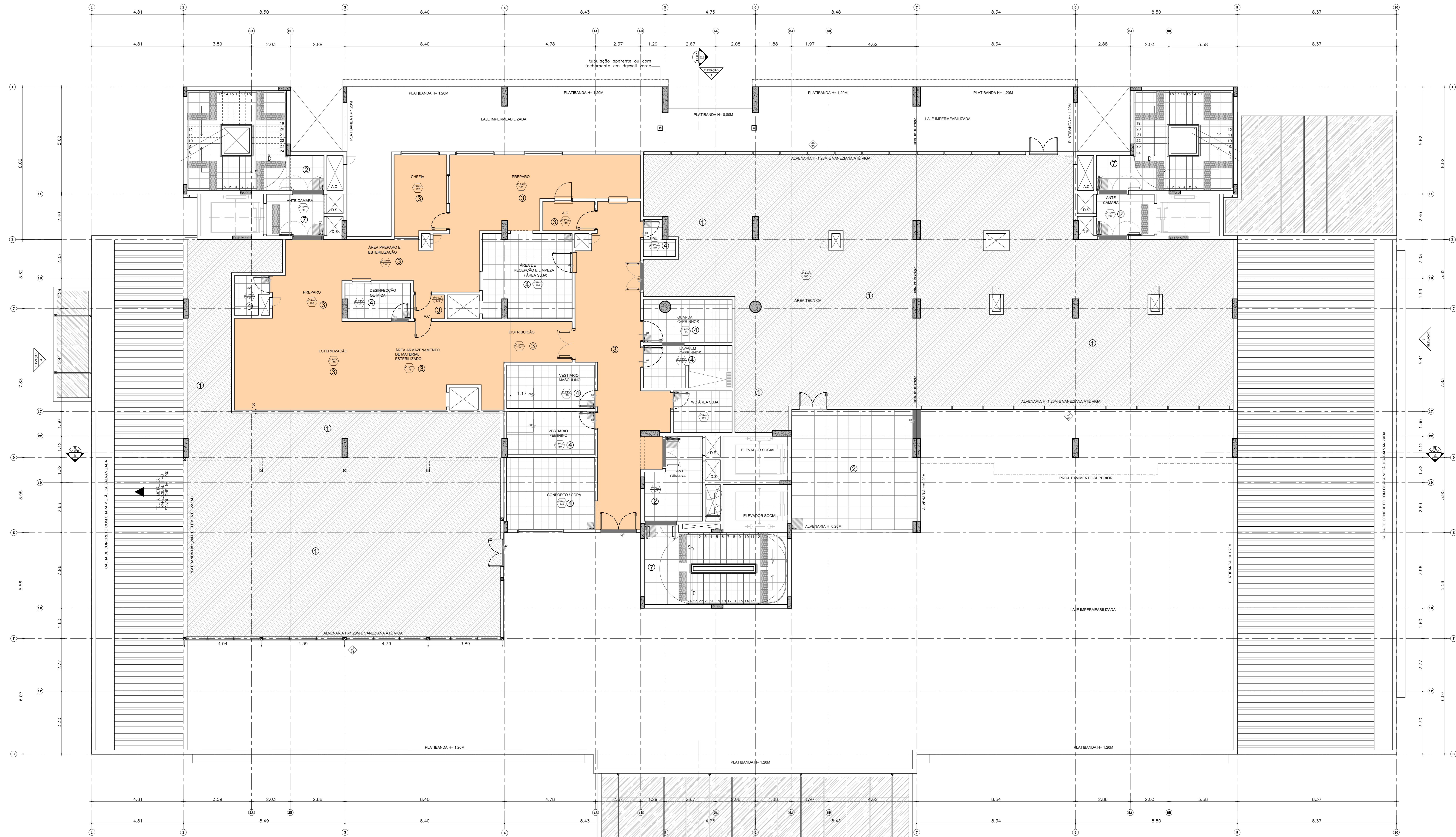
PLANTA PISO BLOCO 1- 2º PAVIMENTO ESC 1:50
