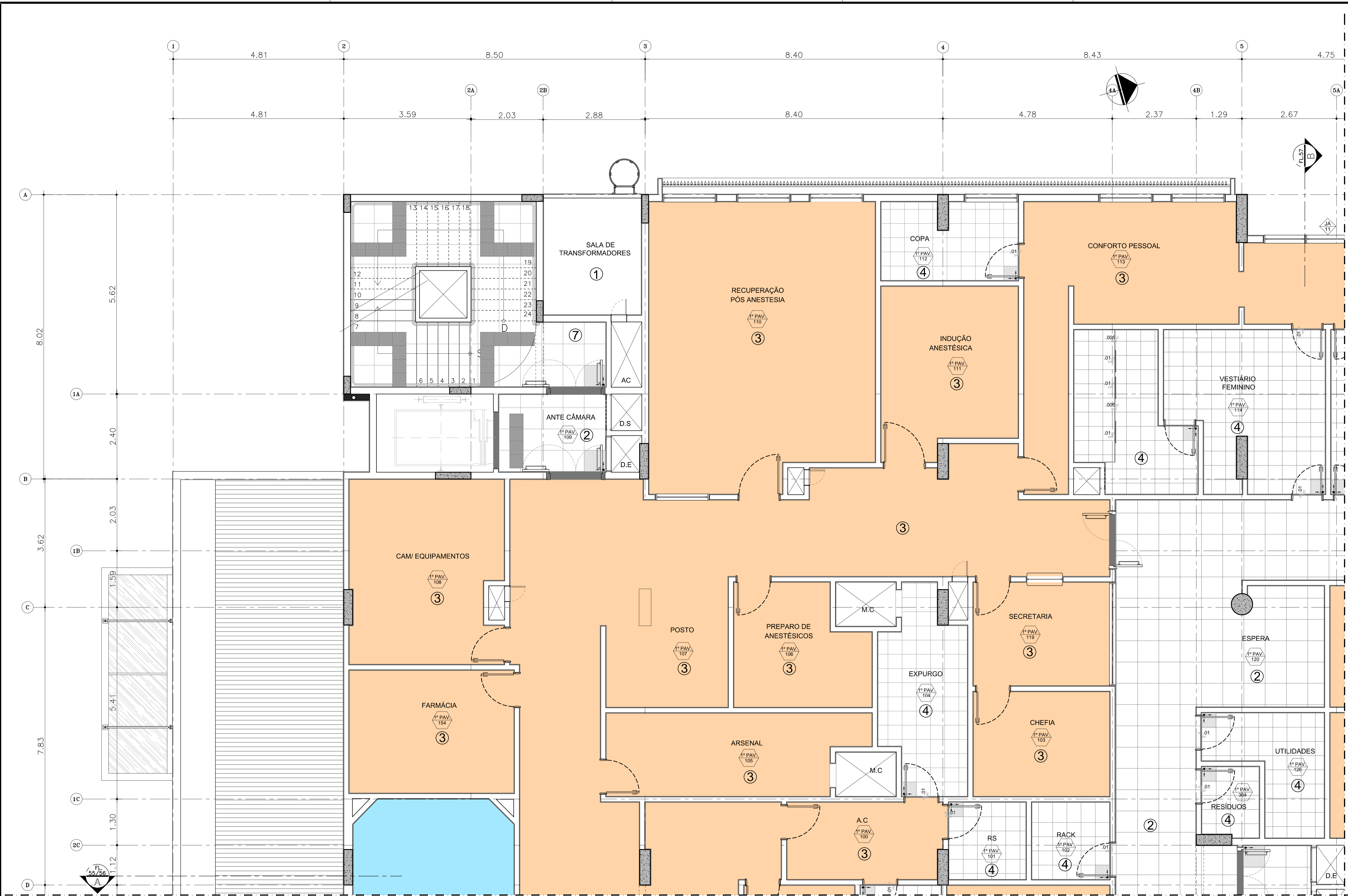
PLANTA PISO BLOCO 1 - 1º PAVIMENTO ESC 1:50
