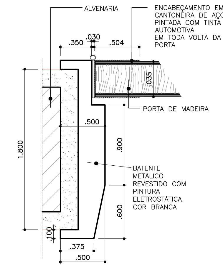
DETALHE 01 ESCALA 1:2
