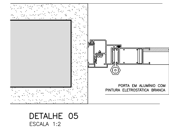
DETALHE BATENTE METÁLICO - PINTURA ELETROSTÁTICA COR BRANCA
