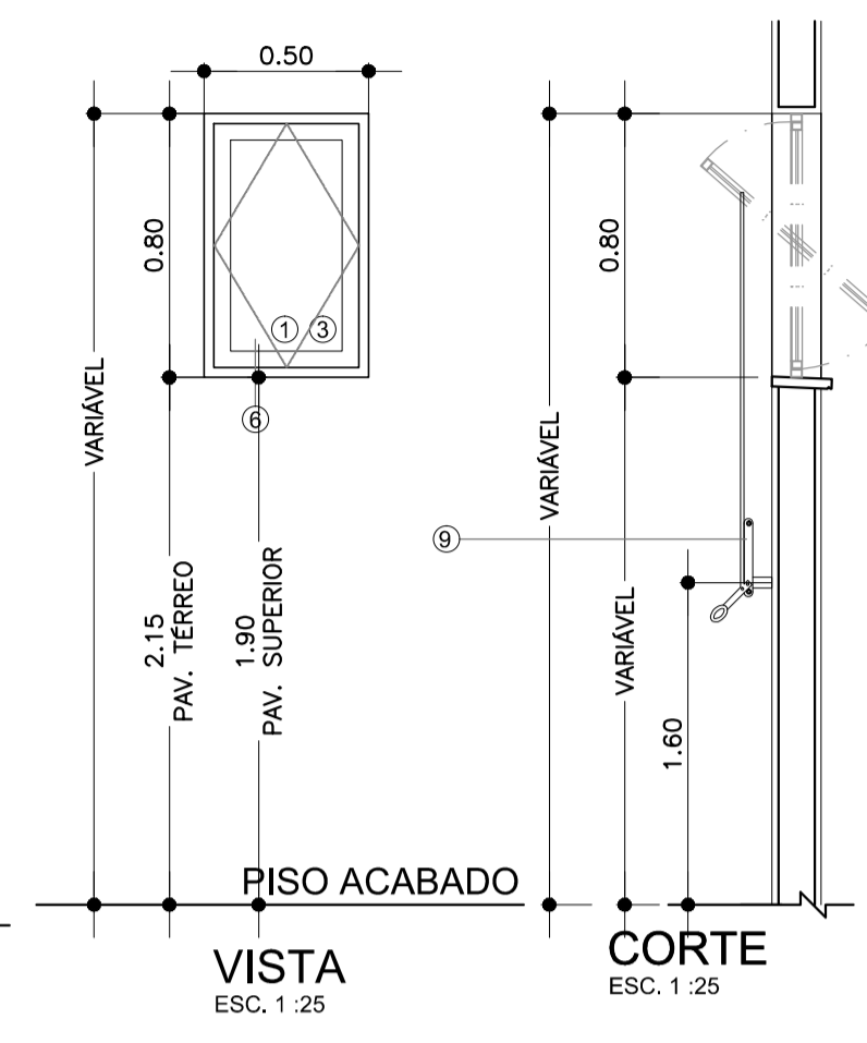
CORTE ESC. 1:25
