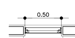
PLANTA ESC. 1:25
