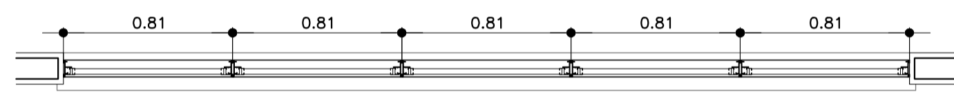
PLANTA ESC. 1:25
