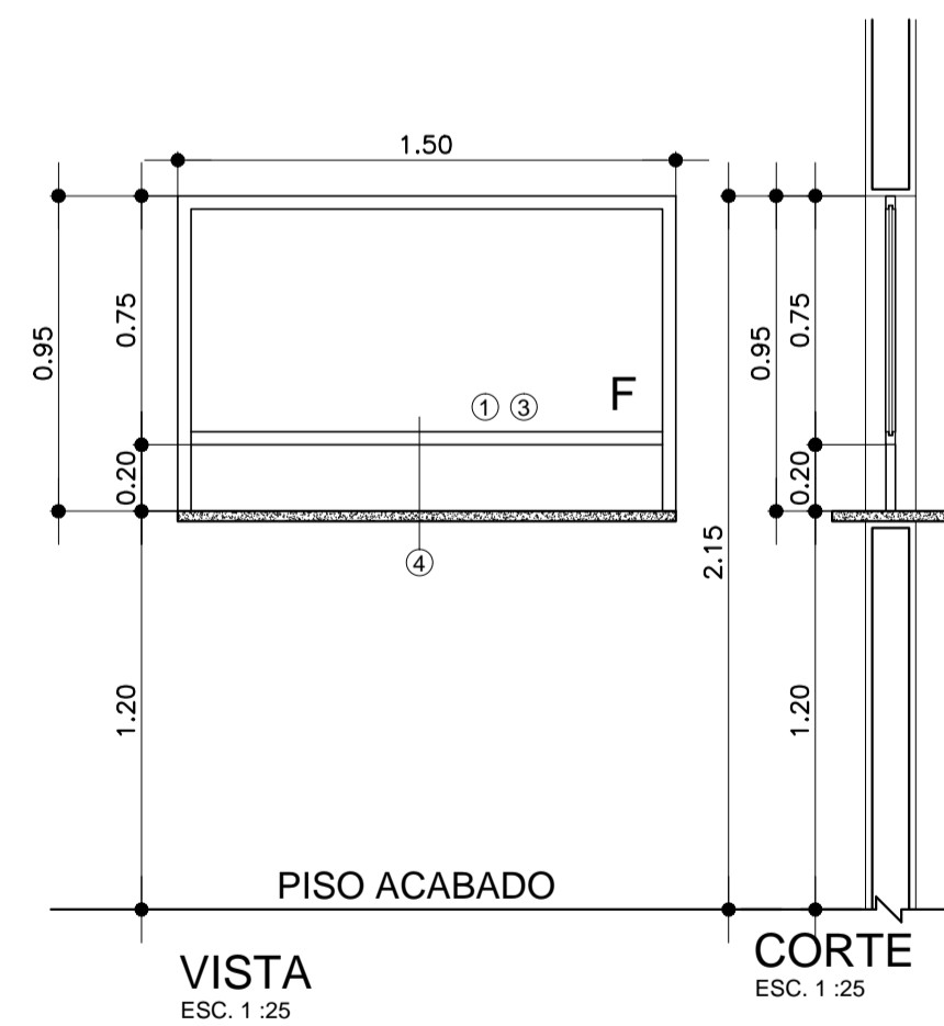
VISTA ESC. 1:25
