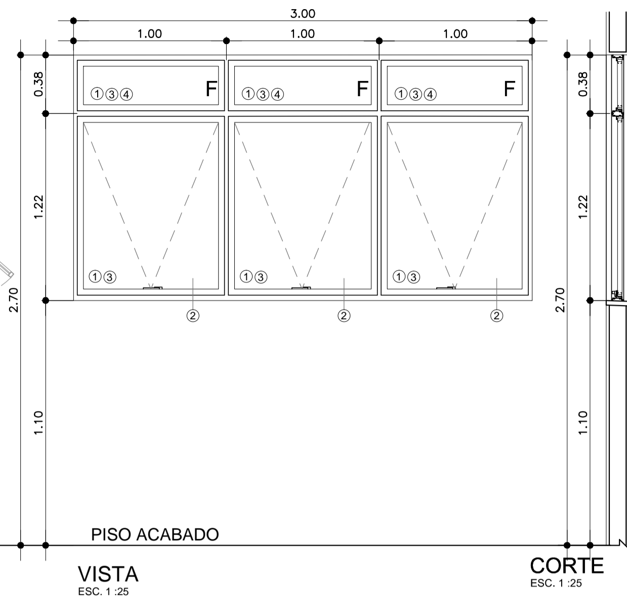
JA 20 ESQUADRIA ALUMÍNIO COM VIDRO TIPO MAXIM-AR E VIDRO FIXO QUANTIDADE: 3 UNIDADES
