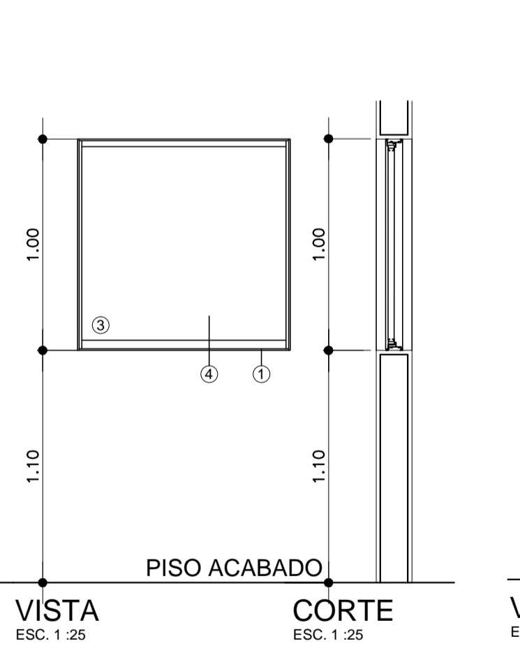
VISTA ESC. 1:25
