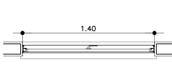
PLANTA ESC. 1:25
