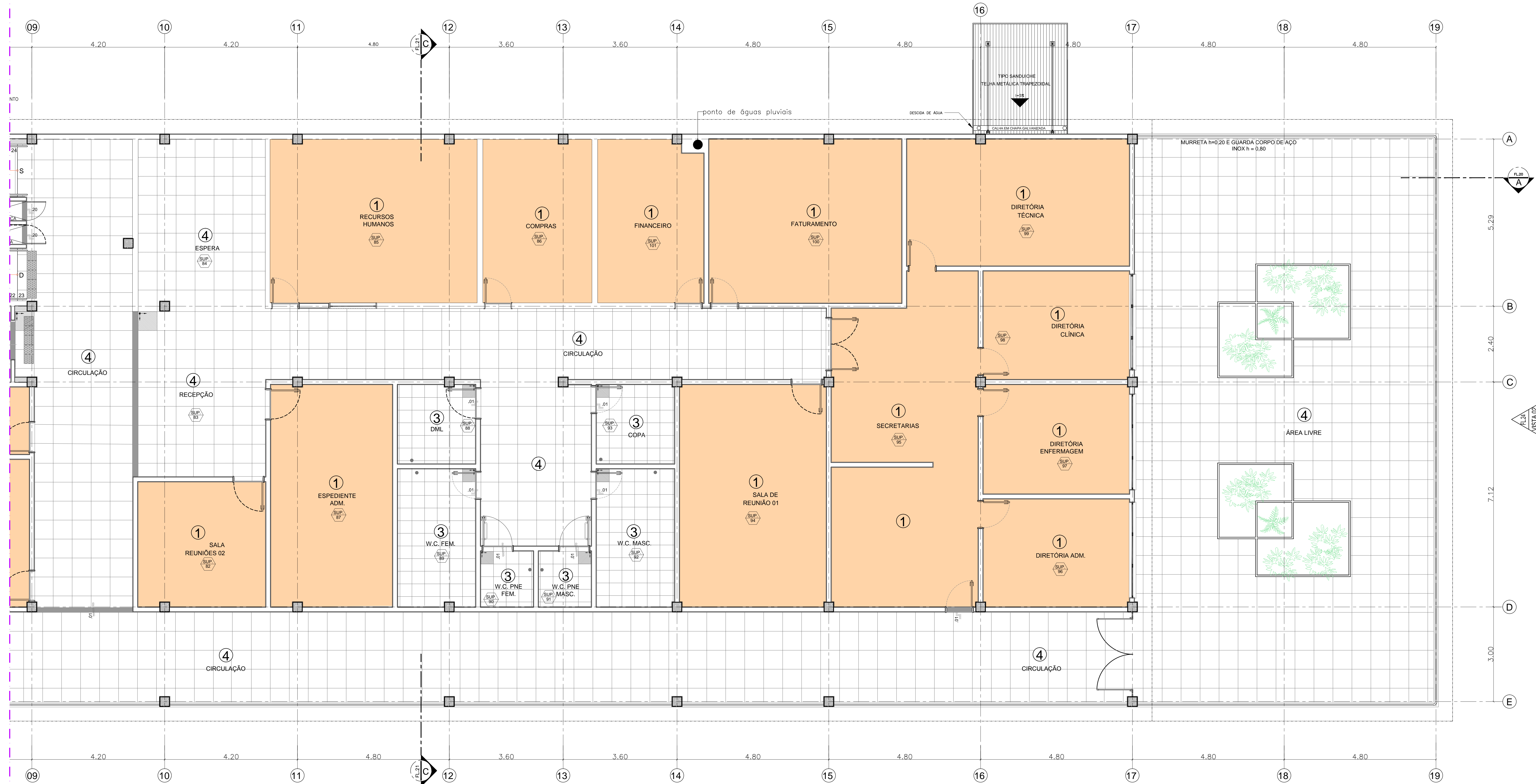
BLOCO 2 - PLANTA PISO PAVIMENTO SUPERIOR ESC 1:50
