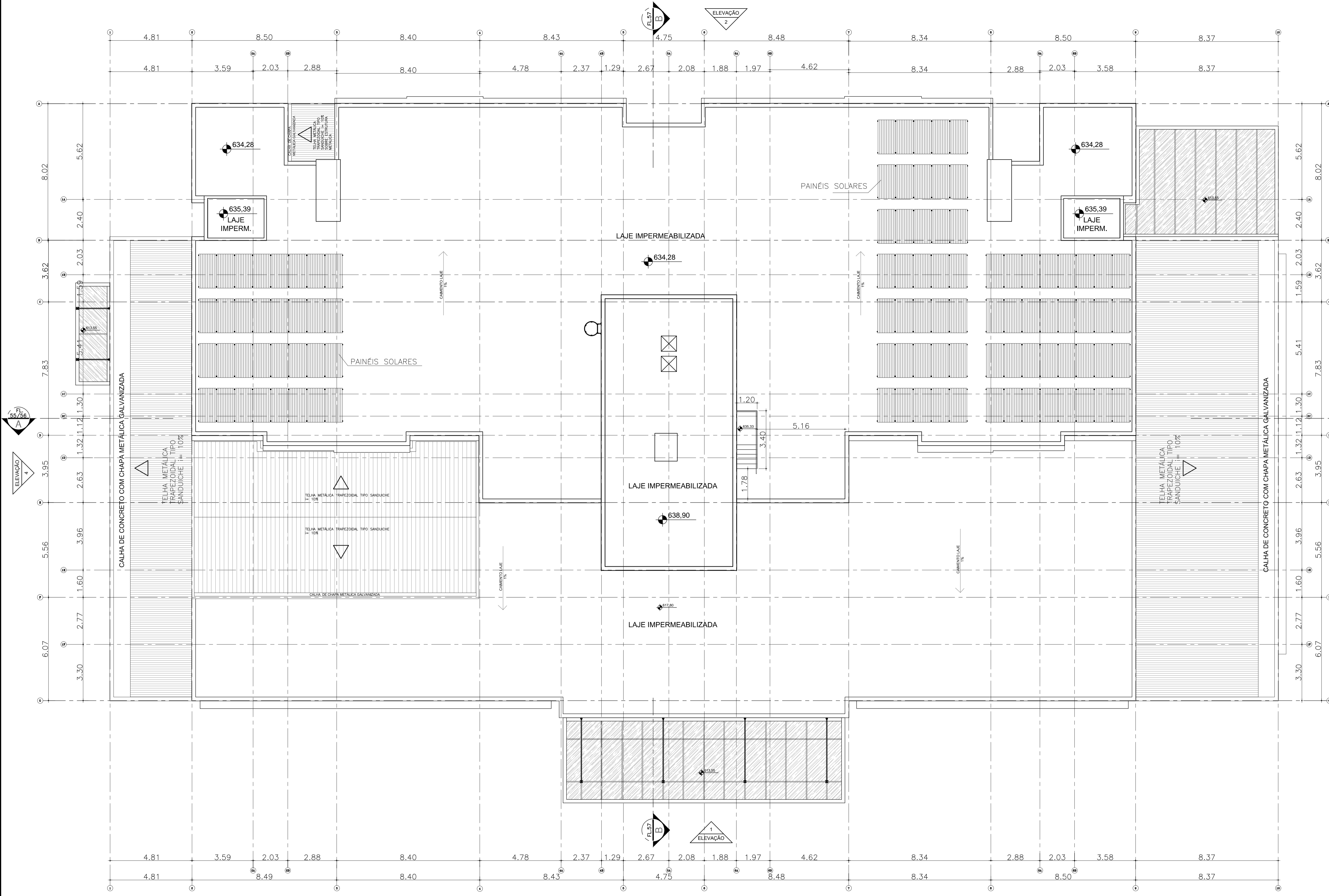
PLANTA BLOCO 1 - COBERTURA ESC 1:100
