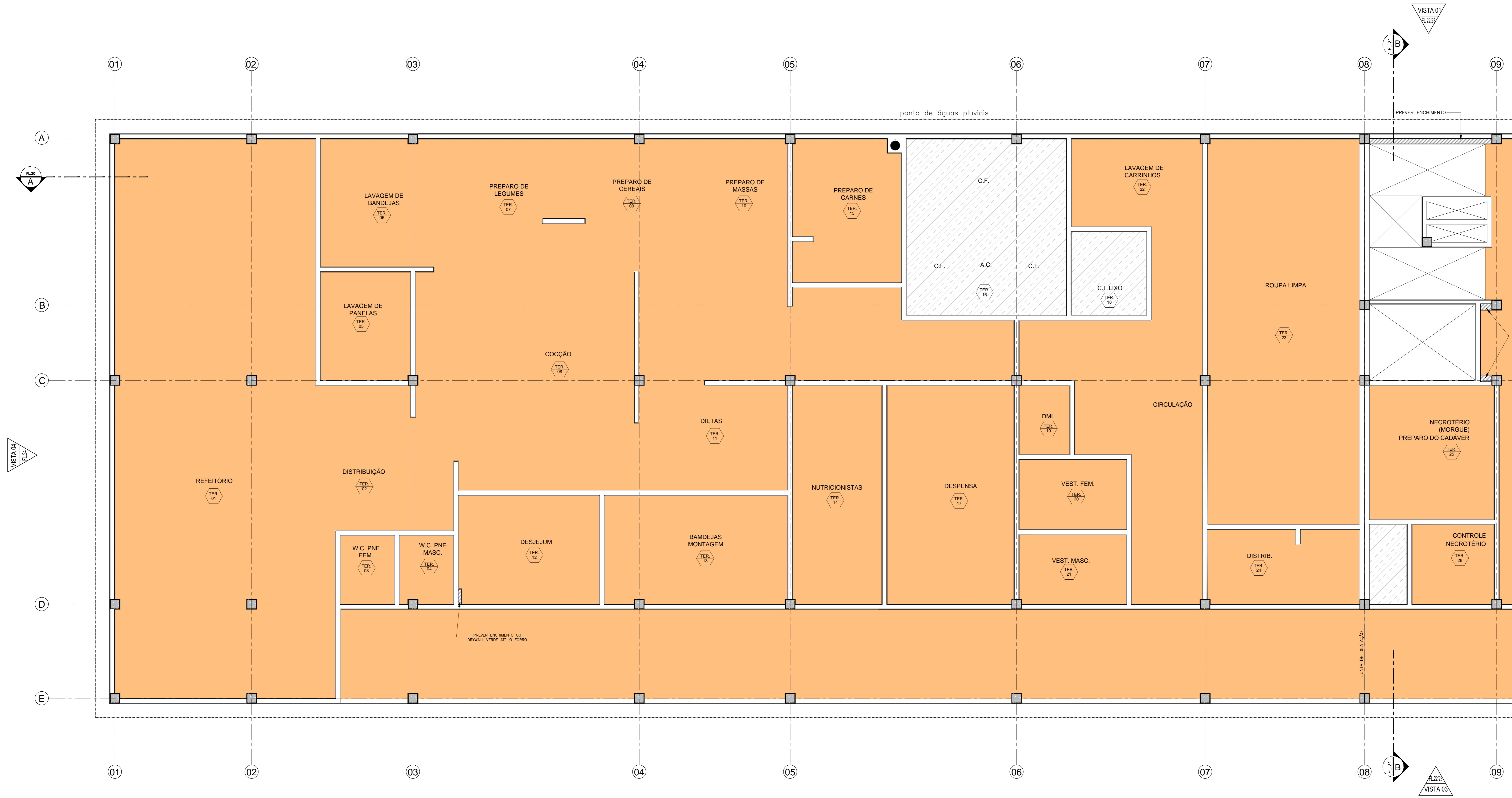
BLOCO 2 - PLANTA FORRO PAVIMENTO TÉRREO ESC 1:50
