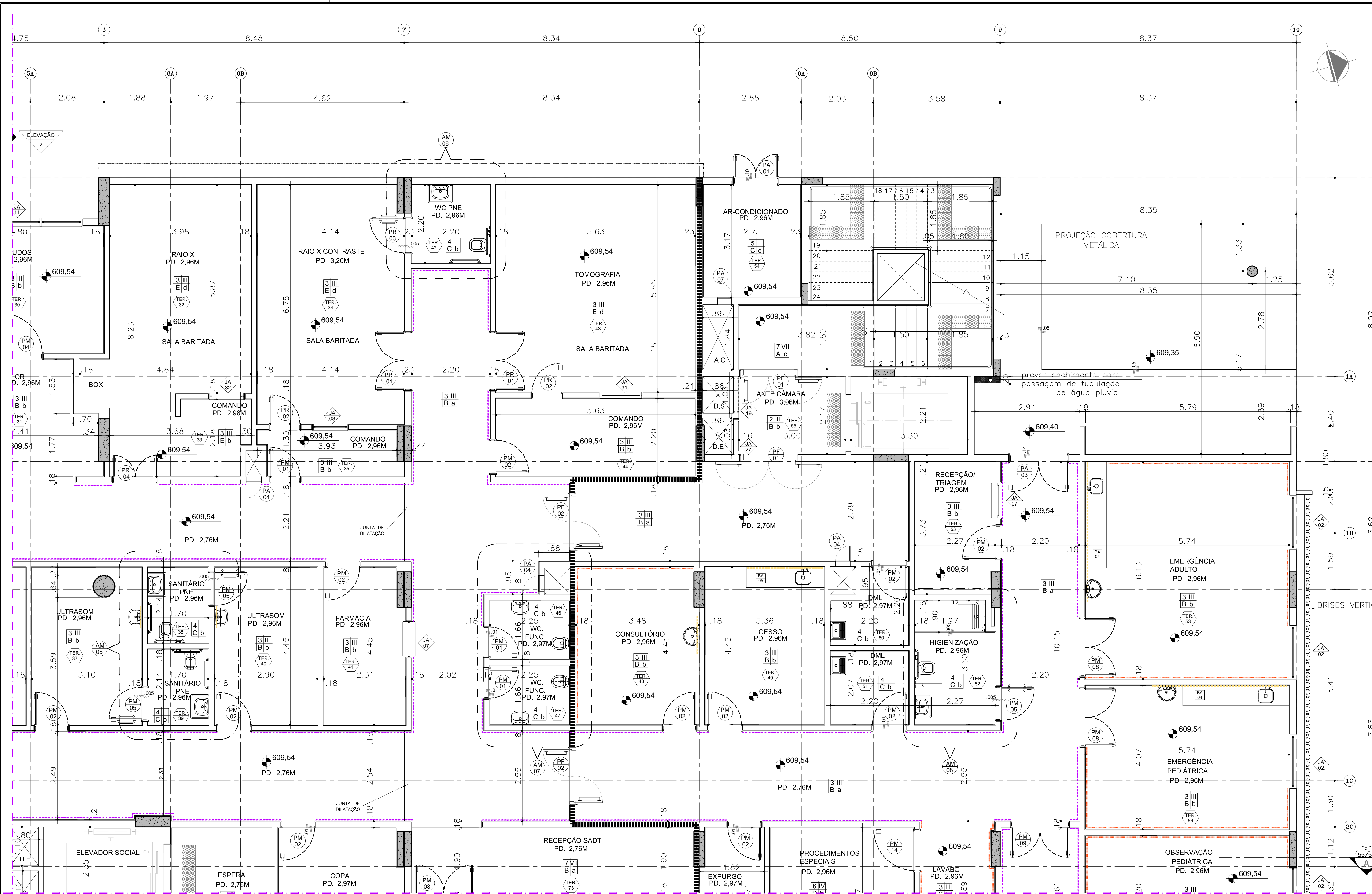
1A PLANTA ALVENARIA BLOCO 1 - TÉRREO ESC 1:50
